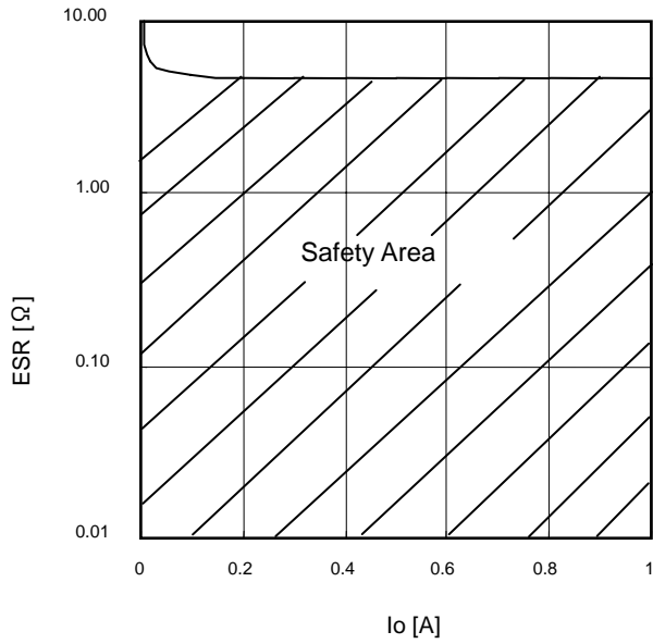
Figure 31. ESR 安全動作範囲
