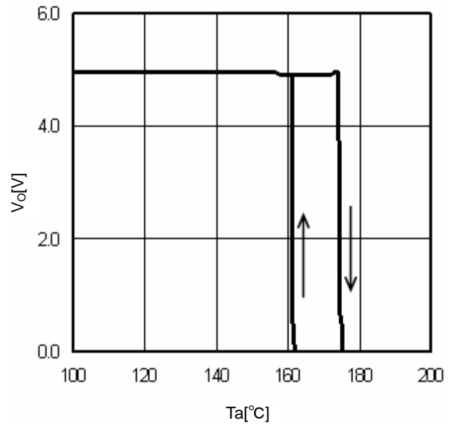
Fig.15 TSD (I O =0mA)
