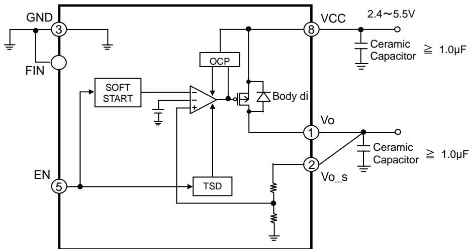
Figure 2. ブロック図 (固定出力タイプ)
