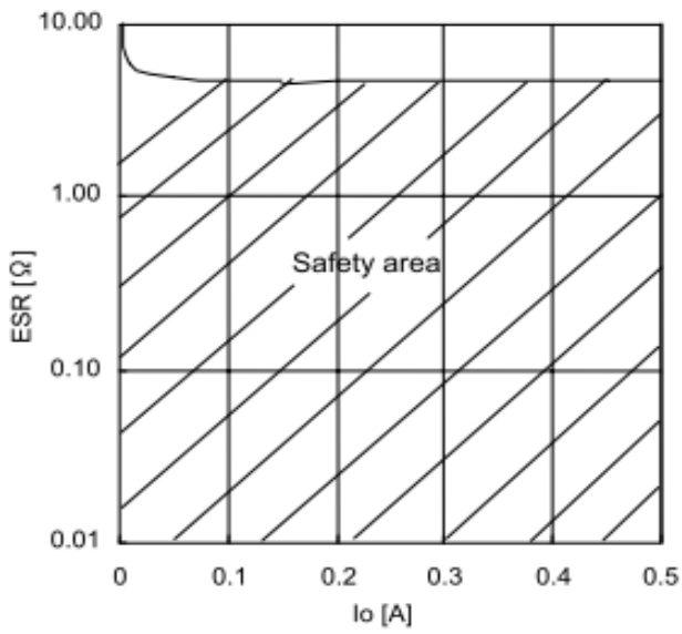
Figure 31. ESR 安全動作範囲
