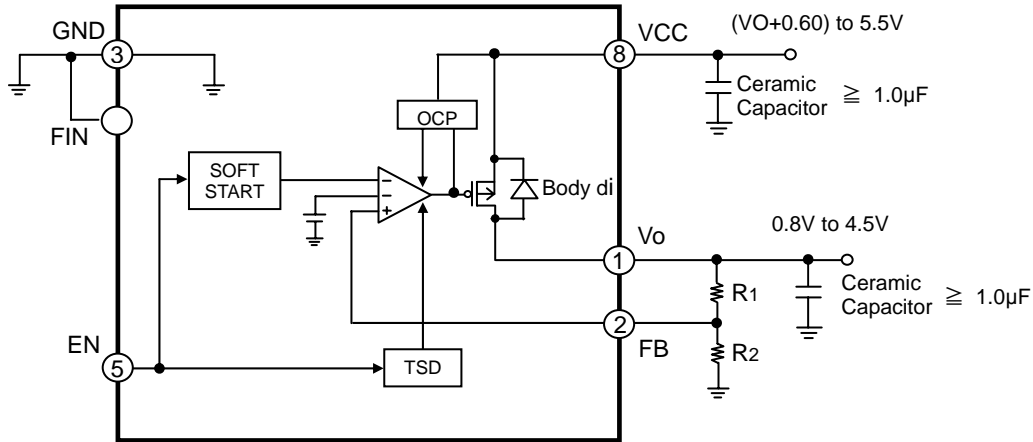
Figure 1. ブロック図 (可変出力タイプ)
