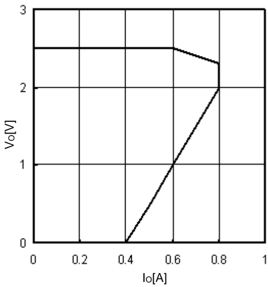
Fig.17 OCP
