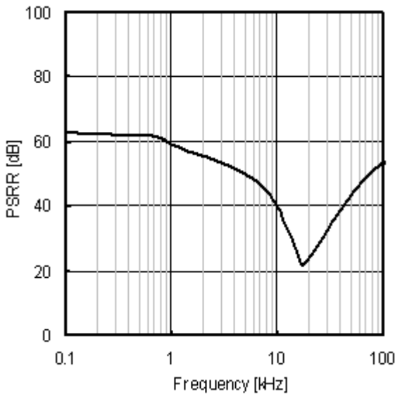
Fig.21 PSRR( I_o=0mA )
