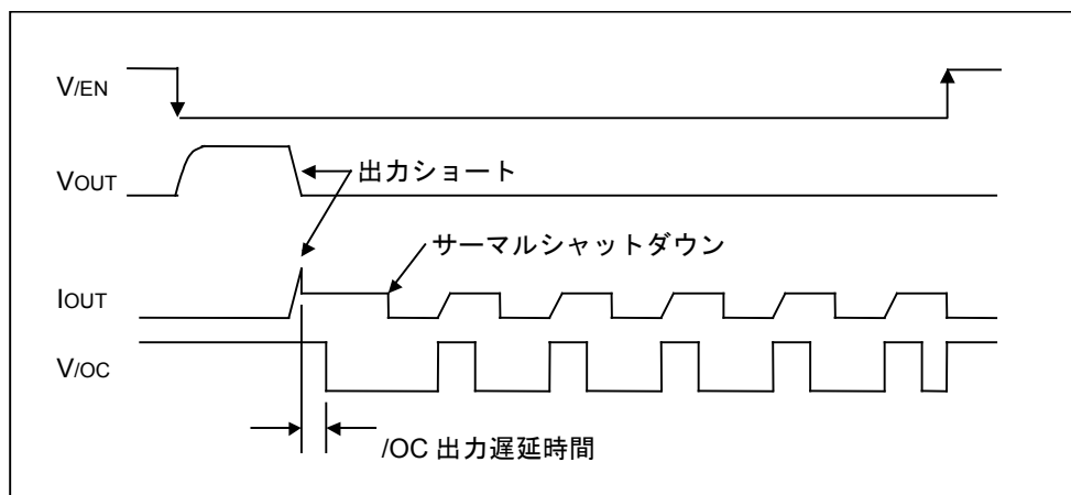
Figure 38. 過電流検出、サーマルシャットダウンタイミング (BD2041AFJ)
