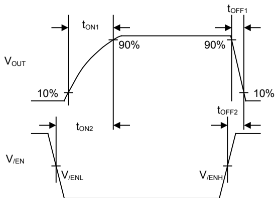
Figure 22. タイミングダイアグラム (BD2041AFJ)
