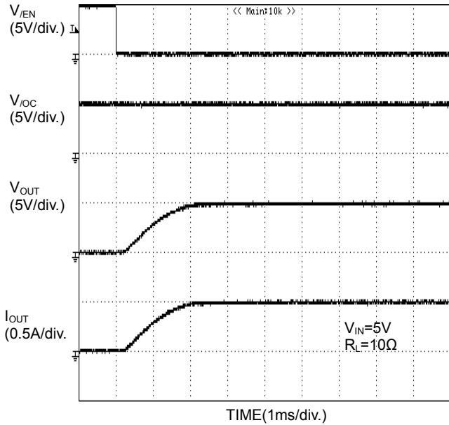
Figure 28. 出力立ち上り特性 (BD2041AFJ)
