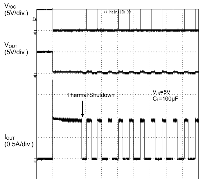
TIME (500ms/div.) Figure 35. 過電流検出特性 Enable時に出力1Ωショート (BD2041AFJ)
