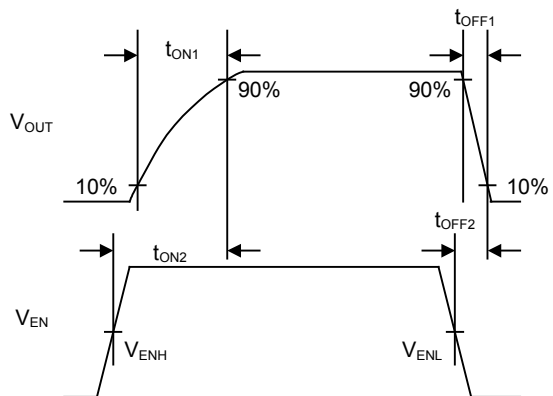
Figure 3. タイミングダイアグラム (BD2051AFJ)
