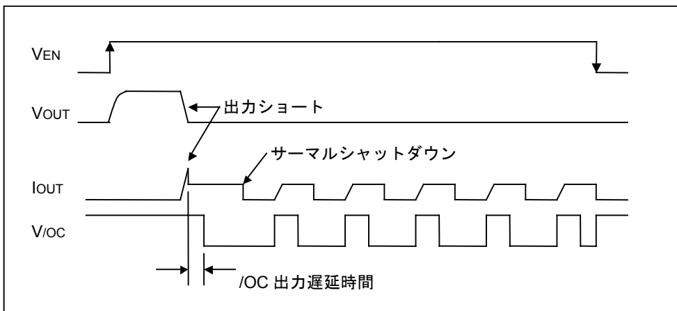
Figure 39. 過電流検出、サーマルシャットダウンタイミング (BD2051AFJ)
