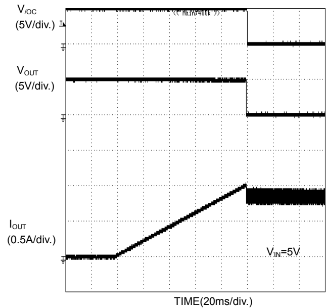
Figure 31. 過電流検出特性 ランプ出力 (BD2041AFJ)
