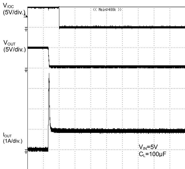
TIME (2ms/div.) Figure 34. 過電流検出特性 Enable時に出力1Ωショート (BD2041AFJ)
