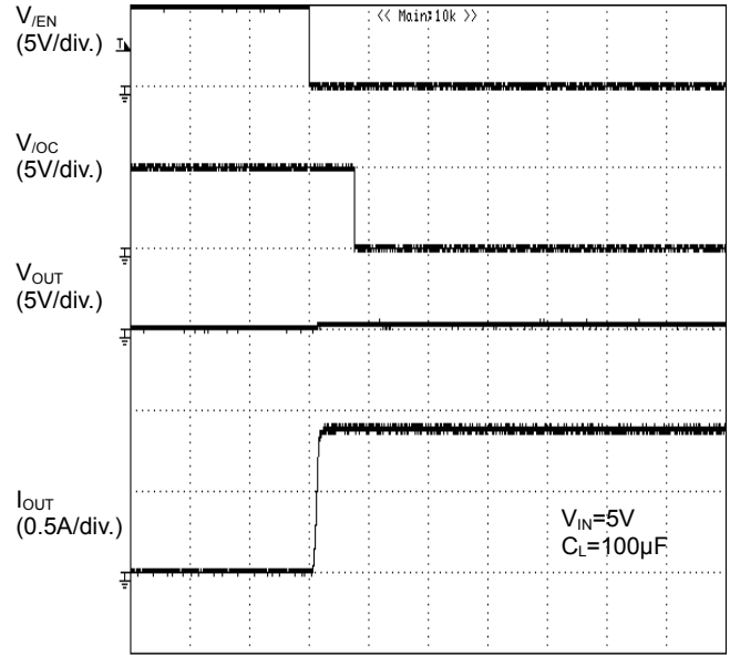
TIME (2ms/div.) Figure 33. 過電流検出特性 ショート状態への Enable (BD2041AFJ)
