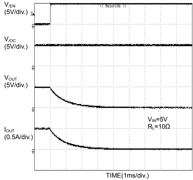
Figure 29. 出力立ち下り特性 (BD2041AFJ)
