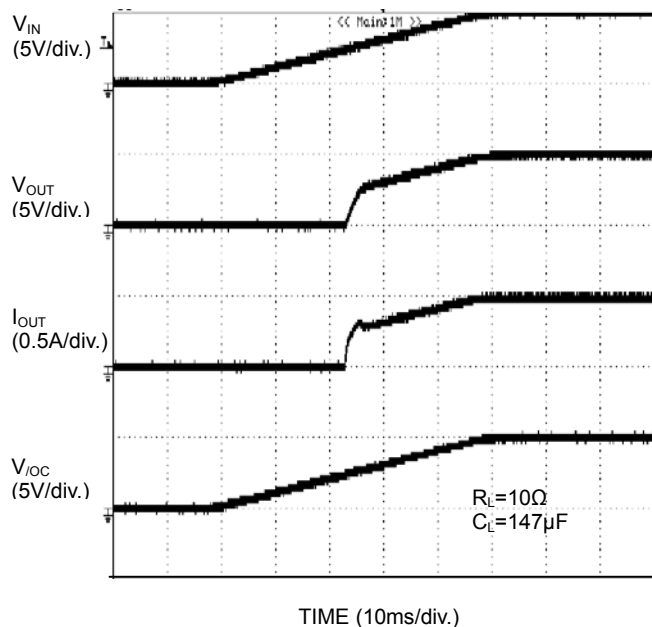
Figure 36. UVLO 特性 V_{IN} 上昇時 (BD2041AFJ)
