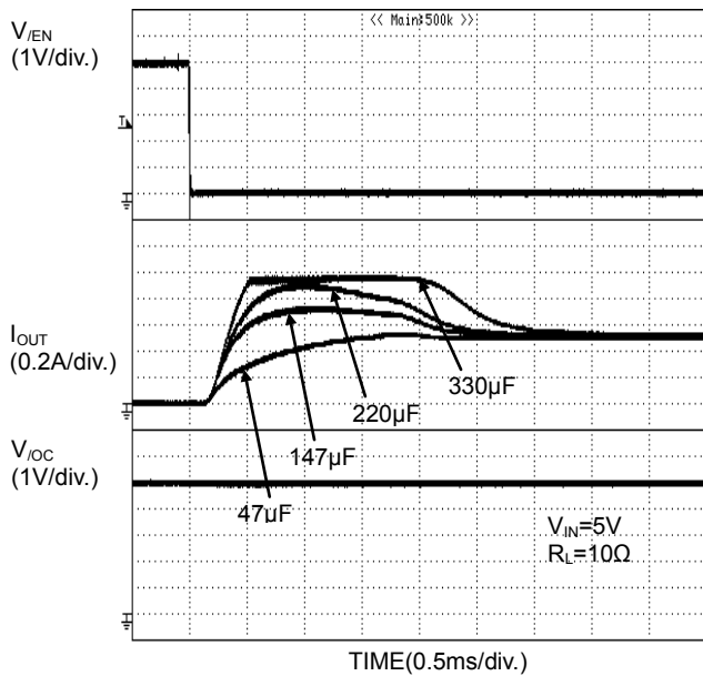
Figure 30. 突入電流特性 (BD2041AFJ)
