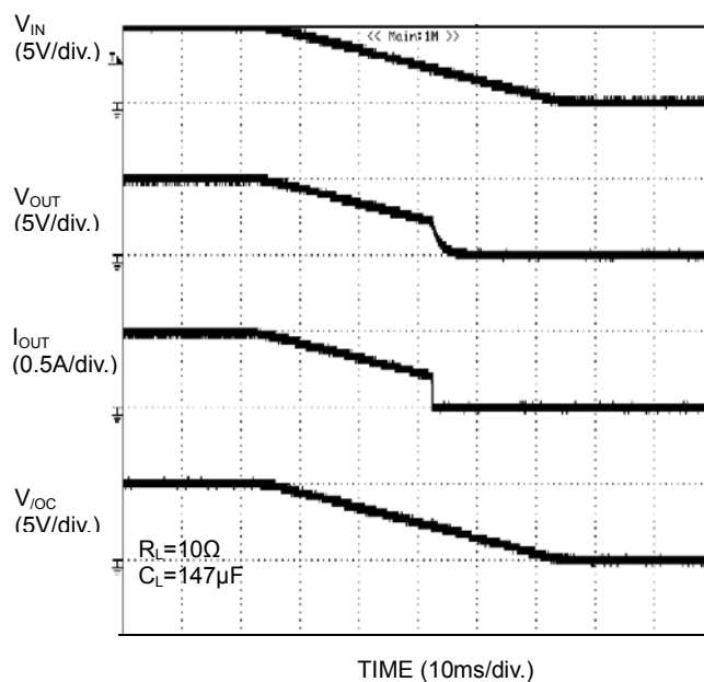
Figure 37. UVLO 特性 V_{IN} 下降時 (BD2041AFJ)
