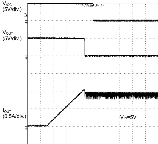
TIME(2ms/div.) Figure 32. 過電流検出特性 ランプ出力 (BD2041AFJ)
