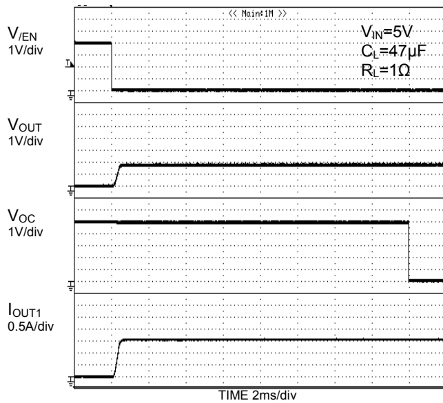
Figure 36. 過電流検出特性 出力1Ω負荷状態でEnable (BD2062FJ)
