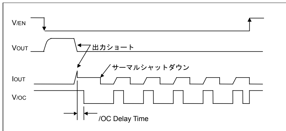
Figure 38. 過電流検出、サーマルシャットダウンタイミング (BD2062FJ)
