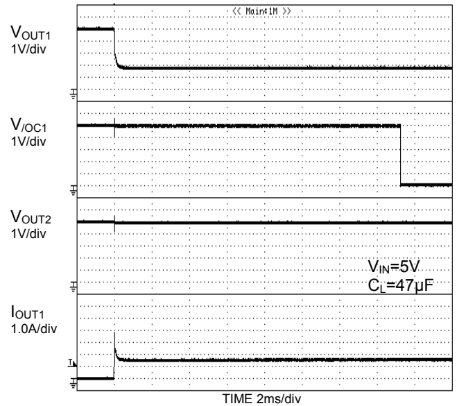
Figure 35. 過電流検出特性 Enable時に1Ωショート (BD2062FJ)
