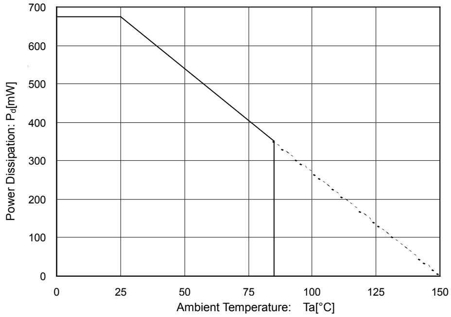
Figure 40. パッケージ熱損失について(Pd-Ta Curve)
