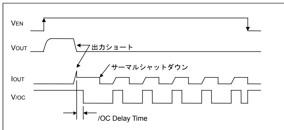
Figure 39. 過電流検出、サーマルシャットダウンタイミング (BD2066FJ)
