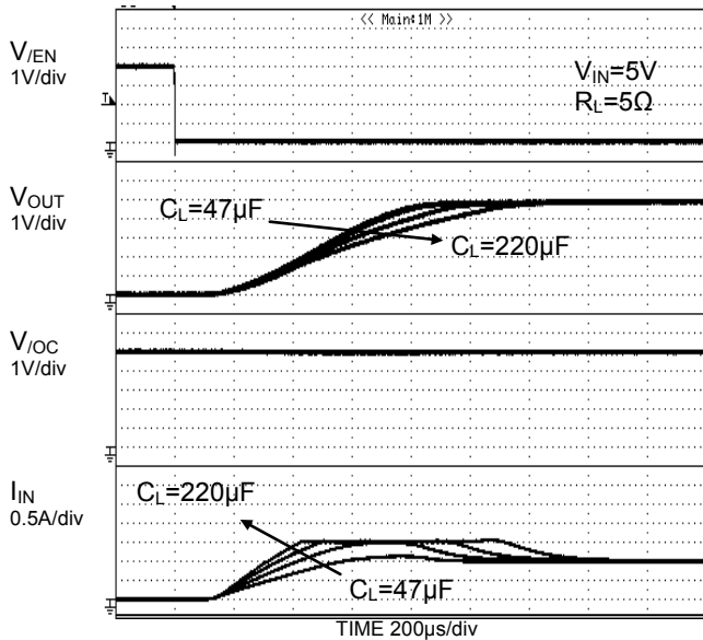
Figure 32. 突入電流特性 C_L=47\mu F, 100\mu F, 147\mu F, 220\mu F (BD2062FJ)
