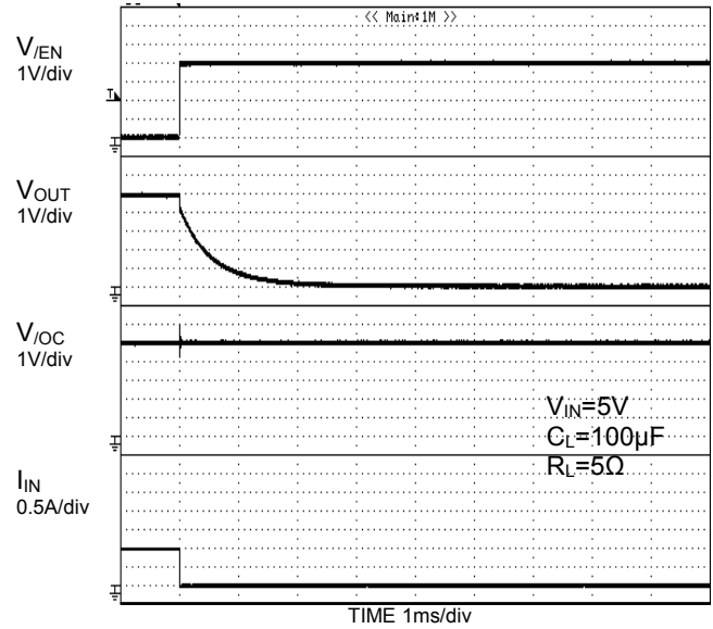
Figure 31. 出力立ち下がり特性 (BD2062FJ)
