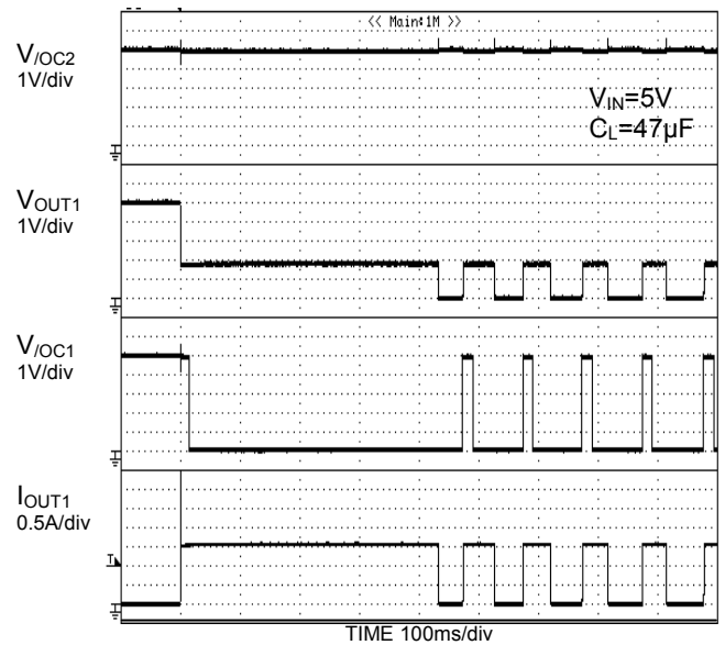
Figure 37. サーマル シャットダウン動作 (BD2062FJ)
