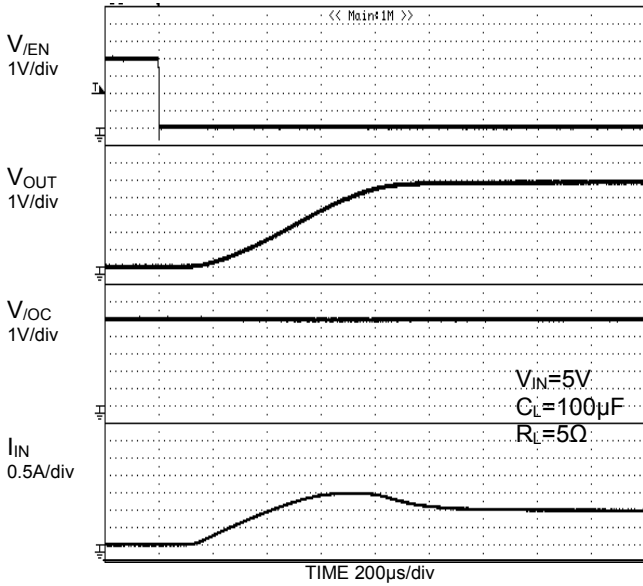
Figure 30. 出力立ち上がり特性 (BD2062FJ)
