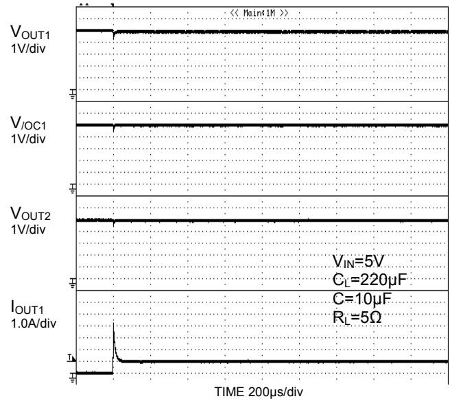
Figure 33. 突入電流特性 (BD2062FJ)
