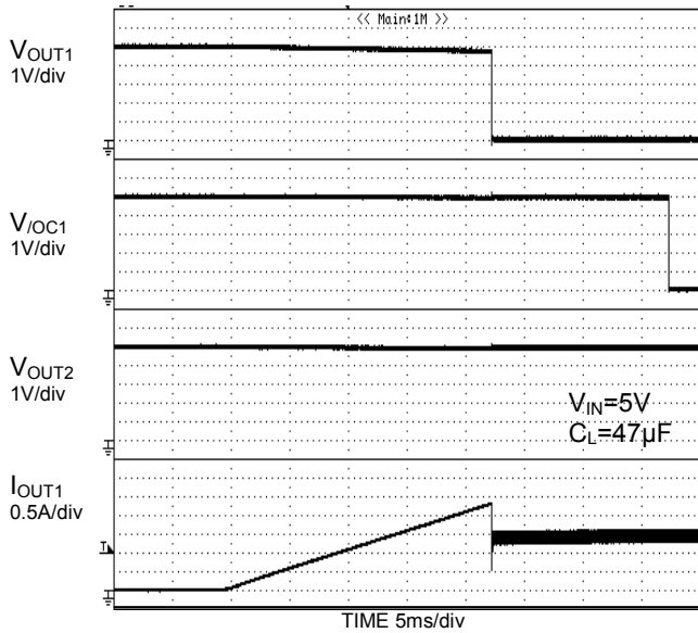
Figure 34. 過電流検出特性 ランプ出力 (BD2062FJ)
