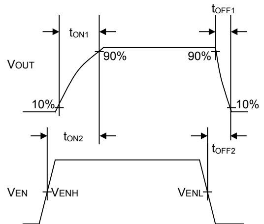
Figure 3. タイミングダイアグラム(BD2066FJ)
