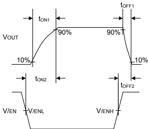
Figure 2. タイミングダイアグラム(BD2062FJ)
