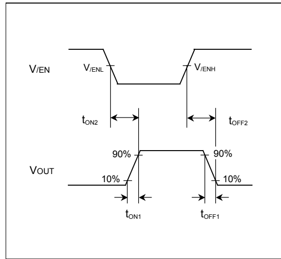
Figure 3. 出力立上り時間、出力立下り時間 (BD2233G)
