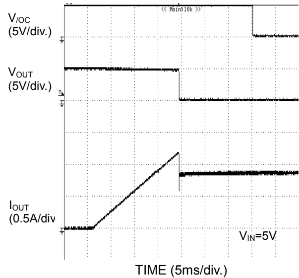
Figure 35. 過電流検出特性 ランプ出力
