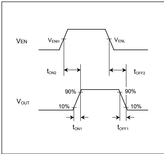
Figure 2. 出力立上り時間、出力立下り時間 (BD2232G)
