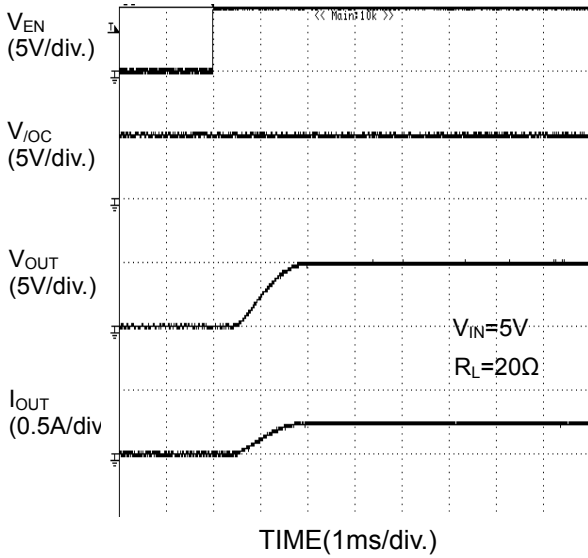
Figure 32. 出力立ち上がり特性
