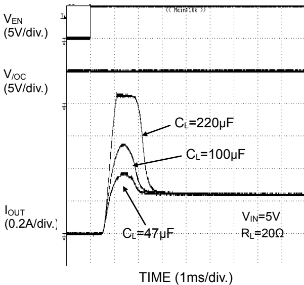
Figure 34. 突入電流特性
