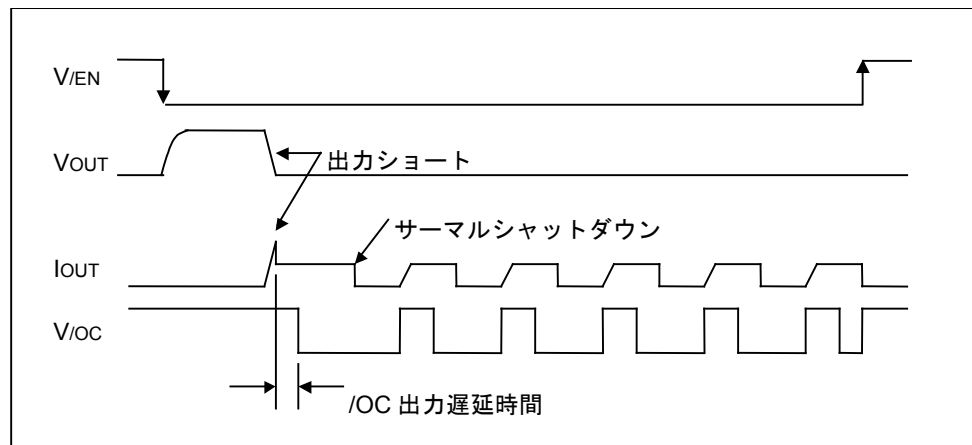
Figure 43. 過電流検出、サーマルシャットダウンタイミング (BD2233G)
