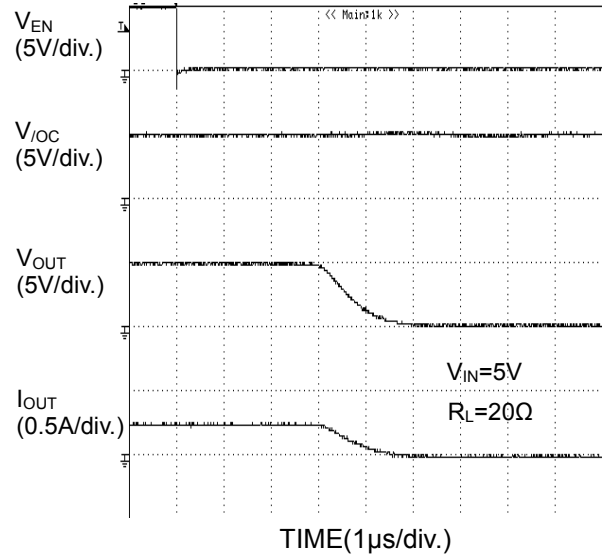
Figure 33. 出力立ち下がり特性
