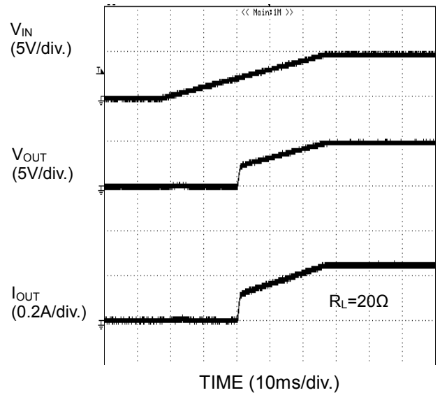
Figure 39. UVLO 特性 V_{IN} 上昇時
