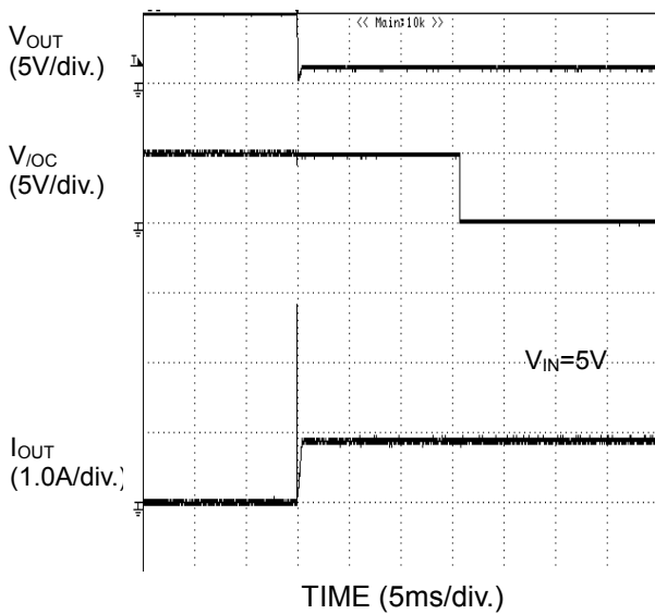
Figure 38. 過電流検出特性 Enable 時に出力 1Ω ショート
