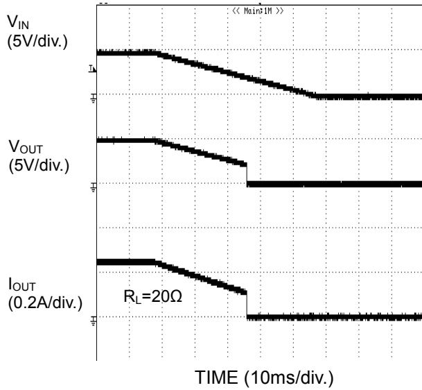
Figure 40. UVLO 特性 V_{IN} 下降時
