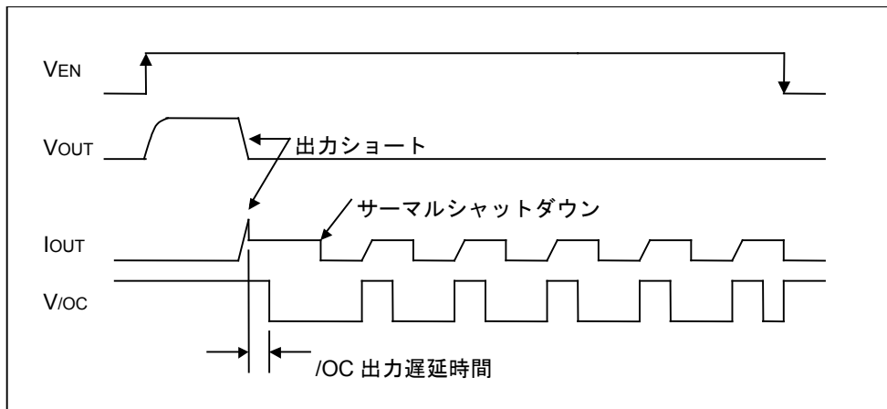
Figure 42. 過電流検出、サーマルシャットダウンタイミング (BD2232G)
