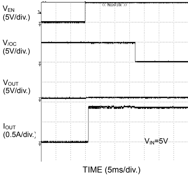
Figure 36. 過電流検出特性 ショート状態への Enable
