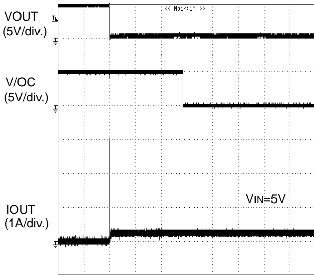
TIME (5ms/div.) Figure 38. 過電流検出特性 Enable に出力 1Ω ショート
