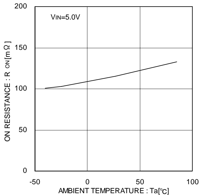
Figure 13. オン抵抗
