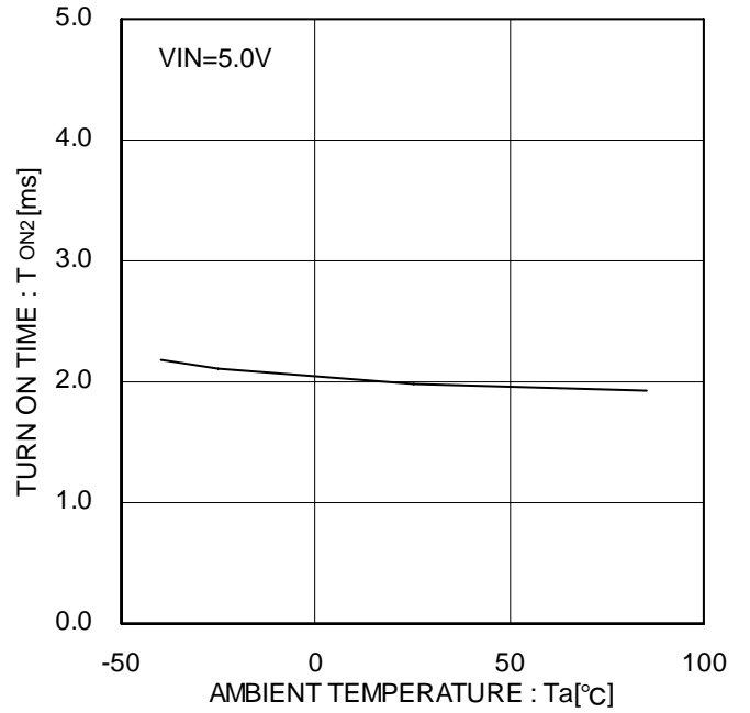
Figure 23. 出力立ち上がり遅延時間
