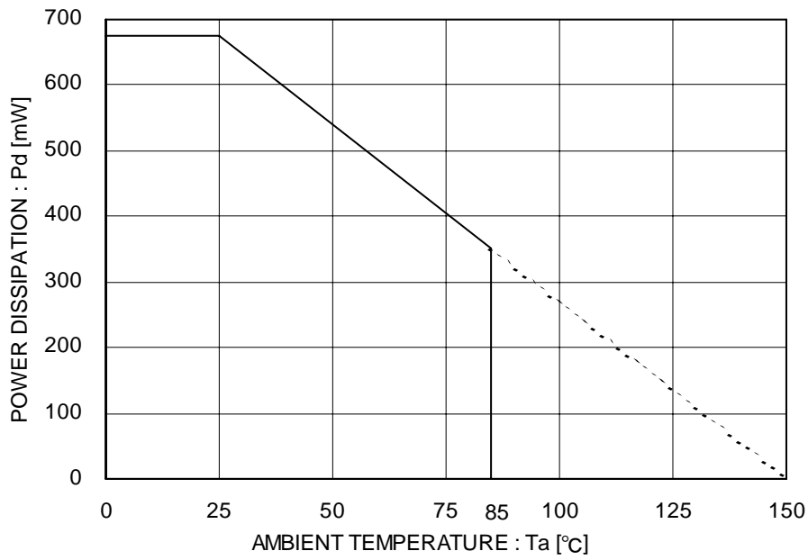
Figure 44. パッケージ熱軽減曲線 (Pd-Ta Curve)
