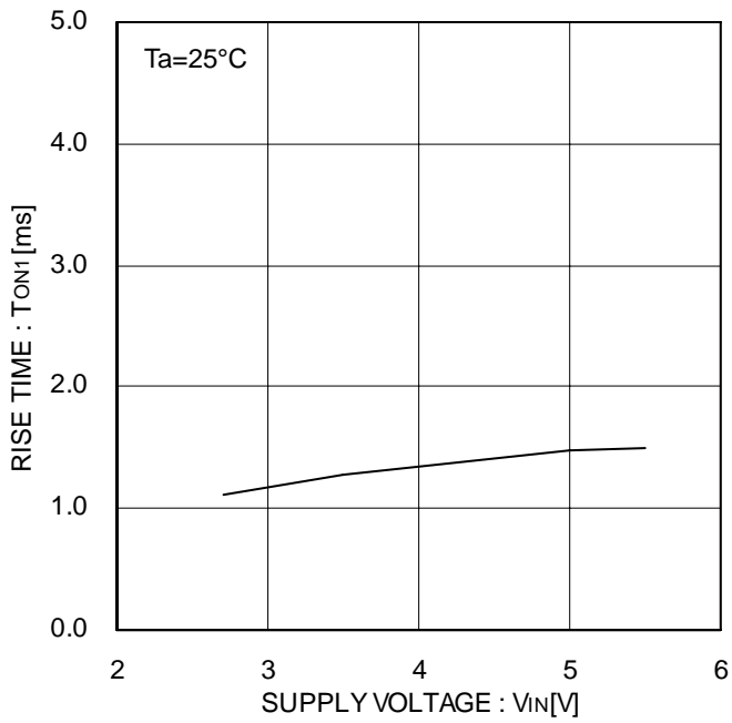
Figure 20. 出力立ち上がり時間
