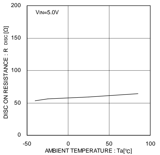
Figure 31. 出力ディスチャージ抵抗
