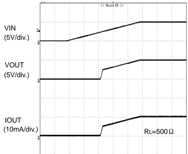
TIME (5ms/div.) Figure 39. UVLO 特性 VIN 上昇時
