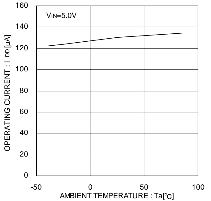
Figure 7. 動作電流 EN enable
