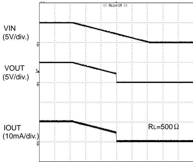
TIME (10ms/div.) Figure 40. UVLO 特性 VIN 下降時
