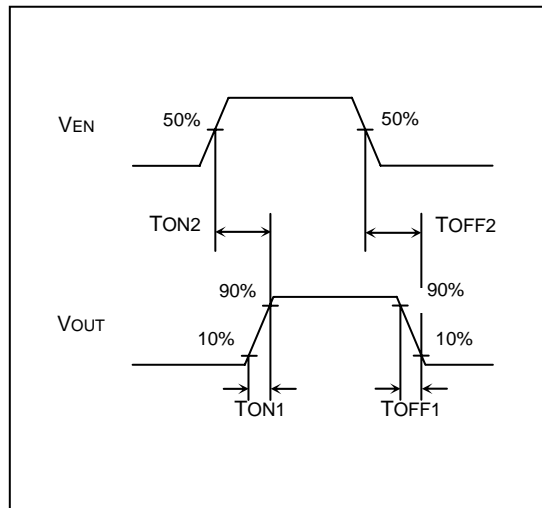
Figure 5. 出力立ち上がり時間、立ち下がり時間
