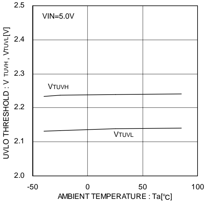
Figure 18. UVLO スレッシュホールド
