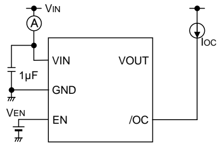
/OC 出力 Low 電圧
