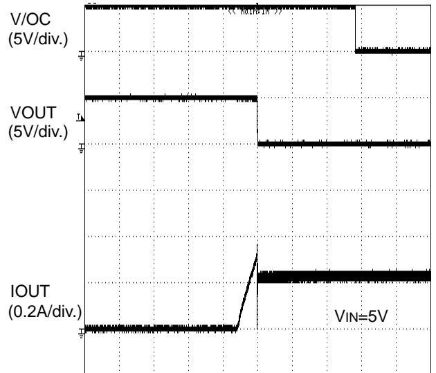
Figure 35. 過電流検出特性 ランプ出力
