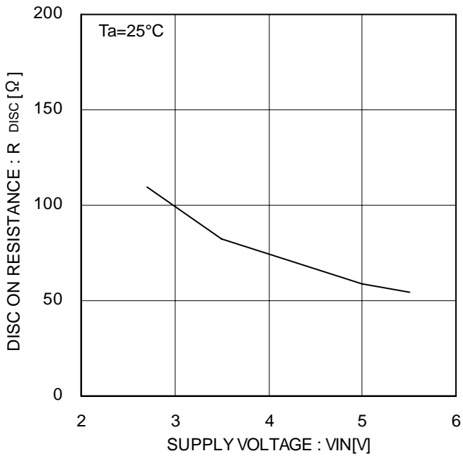
Figure 30. 出力ディスチャージ抵抗
