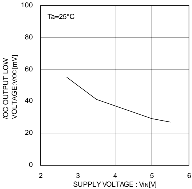
Figure 16. /OC 出力 Low 電圧
