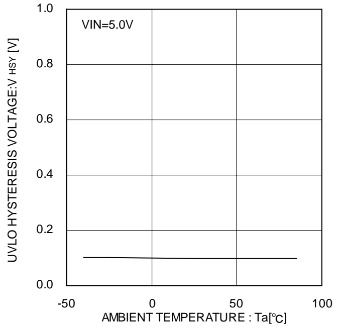
Figure 19. UVLO ヒステリシス電圧
