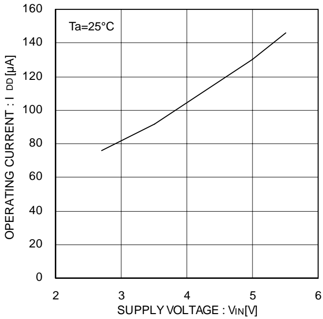
Figure 6. 動作電流 EN enable
