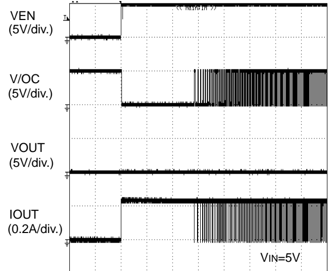
TIME (500ms/div.) Figure 37. 過電流検出特性 ショート状態への Enable
