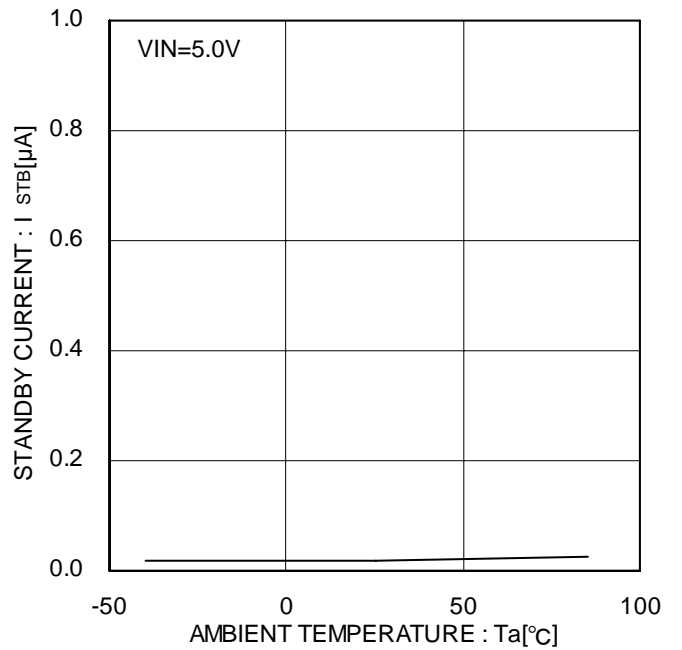
Figure 9. 静止消費電流 EN disable
