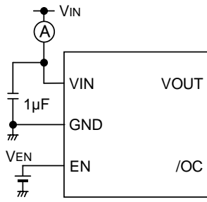
動作電流
