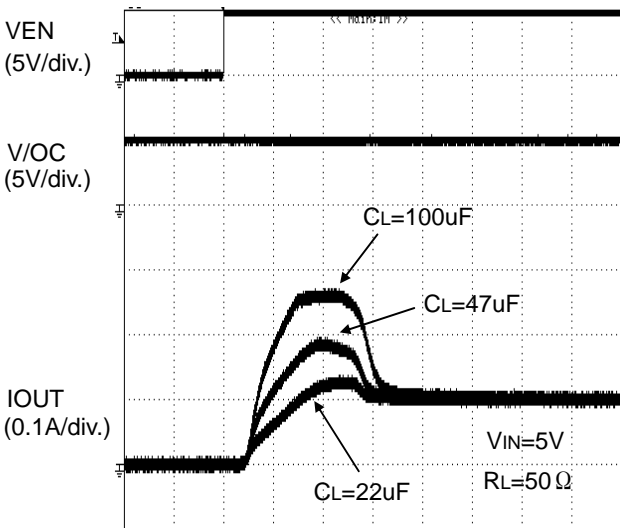
Figure 34. 突入電流特性
