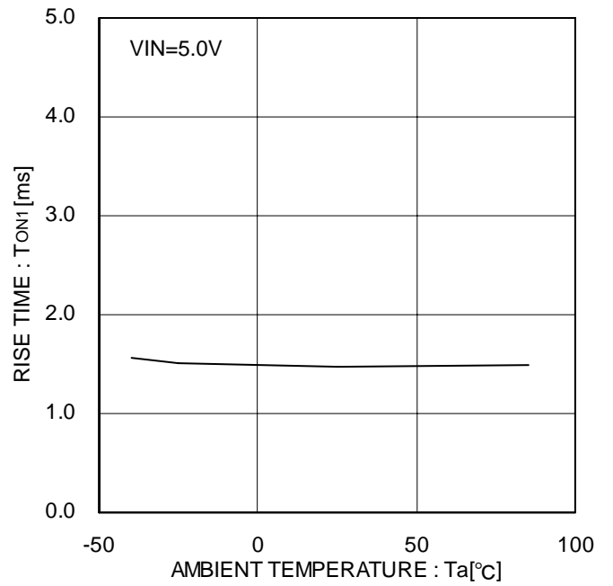
Figure 21. 出力立ち上がり時間
