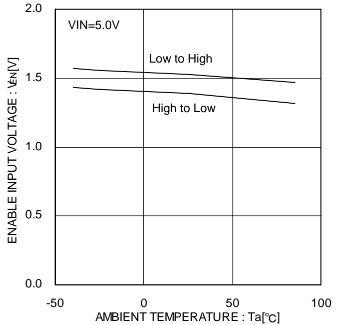
Figure 11. EN 入力電圧
