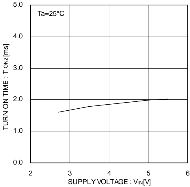
Figure 22. 出力立ち上がり遅延時間
