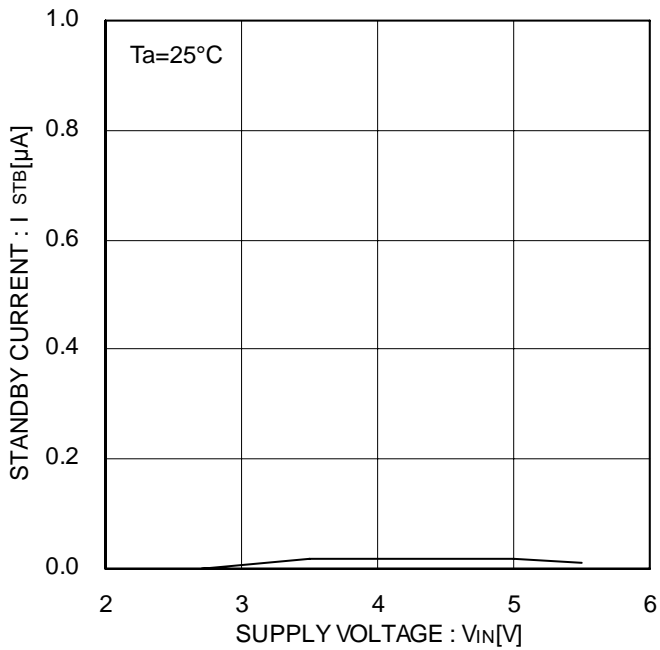
Figure 8. 静止消費電流 EN disable
