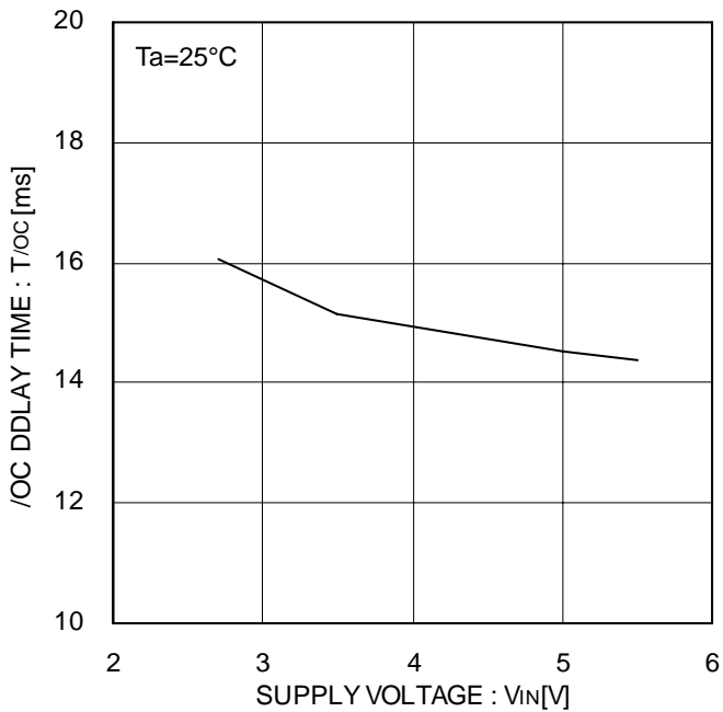
Figure 28. /OC 出力遅延時間
