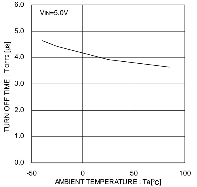
Figure 27. 出力立ち下がり遅延時間
