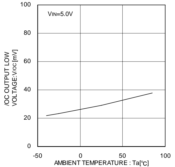
Figure 17. /OC 出力 Low 電圧
