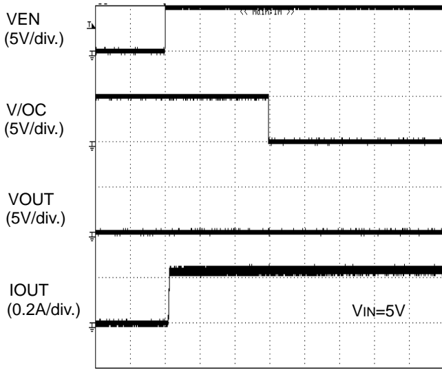
TIME (5ms/div.) Figure 36. 過電流検出特性 ショート状態への Enable
