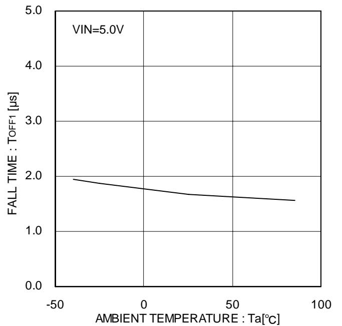
Figure 25. 出力立ち下がり時間
