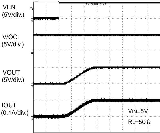
Figure 32. 出力立ち上がり時間
