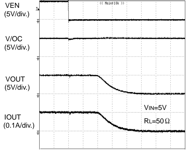
Figure 33. 出力立ち上がり時間
