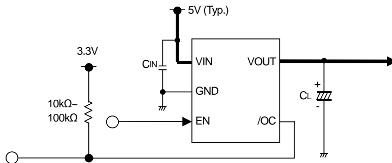
Figure 1. 基本アプリケーション回路
