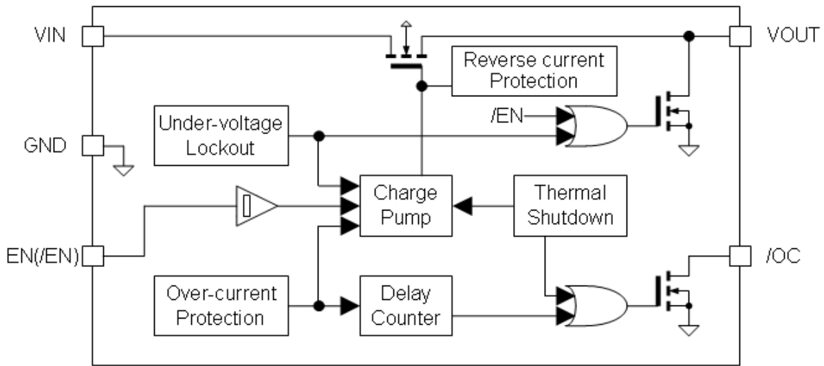
Figure 2. ブロック図
