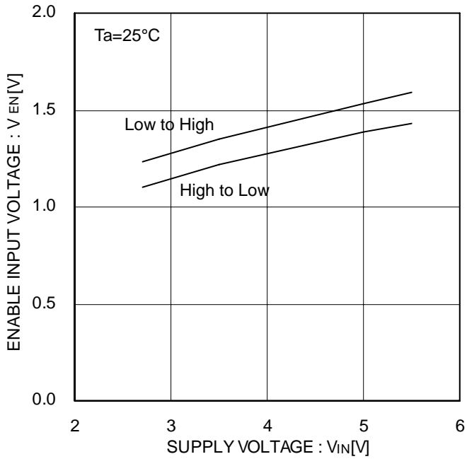
Figure 10. EN 入力電圧
