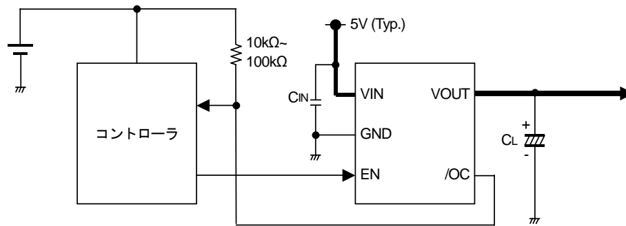
Figure 41. 応用回路例
