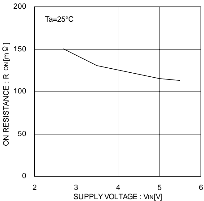
Figure 12. オン抵抗
