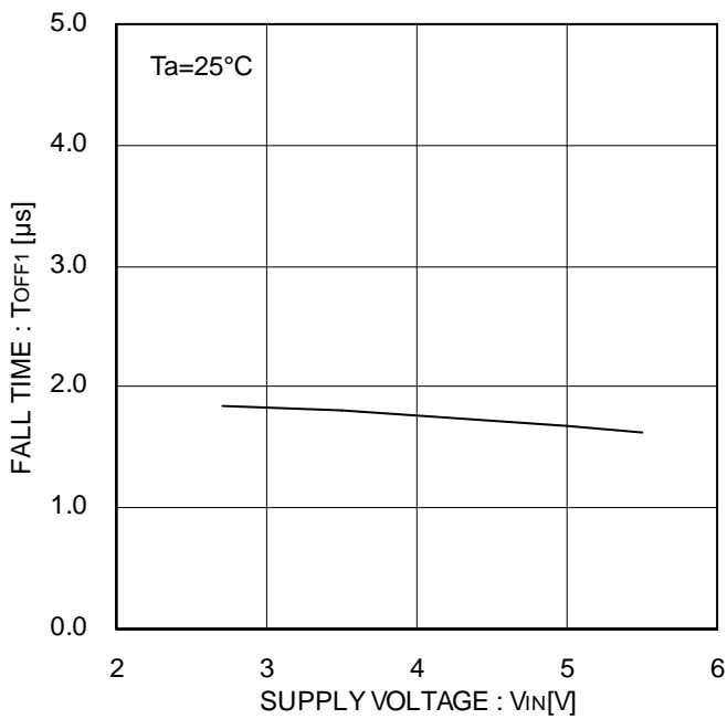
Figure 24. 出力立ち下がり時間
