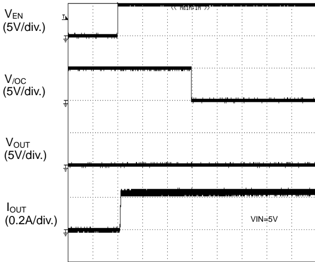
TIME (5ms/div.) Figure 58. 過電流検出特性 ショート状態への Enable
