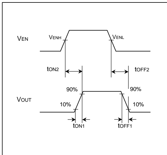
Figure 2. 出力立上り時間、立下り時間 (BD2262G-M, BD2264G-M, BD2266G-M)
