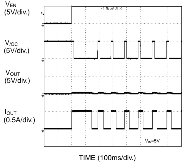
Figure 68. 過電流検出特性 ショート状態への Enable
