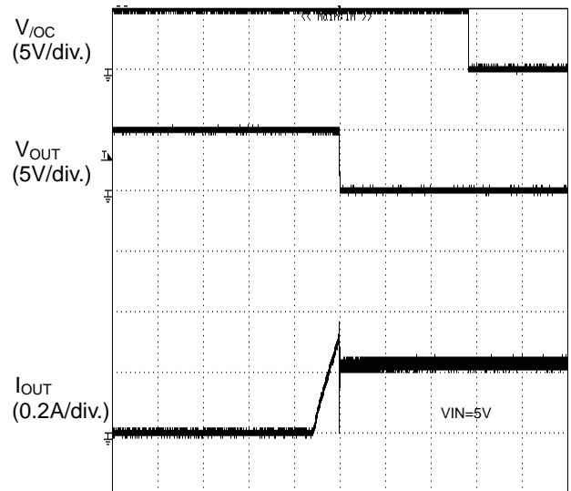
TIME (5ms/div.) Figure 57. 過電流検出特性 ランプ出力
