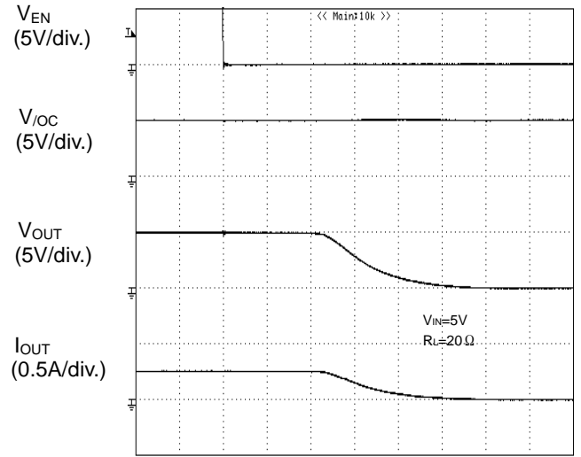
TIME (1μs/div.) Figure 73. 出力立ち下り特性
