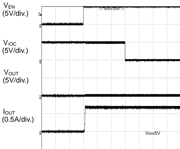
TIME (5ms/div.) Figure 76. 過電流検出特性 ショート状態への Enable
