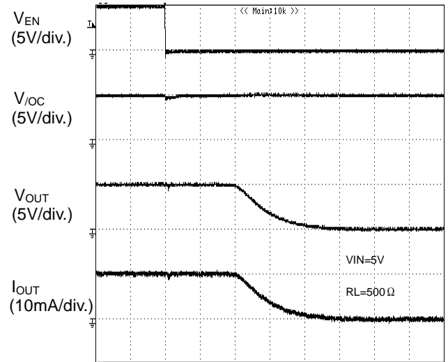
TIME (1us/div.) Figure 55. 出力立下り特性
