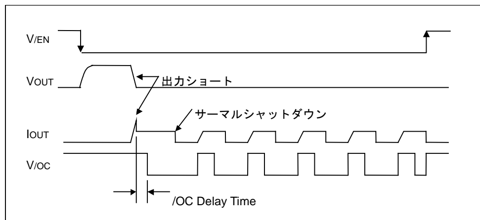
Figure 83. 過電流検出、サーマルシャットダウンタイミング (BD2265G-M, BD2267G-M)
