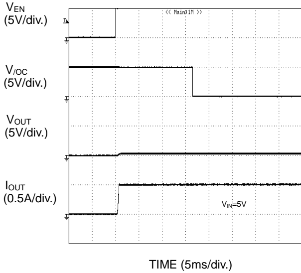
Figure 67. 過電流検出特性 ショート状態への Enable
