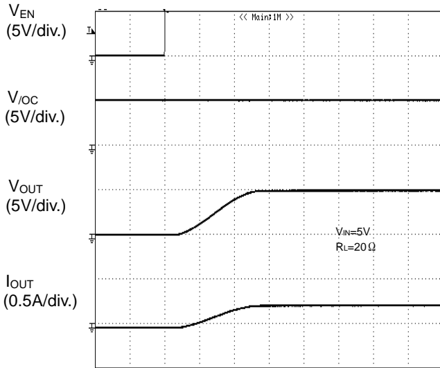
TIME (1ms/div.) Figure 72. 出力立ち上がり特性
