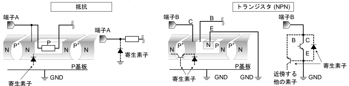
Figure 85. モノリシック IC 構造例
