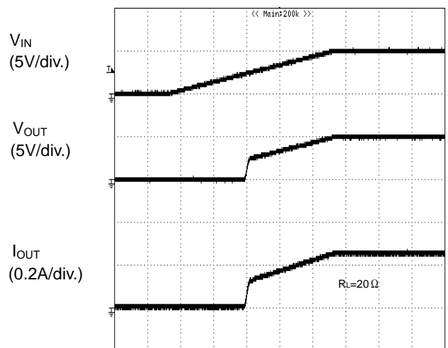
TIME (10ms/div.) Figure 79. UVLO 特性 V_{IN} 上昇時
