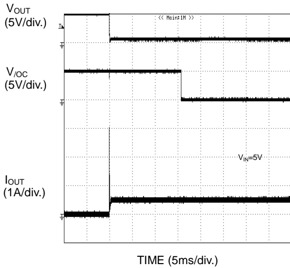
Figure 69. 過電流検出特性 Enable 時に出力 1Ω ショート
