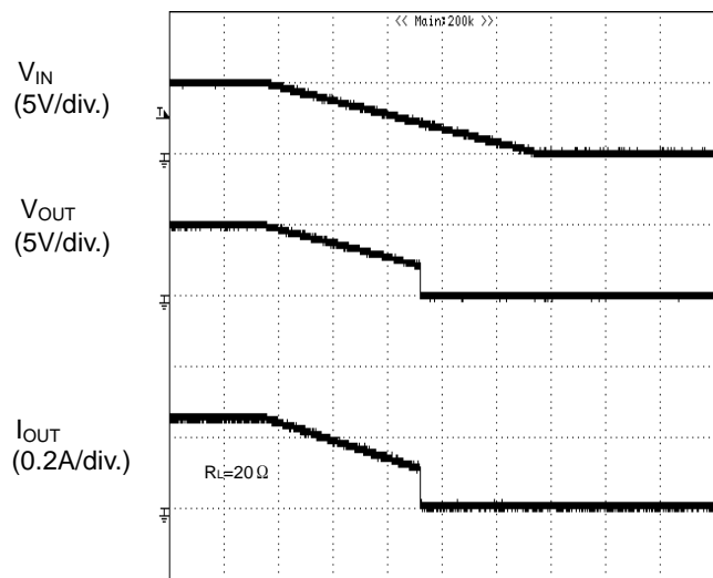
TIME (10ms/div.) Figure 80. UVLO 特性 V_{IN} 下降時
