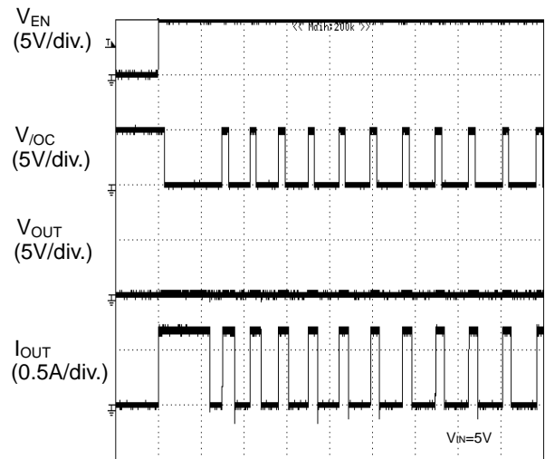
TIME (100ms/div.) Figure 77. 過電流検出特性 ショート状態への Enable
