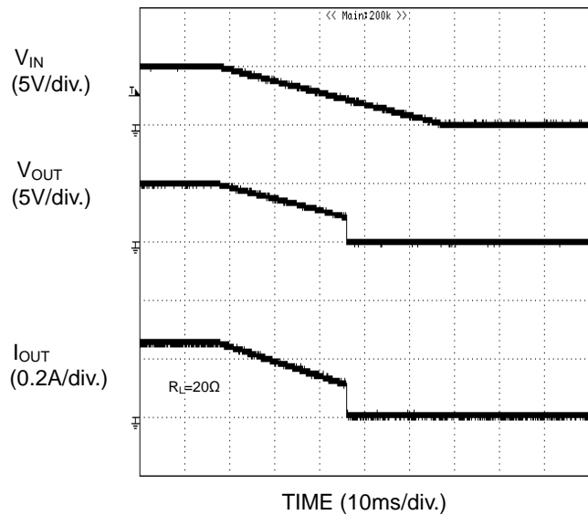
Figure 71. UVLO 特性 V_{IN} 下降時
