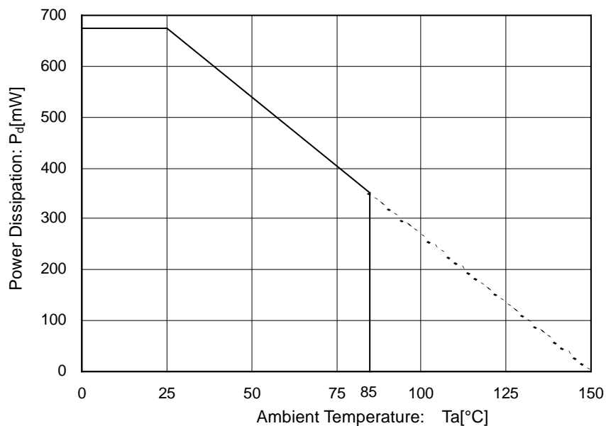
Figure 84. パッケージ熱損失について (Pd-Ta Curve)
