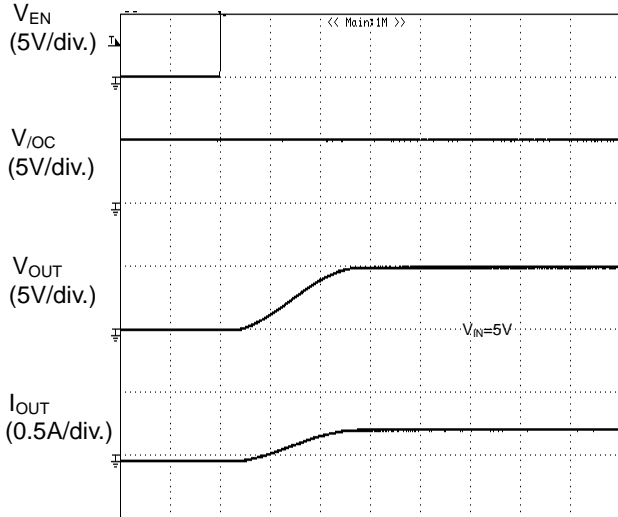
TIME (1ms/div.)
