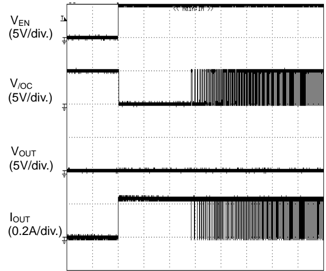
TIME (500ms/div.) Figure 59. 過電流検出特性 ショート状態への Enable
