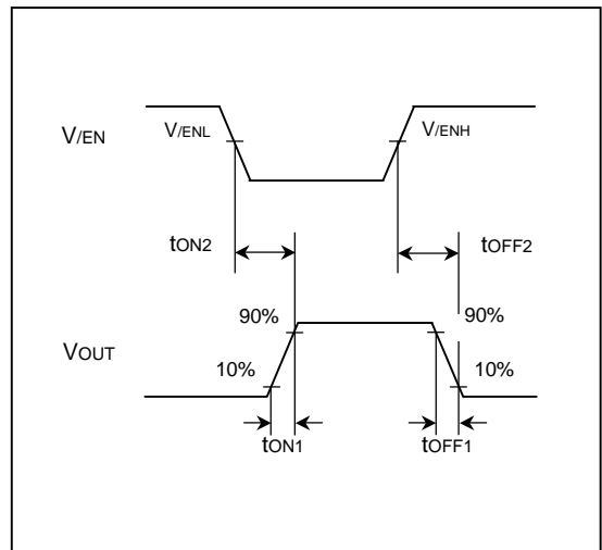
Figure 3. 出力立上り時間、立下り時間 (BD2265G-M, BD2267G-M)
