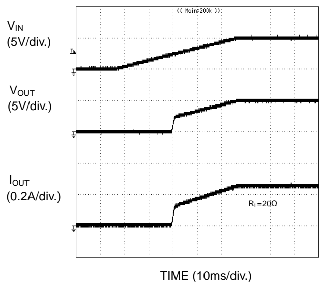
Figure 70. UVLO 特性 V_{IN} 上昇時
