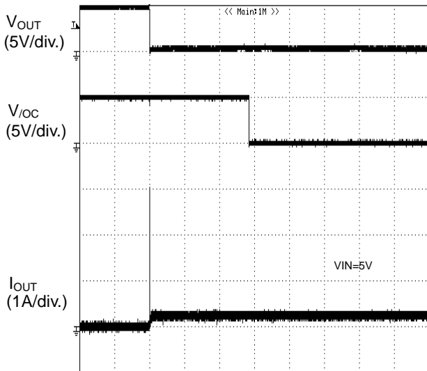
TIME (5ms/div.) Figure 60. 過電流検出特性 Enable 時に出力 1Ω ショート
