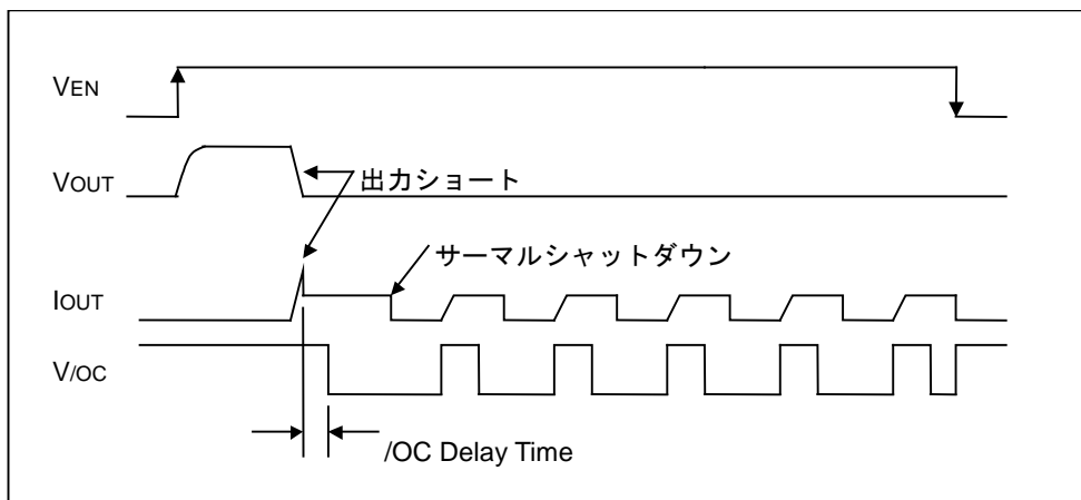
Figure 82. 過電流検出、サーマルシャットダウンタイミング (BD2262G-M, BD2264G-M, BD2266G-M)
