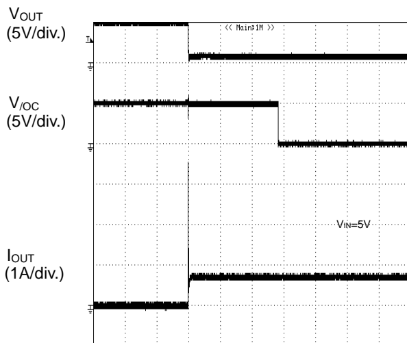
TIME (5ms/div.) Figure 78. 過電流検出特性 Enable 時に出力 1Ω ショート
