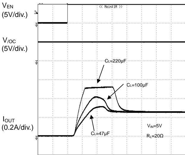
TIME (1ms/div.)
