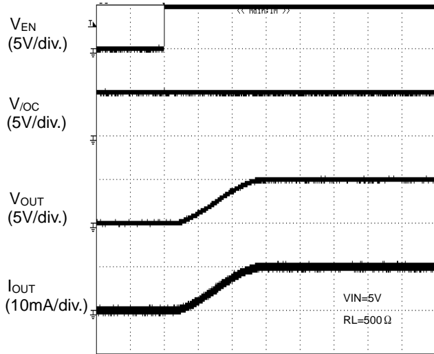
TIME (1ms/div.) Figure 54. 出力立上り特性
