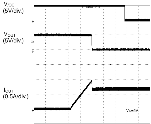
TIME (5ms/div.) Figure 75. 過電流検出特性 ランプ出力
