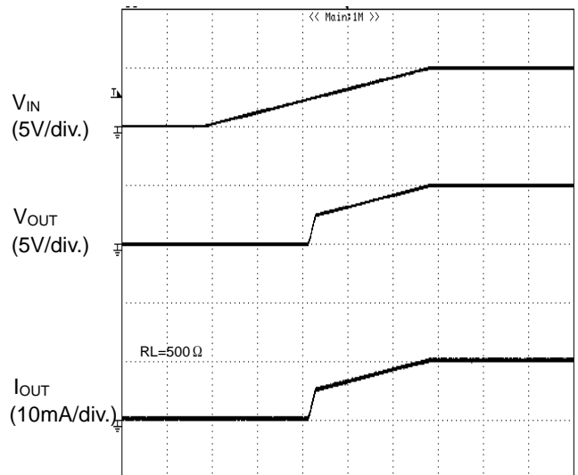
TIME (5ms/div.) Figure 61. UVLO 特性 V IN 上昇時
