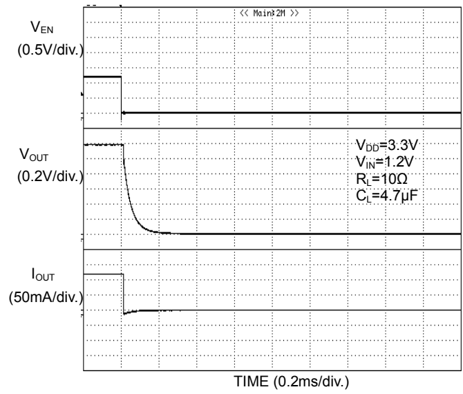
Figure 28. 出力立ち下がり特性 BD6528HFV
