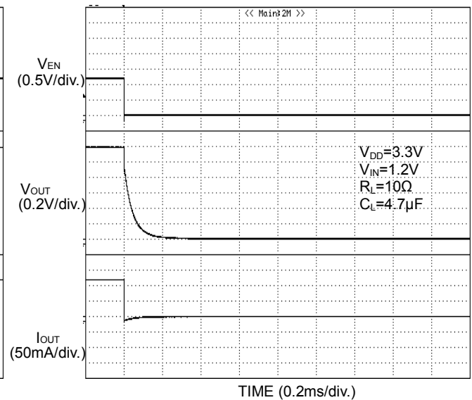
Figure 32. 出力立ち下がり特性 BD6529GUL
