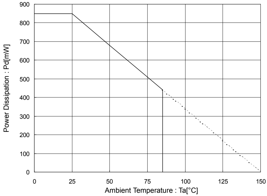
Figure 35. パッケージ熱損失について(Pd-Ta Curve) 70mm * 70mm * 1.6mm ガラスエポキシ基板実装時 (HVSO6)
