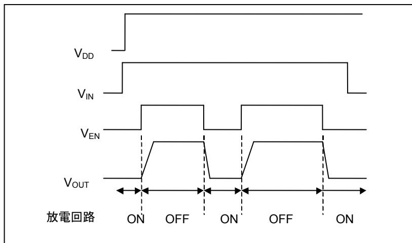
Figure 34. 動作タイミング
