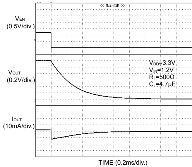
Figure 30. 出力立ち下がり特性 BD6529GUL
