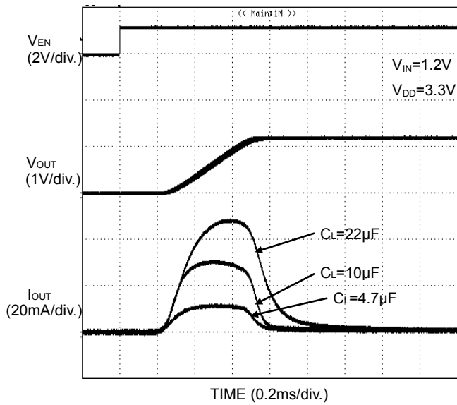
Figure 33. 突入電流特性
