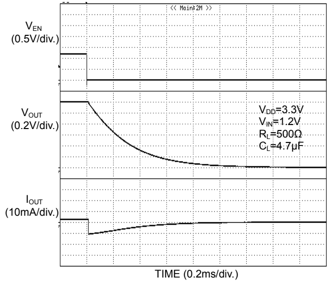
Figure 26. 出力立ち下がり特性 BD6528HFV
