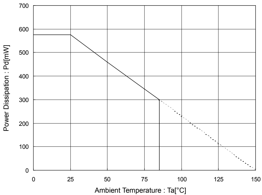
Figure 36. パッケージ熱損失について(Pd-Ta Curve) 50mm x 58mm x 1.75mm ガラスエポキシ基板実装時 (VCSP50L1)
