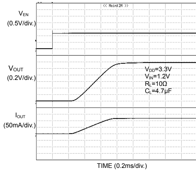
Figure 27. 出力立ち上がり特性 BD6528HFV
