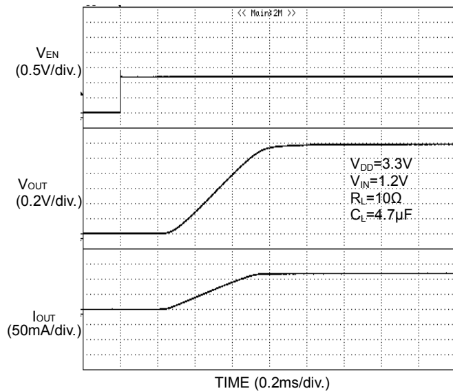
Figure 31. 出力立ち上がり特性 BD6529GUL
