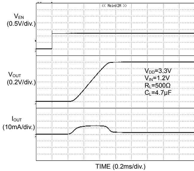
Figure 29. 出力立ち上がり特性 BD6529GUL
