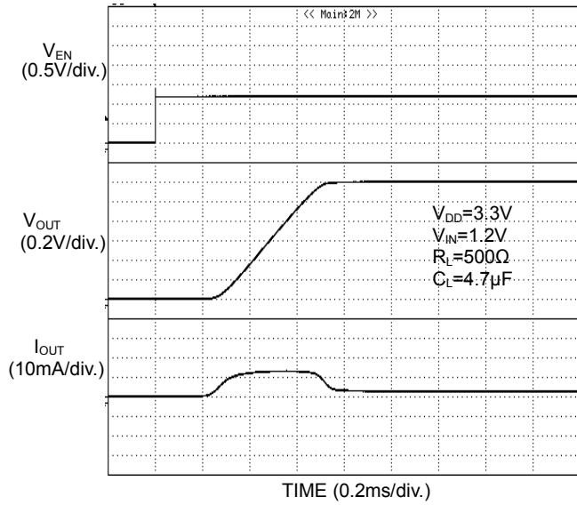
Figure 25. 出力立ち上がり特性 BD6528HFV
