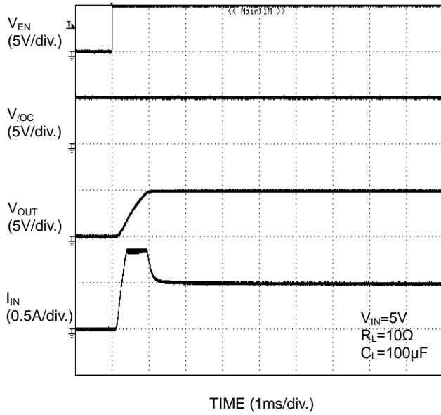
Figure 30. 出力立ち上がり特性
