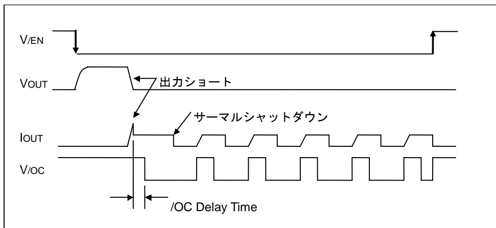
Figure 41. 過電流検出、サーマルシャットダウンタイミング (BD82005FVJ-M)
