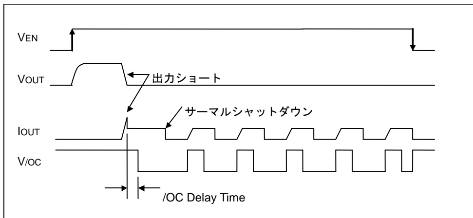
Figure 40. 過電流検出、サーマルシャットダウンタイミング (BD82004FVJ-M)
