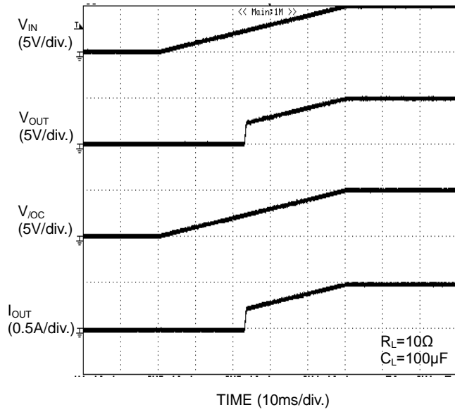
Figure 38. UVLO 特性 V_{IN} 上昇時
