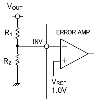
Figure 34. 電圧帰還抵抗設定方法
