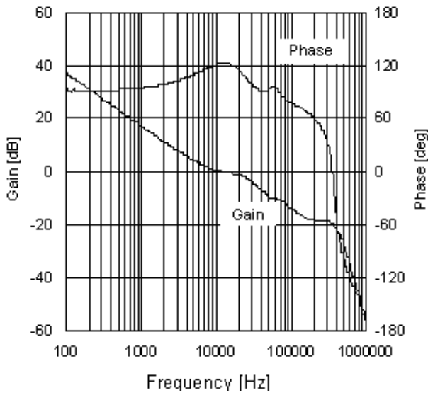
Figure 29. 周波数応答特性 5 ( V_{CC}=4.5V 、 I_o=500mA )
