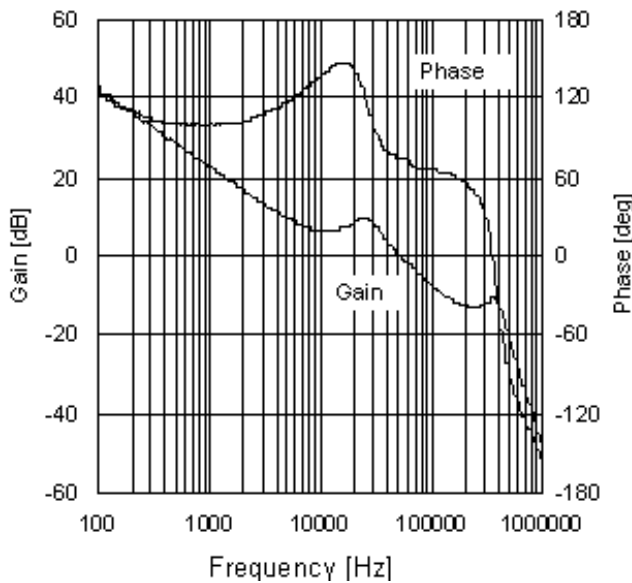
Figure 31. 周波数応答特性 7 ( V_{CC}=8.4V 、 I_o=500mA )
