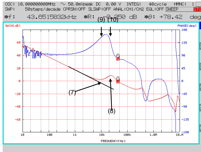
Figure 36. DC/DC コンバータ周波数特性例 (NF 回路ブロック製 FRA5097 にて測定)
