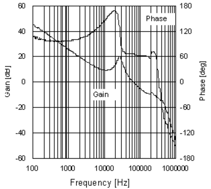
Figure 28. 周波数応答特性 4 ( V_{CC}=10V 、 I_o=250mA )
