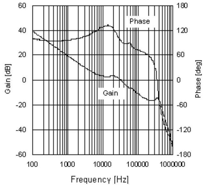
Figure 30. 周波数応答特性 6 ( V_{CC}=6.0V 、 I_o=500mA )
