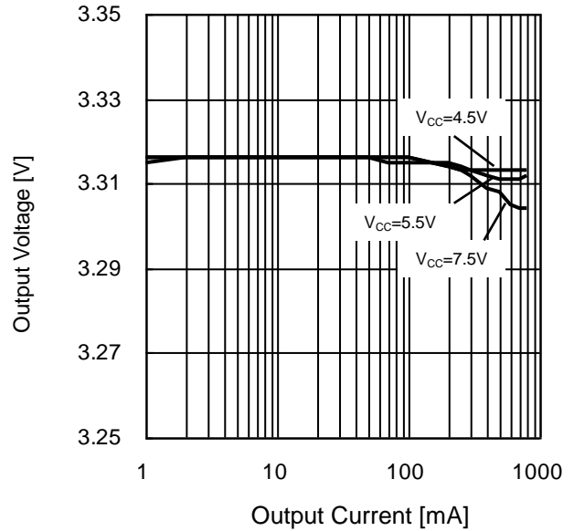
Figure 24. ロードレギュレーション ( V_{OUT}=3.3V )
