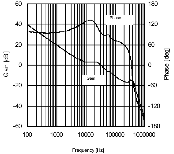
Figure 26. 周波数応答特性 2 ( V_{CC}=6.0V 、 I_o=250mA )
