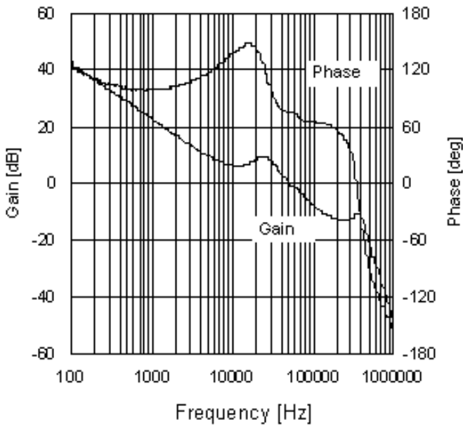
Figure 27. 周波数応答特性 3 ( V_{CC}=8.4V 、 I_o=250mA )
