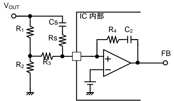
Figure 35. 位相補償設定例
