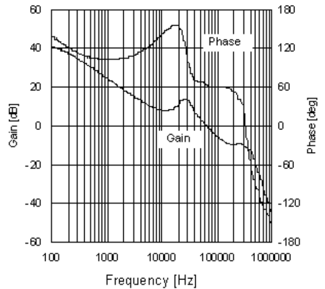
Figure 32. 周波数応答特性 8 ( V_{CC}=10V 、 I_o=500mA )
