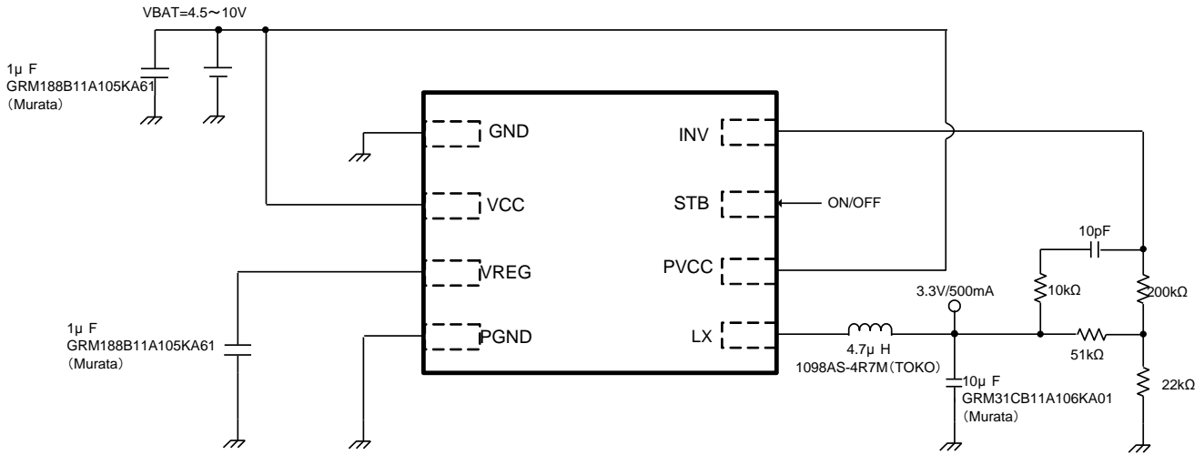
Figure 22. アプリケーション例
