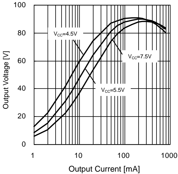
Figure 23. 電力変換効率( V_{OUT}=3.3V )
