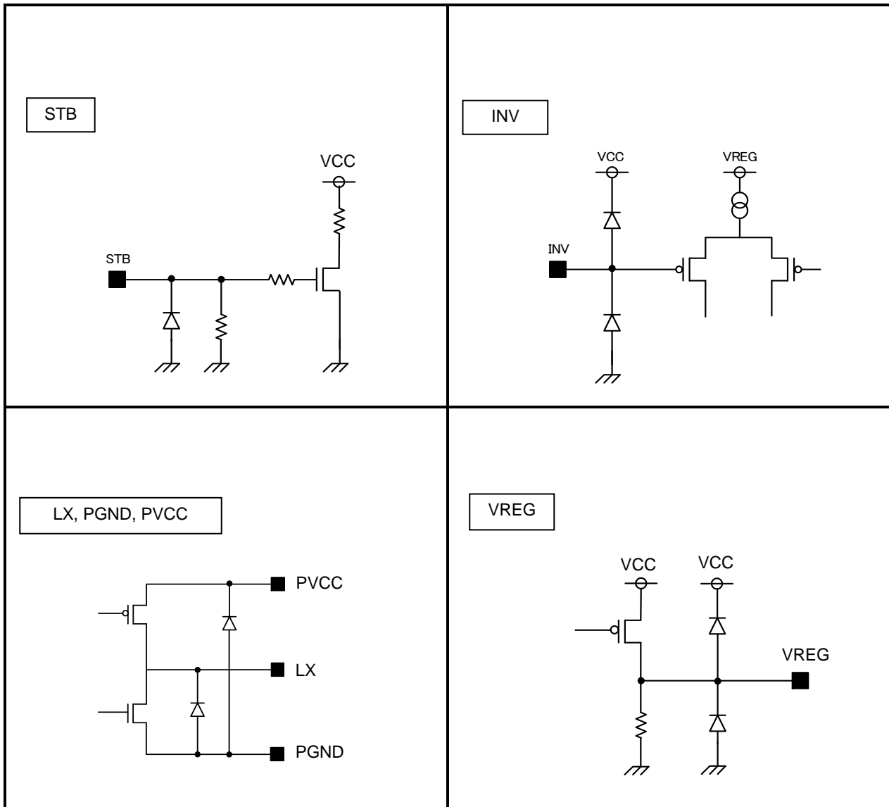
Figure 37. 入出力等価回路図
