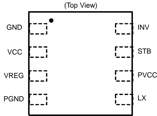
Figure 2. 端子配置図
