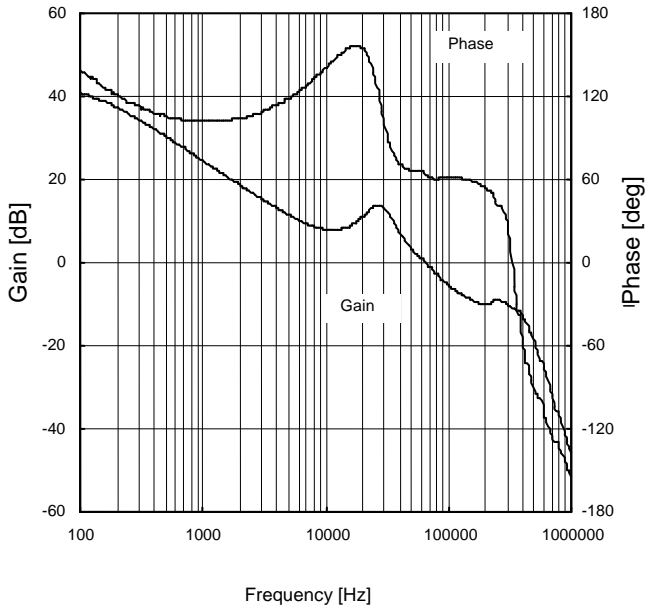
Figure 25. 周波数応答特性 1 ( V_{CC}=4.5V 、 I_o=250mA )
