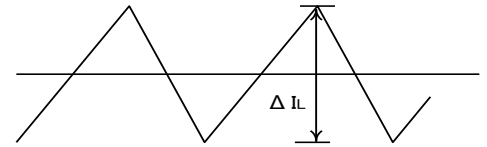
Figure 33. インダクタ電流
