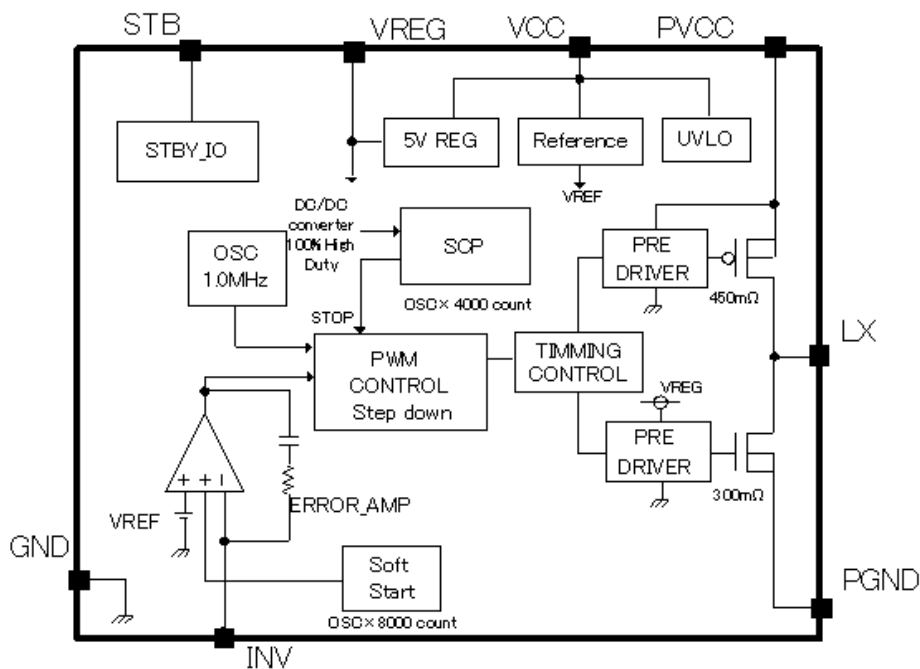
Figure 3. ブロック図
