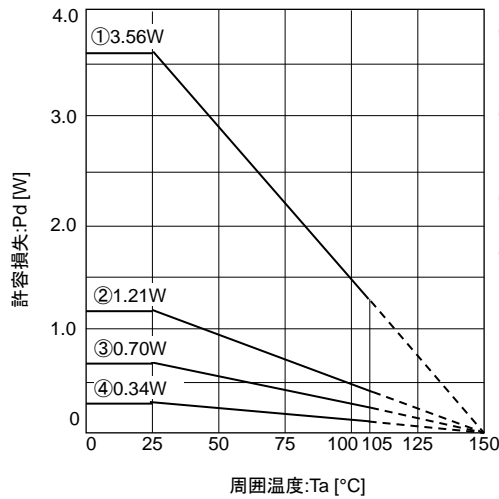
Figure 25. 熱軽減特性 (VQFN020-V4040)
