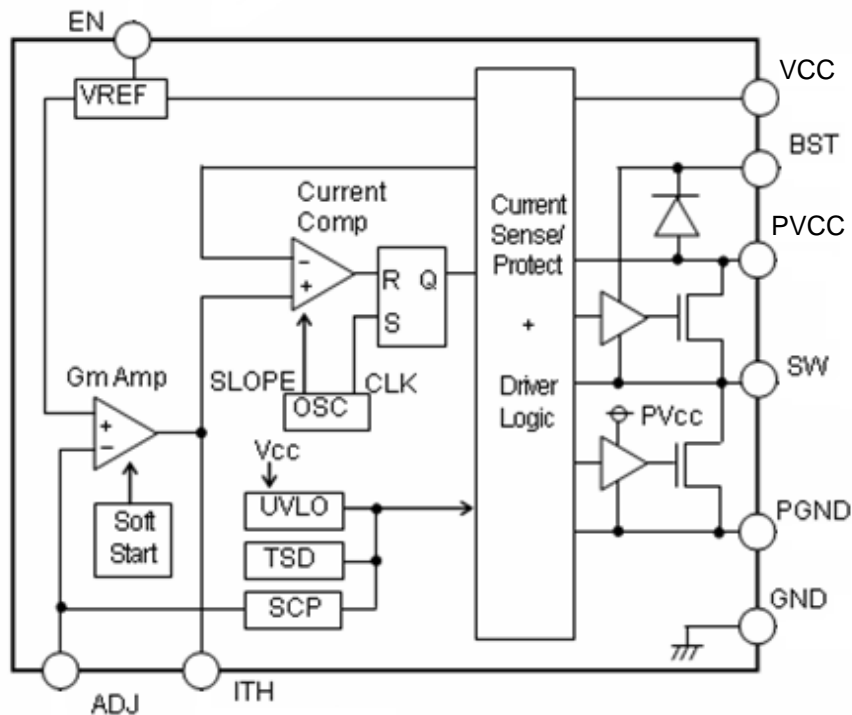
Figure 3. ブロック図
