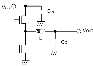
Figure 28. 入力コンデンサ
