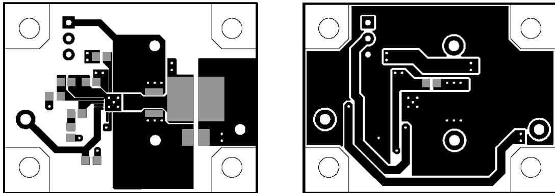
Figure 34. 基板レイアウト簡易図
