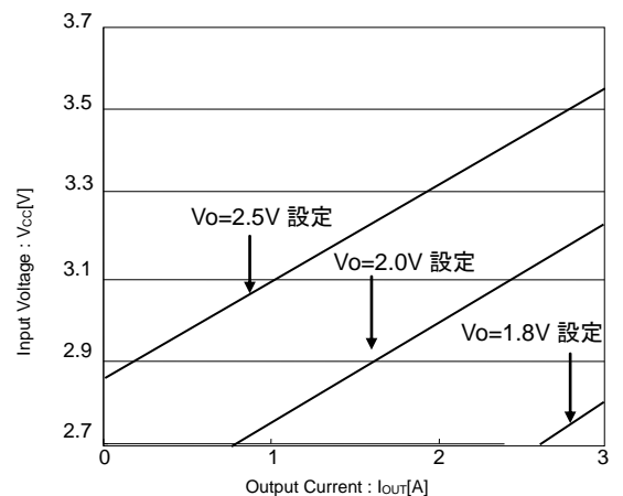
Figure 33. 各出力電圧における必要最低入力電圧
