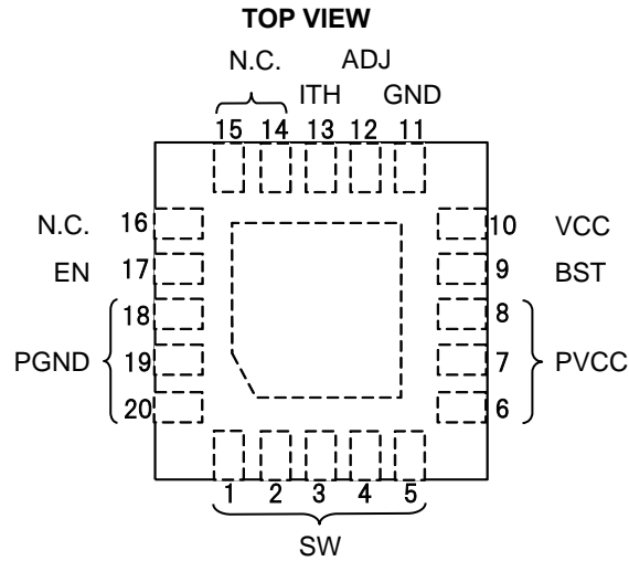
Figure 2. 端子配置図
