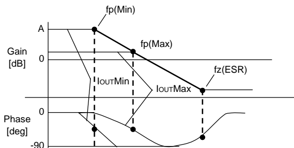
Figure 29. オープンループゲイン特性
