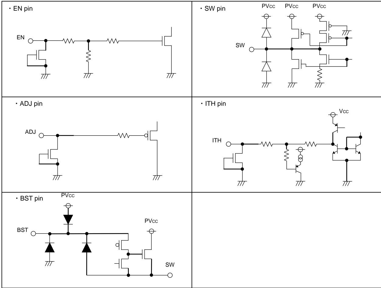
Figure 35. 入出力等価回路図
