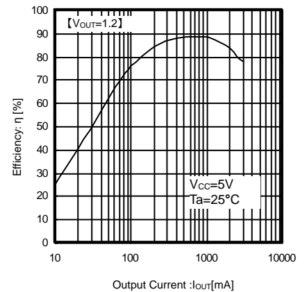
Figure 23. 効率特性
