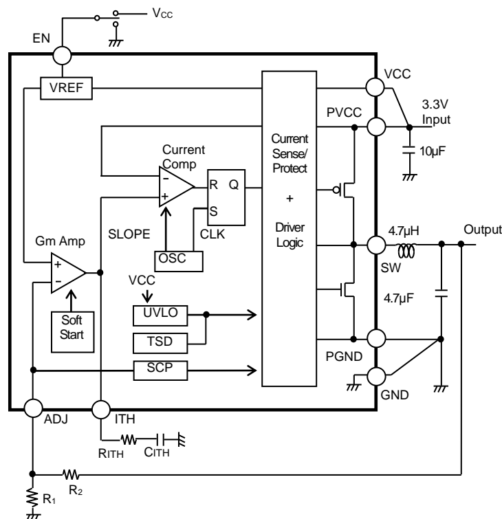
Figure 3. ブロック図
