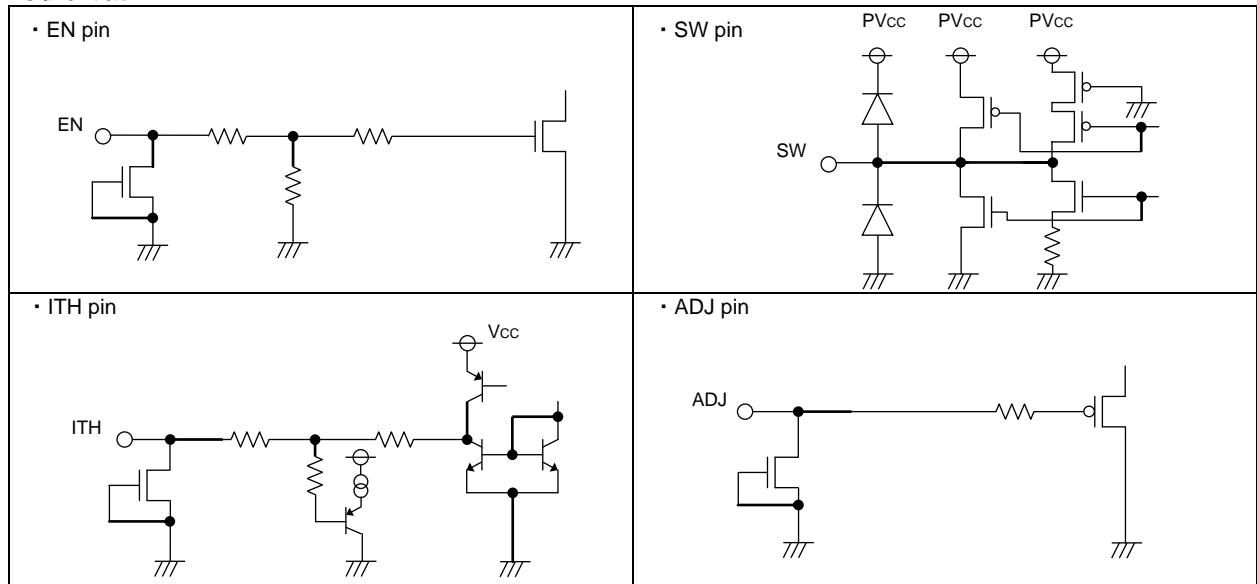
Figure 36. 入出力等価回路図
