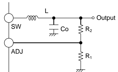
Figure 34. 出力電圧設定抵抗
