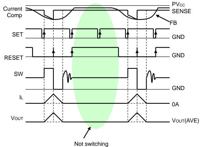
Figure 21. SLLMスイッチングタイミングチャート
