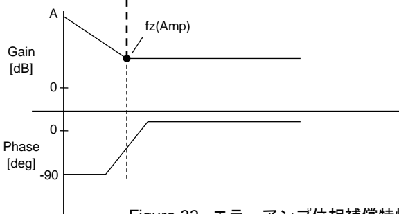
Figure 32. エラーアンプ位相補償特性
