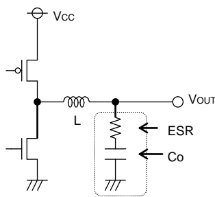
Figure 29. 出力コンデンサ
