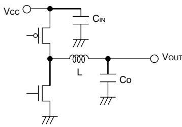
Figure 30. 入力コンデンサ
