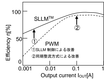
Figure 25. 効率特性
