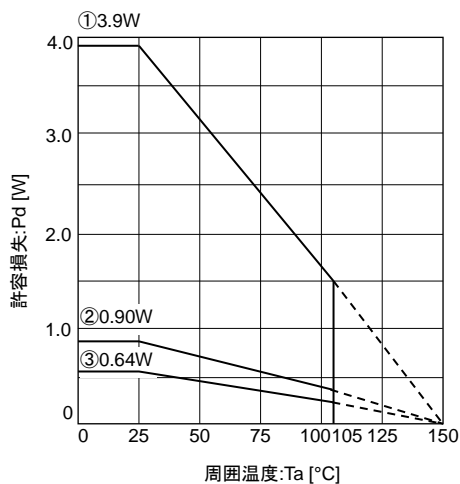
Figure 27. 熱軽減特性 (SON008V5060)
