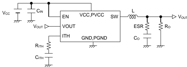
Figure 33. 外付け部品概略図
