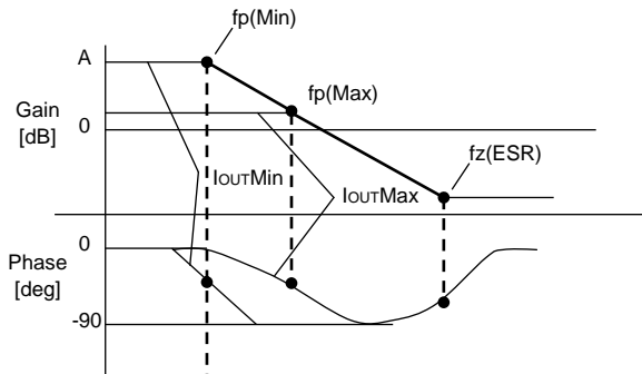
Figure 31. オープンループゲイン特性
