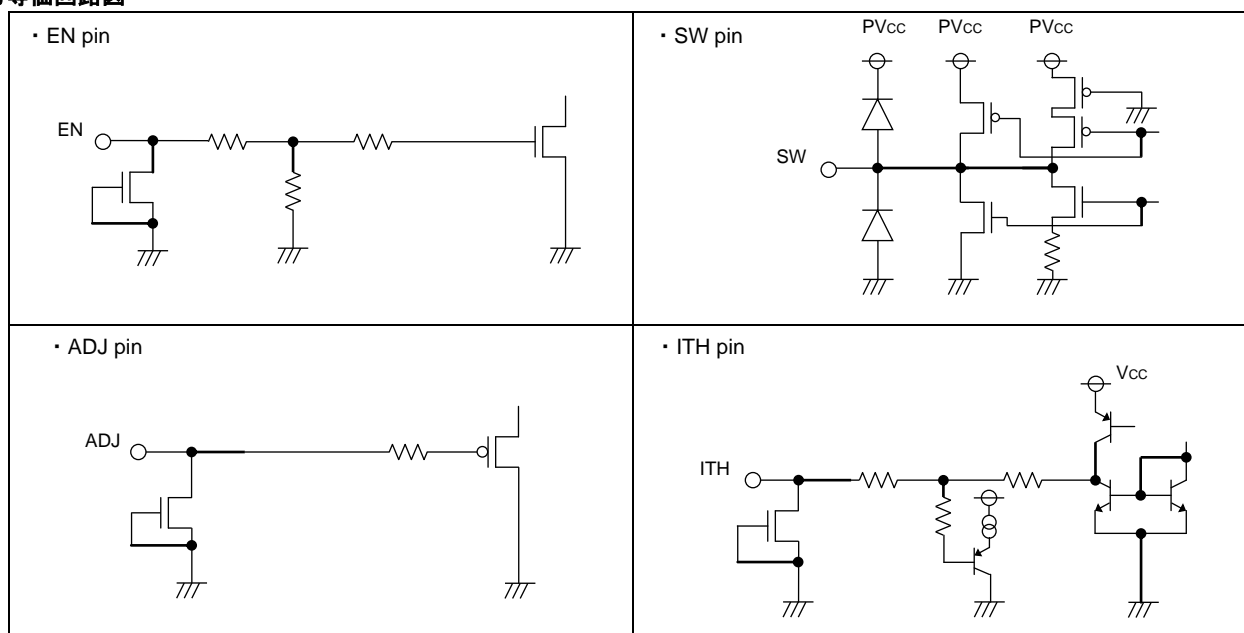
Figure 37. I/O 入出力等価回路図
