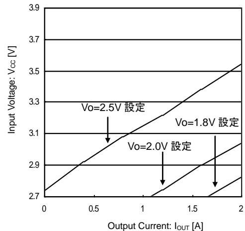
Figure 35. 各出力電圧における必要最低入力電圧
