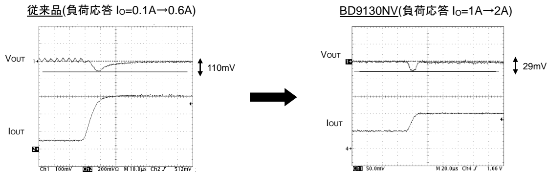
負荷急変による出力電圧ドロップが大幅に減少 Figure 24. 過渡応答比較
