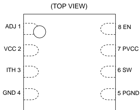
Figure 2. 端子配置図
