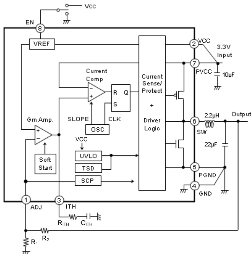
Figure 3. ブロック図
