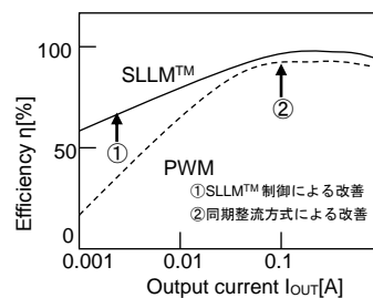
Figure 25. 効率特性
