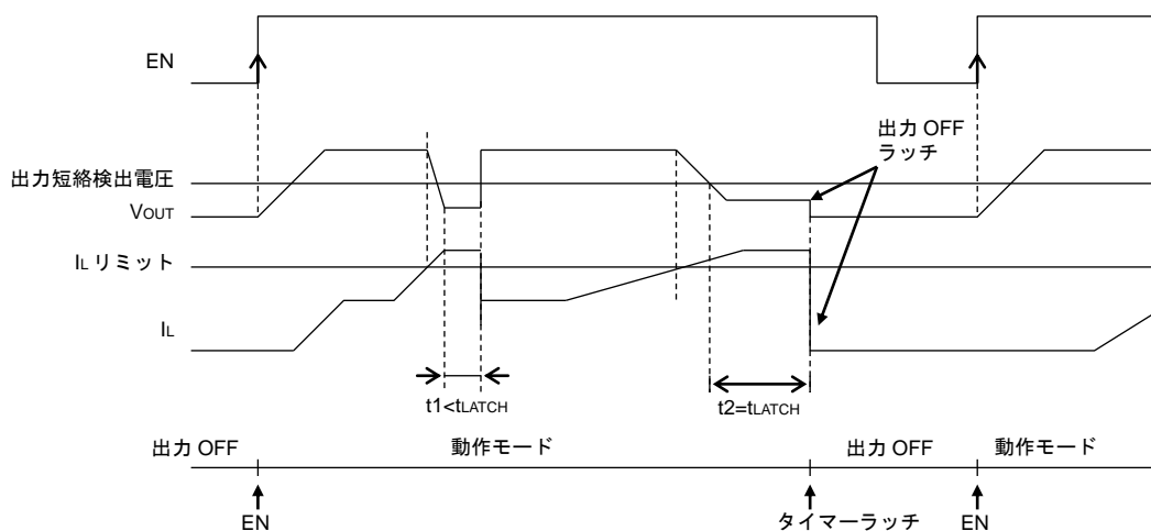
Figure 23. タイマーラッチ式ショート保護タイミングチャート
