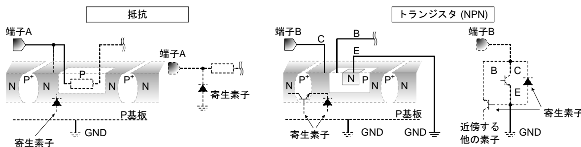
Figure 38. モノリシック IC 構造例
