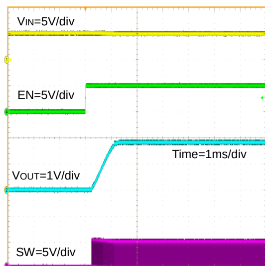
Figure 28. 起動波形 (EN = 0V → 5V)
