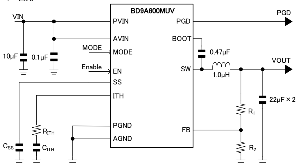
Figure 1. アプリケーション回路
