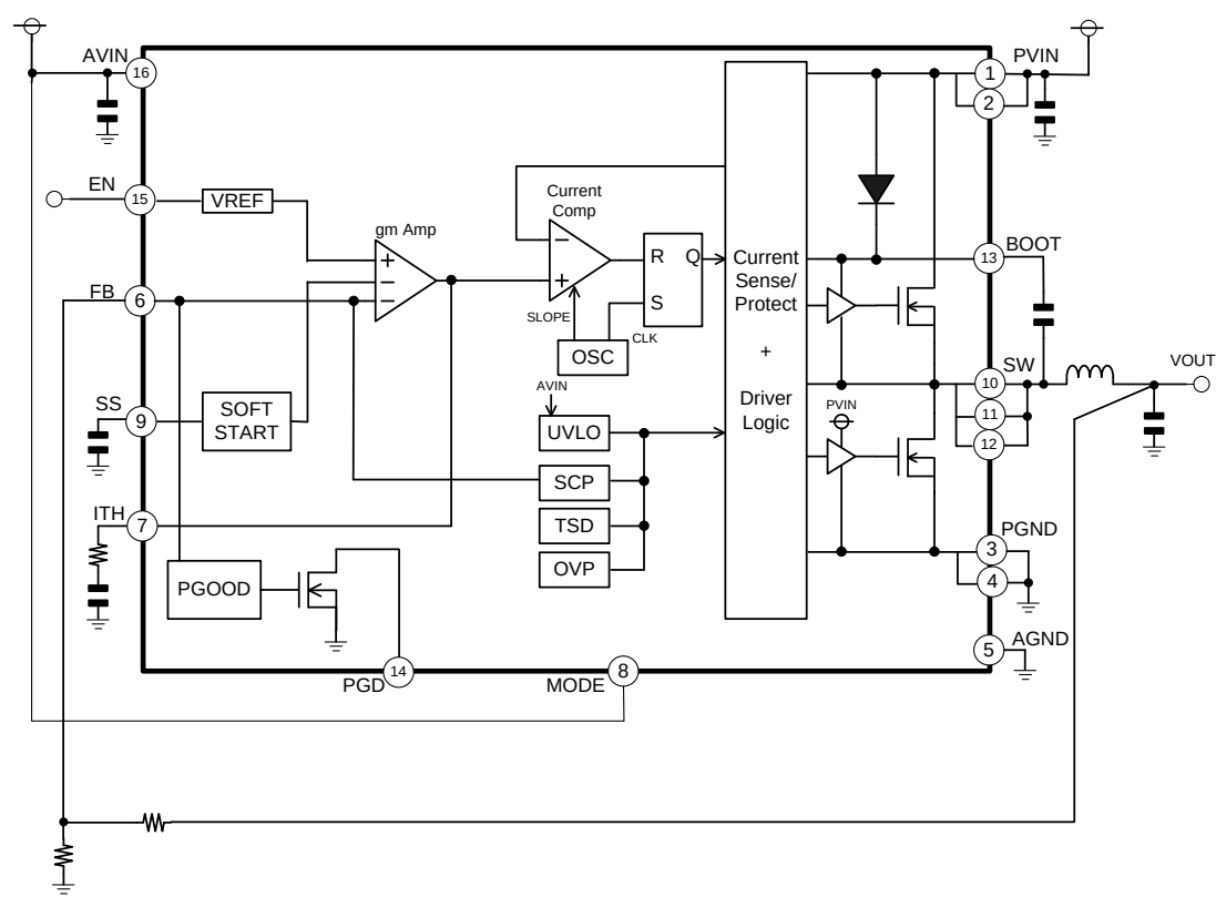
Figure 3. ブロック図
