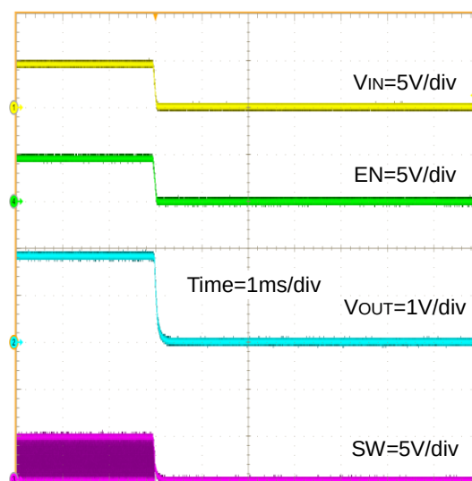
Figure 27. シャットダウン波形 (VIN = EN)
