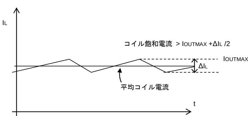
Figure 49. インダクタに流れる電流波形
