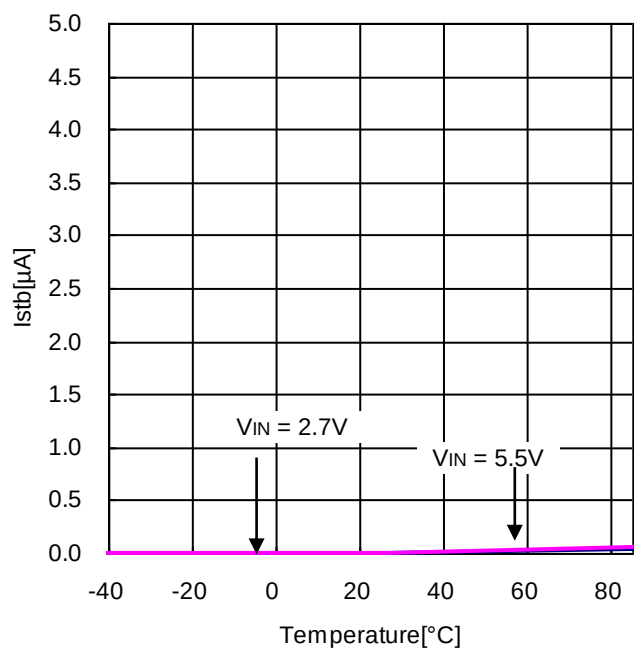
Figure 5. スタンバイ時回路電流 vs 温度
