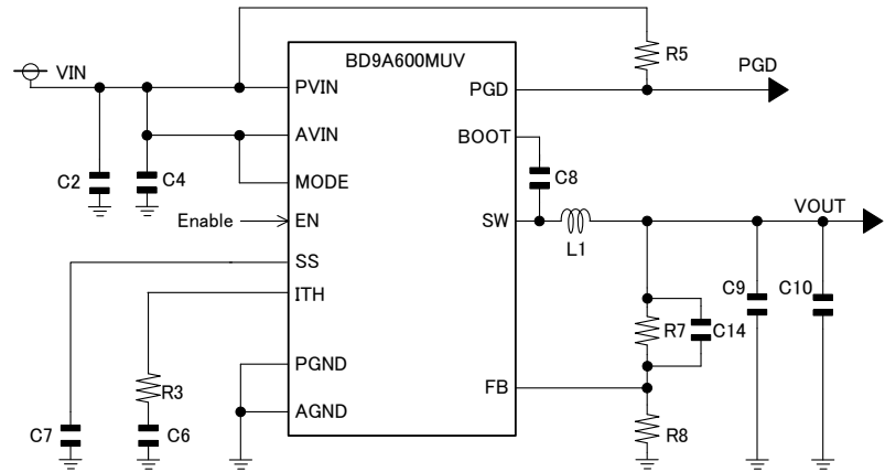
Figure 48. アプリケーション回路 Table 1. 推奨部品値( V_{IN} = 5V )
