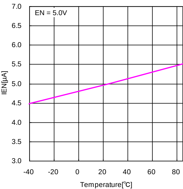
Figure 21. EN 流入電流 vs 温度
