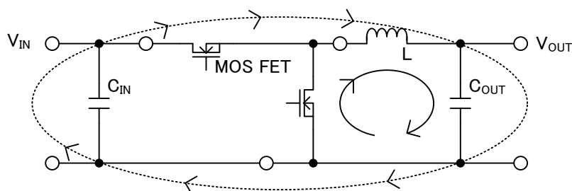
Figure 54. 降圧コンバータの電流ループ
