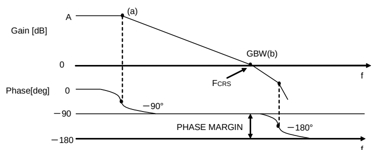
Figure 53. ボード線図
