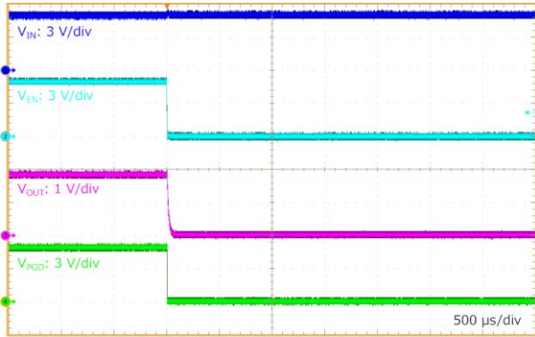
Figure 59. R_{Load} = 0.6\ \Omega EN シャットダウン波形 ( V_{IN} = 5.0\text{ V} , V_{OUT} = 1.8\text{ V} , V_{EN} = 5\text{ V to }0\text{ V} )
