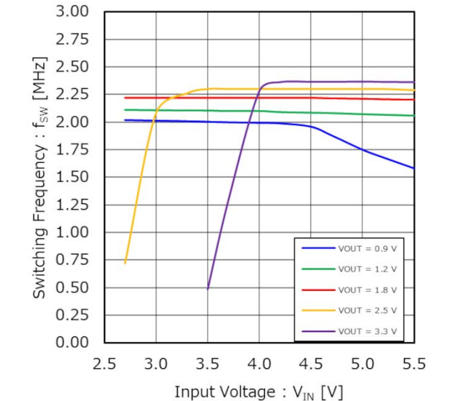
Figure 45. スイッチング周波数 vs 入力電圧 ( I_{OUT} = 1.0\text{ A} )
