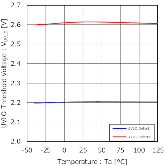
Figure 3. UVLO スレッショルド電圧 vs 温度
