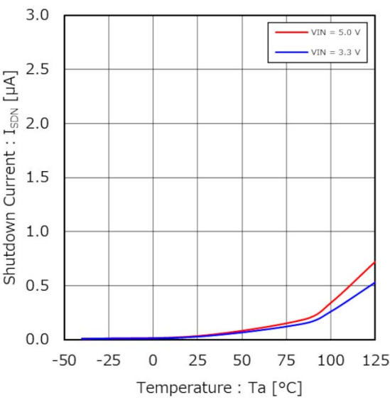
Figure 1. シャットダウン電流 vs 温度
