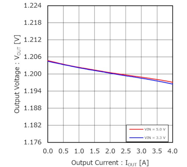
Figure 36. 出力電圧 vs 出力電流（ロードレギュレーション） ( V_{OUT} = 1.2\text{ V} )
