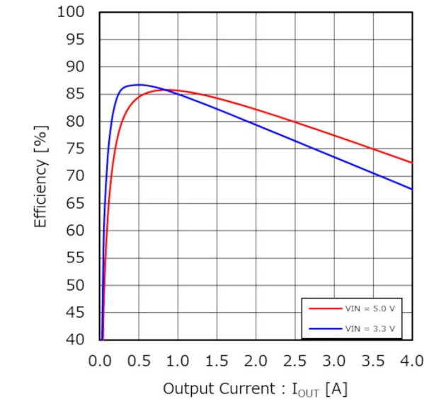
Figure 28. 効率 vs 出力電流 (VOUT = 0.6 V)
