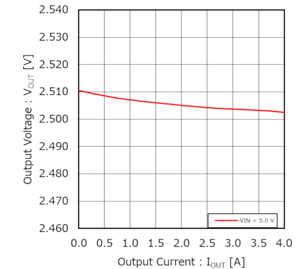
Figure 38. 出力電圧 vs 出力電流（ロードレギュレーション） ( V_{OUT} = 2.5\text{ V} )
