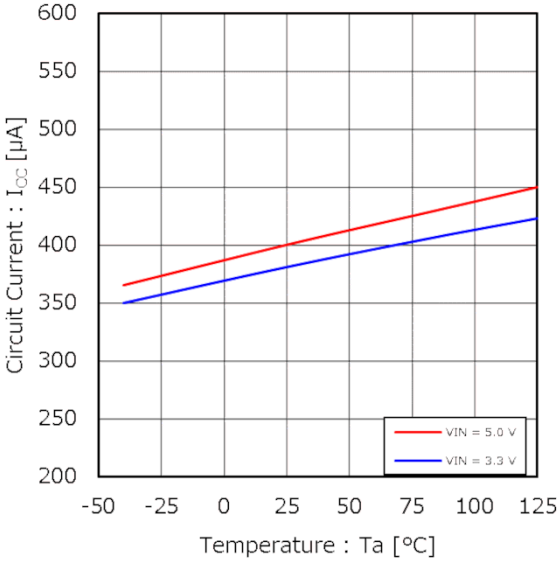
Figure 2. 回路電流 vs 温度
