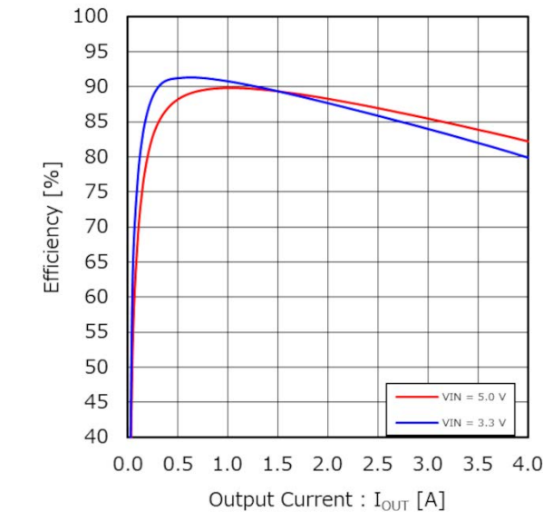
Figure 30. 効率 vs 出力電流 (VOUT = 1.2 V)
