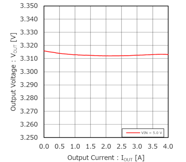
Figure 39. 出力電圧 vs 出力電流（ロードレギュレーション） ( V_{OUT} = 3.3\text{ V} )
