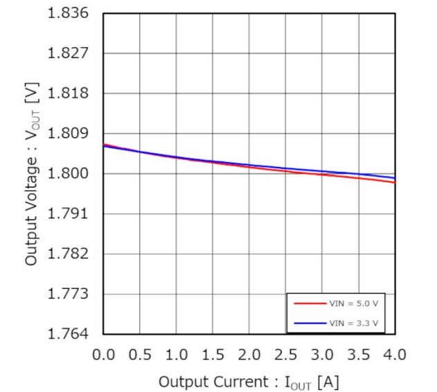
Figure 37. 出力電圧 vs 出力電流（ロードレギュレーション） ( V_{OUT} = 1.8\text{ V} )
