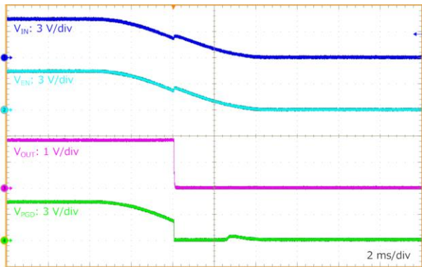
Figure 63. R_{Load} = 0.45\text{ }\Omega VIN シャットダウン波形 ( V_{IN} = V_{EN} = 5\text{ V} to 0\text{ V} , V_{OUT} = 1.8\text{ V} )
