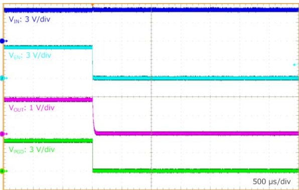
Figure 59. R_{Load} = 0.45\ \Omega EN シャットダウン波形 ( V_{IN} = 5.0\text{ V} , V_{OUT} = 1.8\text{ V} , V_{EN} = 5\text{ V to } 0\text{ V} )
