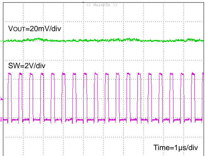
Figure 33. スイッチング波形 (VIN=5V, VOUT=1.2V, FREQ=L, IOUT=6A)
