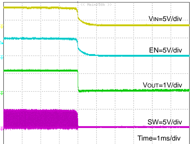
Figure 31. VIN シャットダウン波形 (FREQ=H, RLOAD=0.2Ω)
