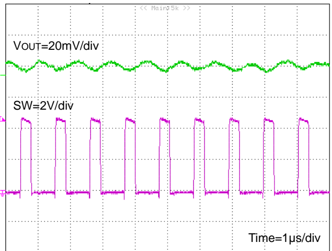
Figure 35. スイッチング波形 (VIN=5V, VOUT=1.2V, FREQ=H, IOUT=6A)
