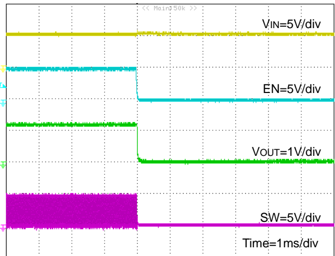
Figure 29. EN シャットダウン波形 (FREQ=H, RLOAD=0.2Ω)
