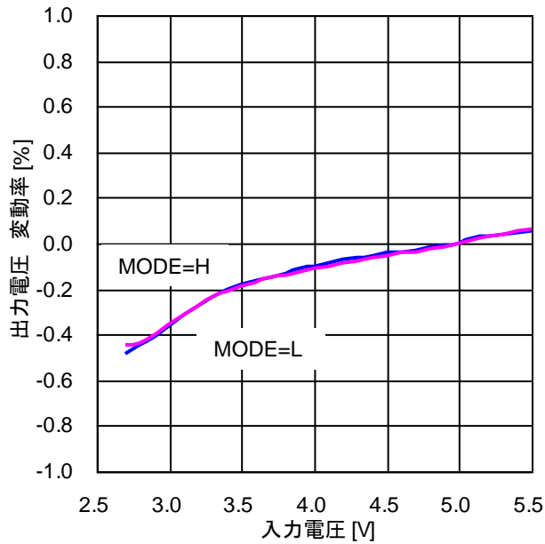
Figure 36. ラインレギュレーション ( V_{OUT}=1.2V , L=1.0\mu H , FREQ=H , I_{OUT}=6A )
