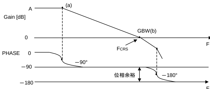
Figure 27. ボード線図
