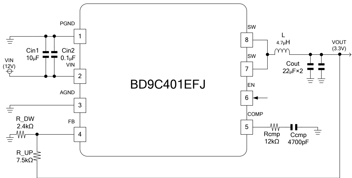
Figure 20. アプリケーション回路図 ( V_{IN}=12V , V_{OUT}=3.3V )
