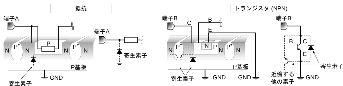
Figure 29. モノリシック IC 構造例
