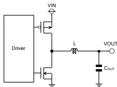
Figure 24. 出力 LC フィルタ回路
