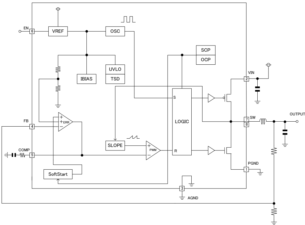
Figure 3. ブロック図
