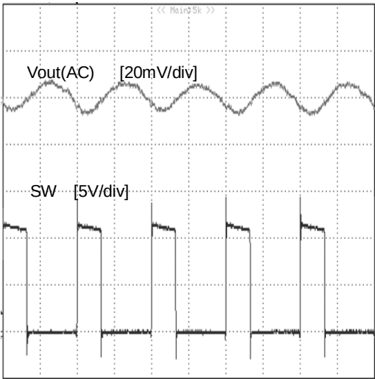
Figure 7. 出力リップル電圧 (VIN=12V, Vout=3.3V, L=4.7μH, Cout=44μF, Iout=4A)
