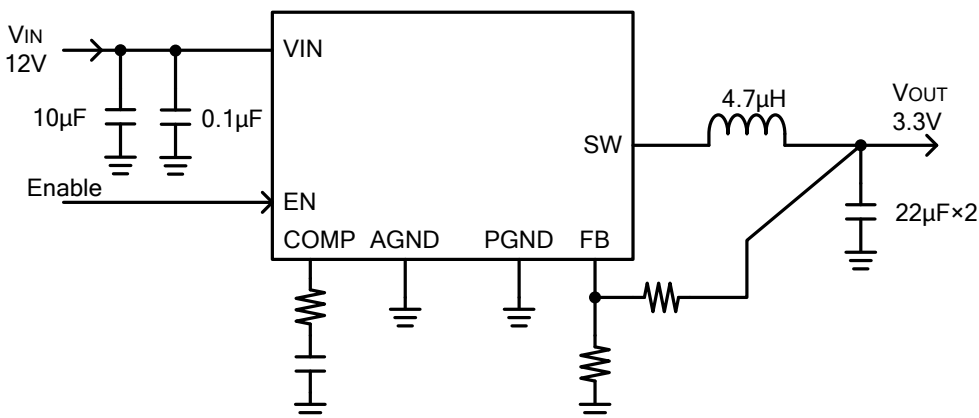
Figure 1. アプリケーション回路例
