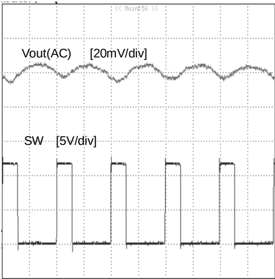
Figure 6. 出力リップル電圧 (VIN=12V, Vout=3.3V, L=4.7μH, Cout=44μF, Iout=0A)
