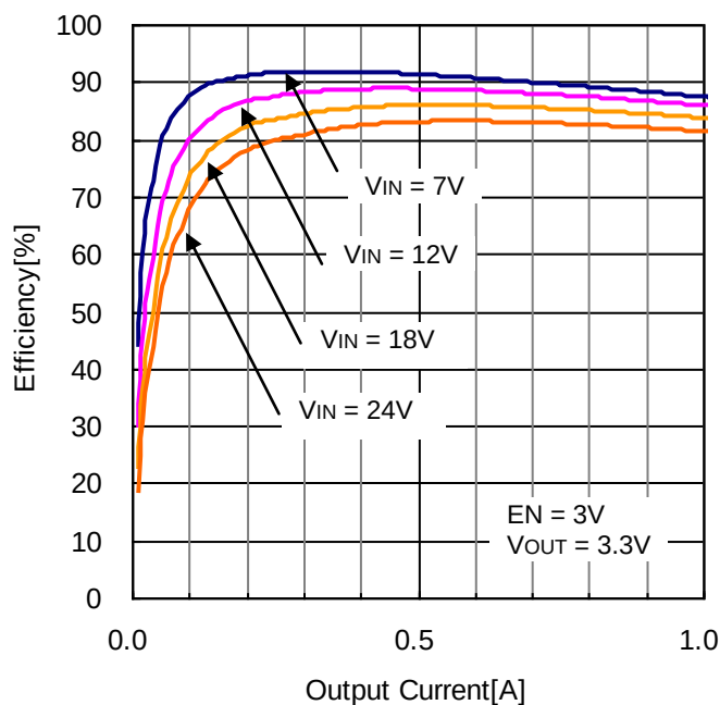
Figure 18. 効率 vs 出力負荷電流 ( V_{OUT} = 3.3V , L = 10\mu H )
