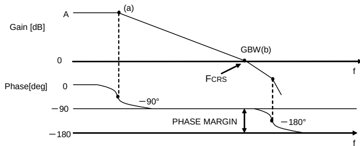
Figure 50. ボード線図
