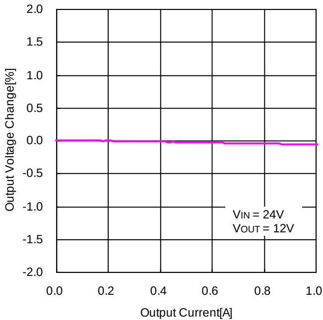
Figure 36. V OUT ロードレギュレーション
