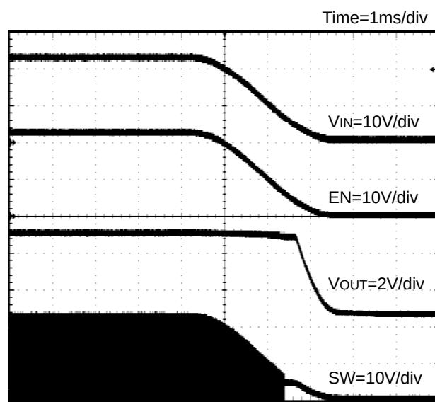
Figure 22. シャットダウン波形 ( V_{IN} = EN ) ( V_{OUT} = 5.0V )
