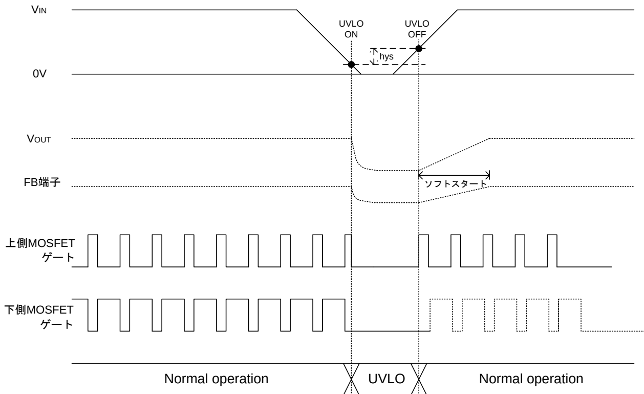
Figure 43. UVLO タイミングチャート
