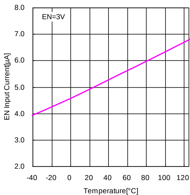
Figure 16. EN 端子流入電流 vs ジャンクション温度
