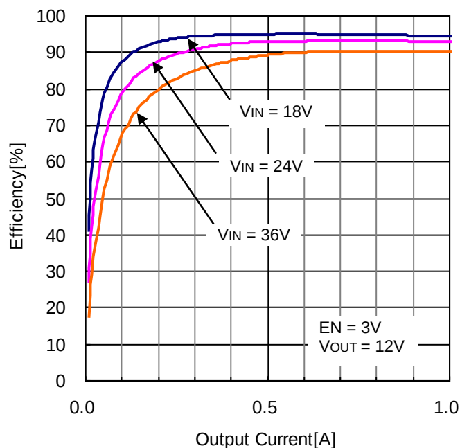
Figure 20. 効率 vs 出力負荷電流 ( V_{OUT} = 12V , L = 10\mu H )
