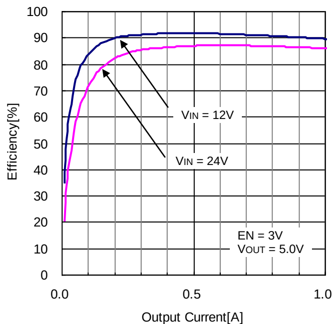
Figure 19. 効率 vs 出力負荷電流 ( V_{OUT} = 5.0V , L = 10\mu H )
