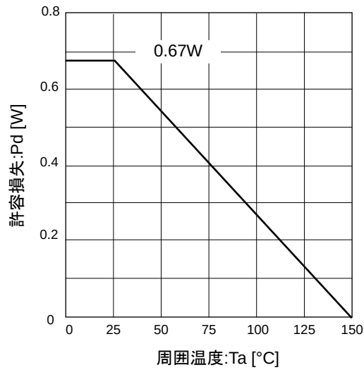
Figure 53. 熱軽減特性(SOP-J8)
