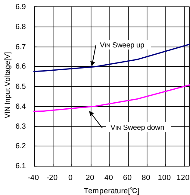
Figure 13. UVLO スレッシュホールド vs ジャンクション温度
