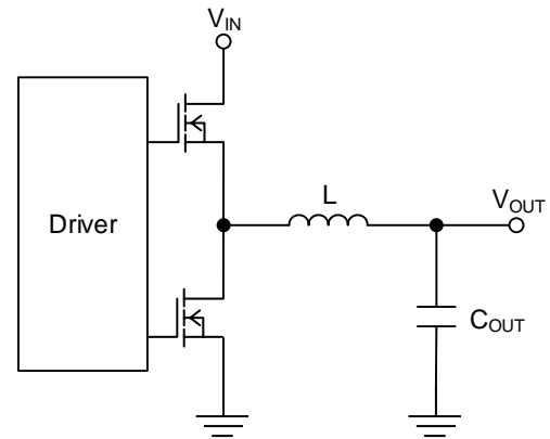
Figure 57. 出力 LC フィルタ回路
