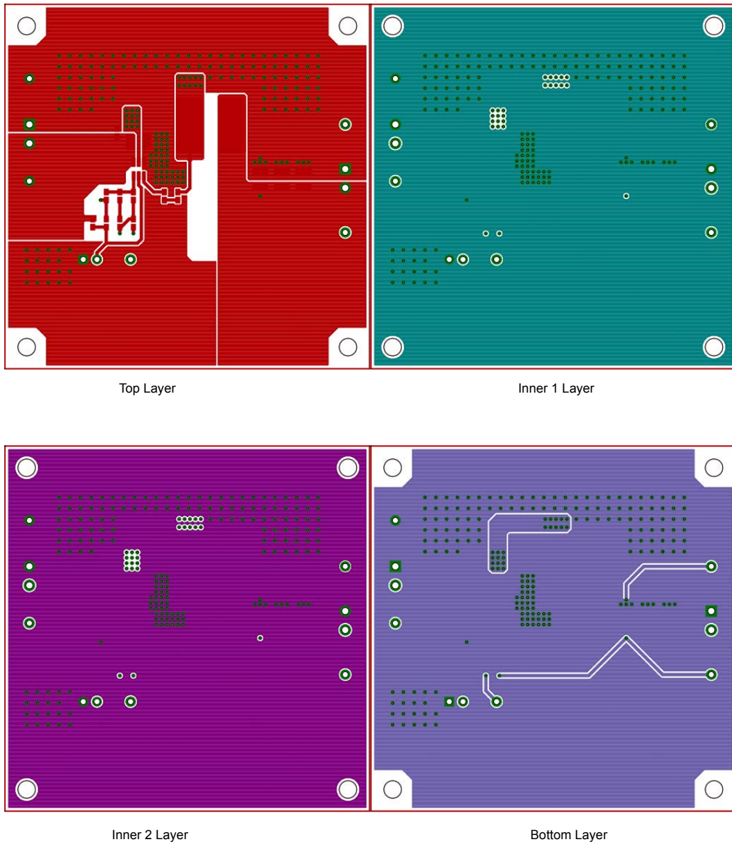
Figure 62. PCB レイアウト例
