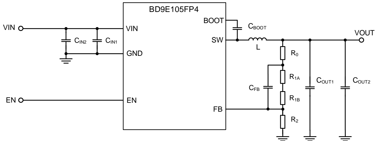
Figure 51. アプリケーション回路図
