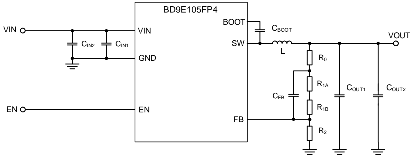
Figure 31. アプリケーション回路図
