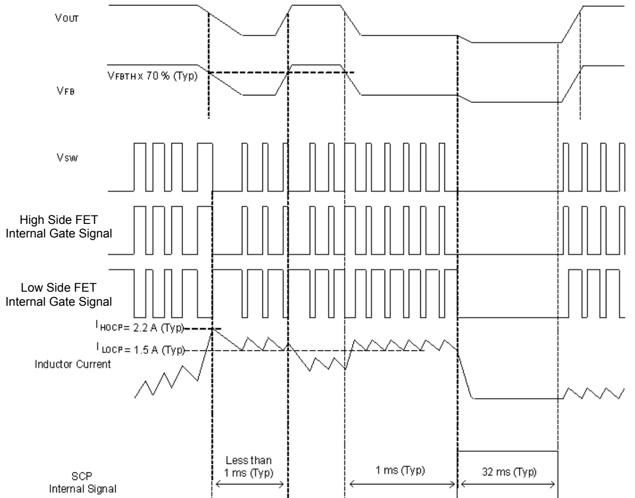
Figure 29. OCP・SCP タイミングチャート
