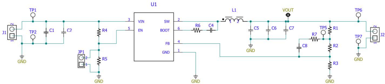
Figure 60. アプリケーション回路図
