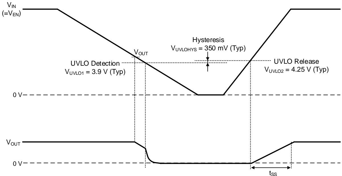
Figure 30. UVLO タイミングチャート
