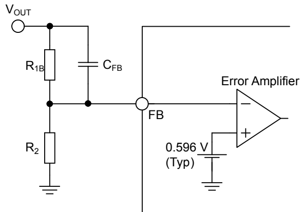
Figure 58. フィードバック抵抗回路
