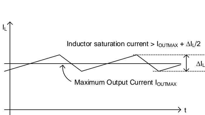
Figure 56. インダクタに流れる電流波形
