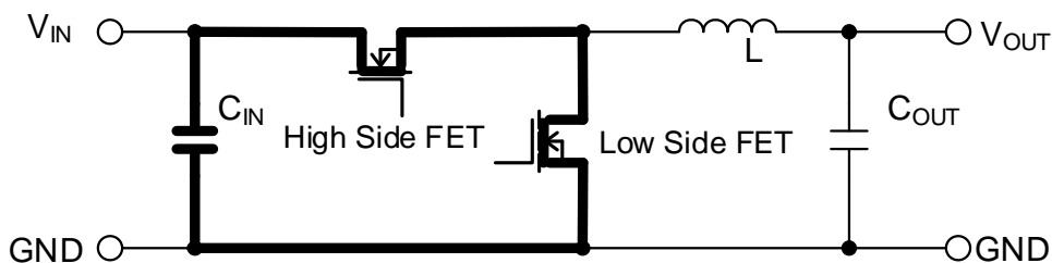
Figure 59-c. 電流の差分、レイアウト上での重要箇所
