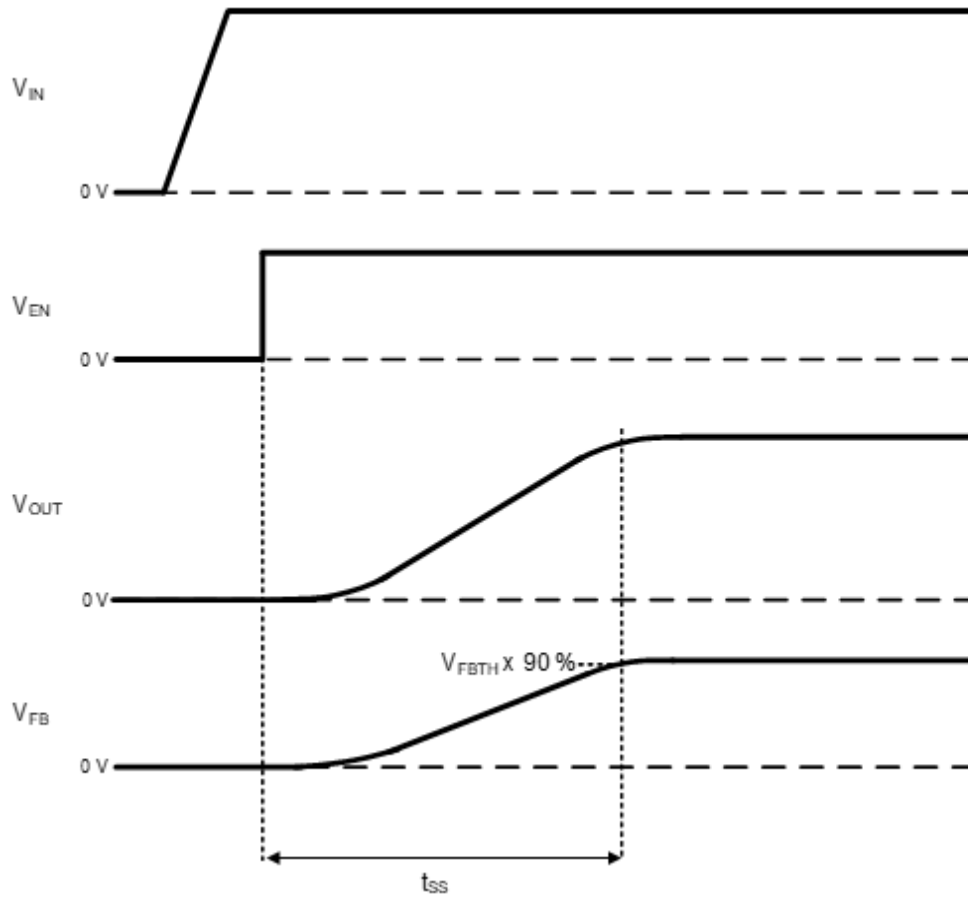
Figure 28. ソフトスタート タイミングチャート
