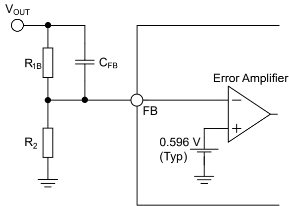
Figure 53. フィードバック抵抗回路
