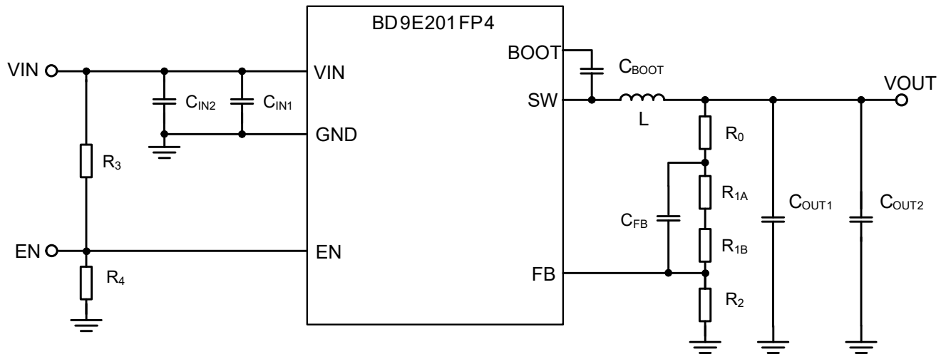
Figure 36. アプリケーション回路図
