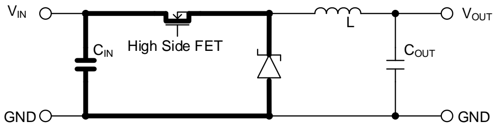
Figure 61-c. 電流の差分、レイアウト上での重要箇所
