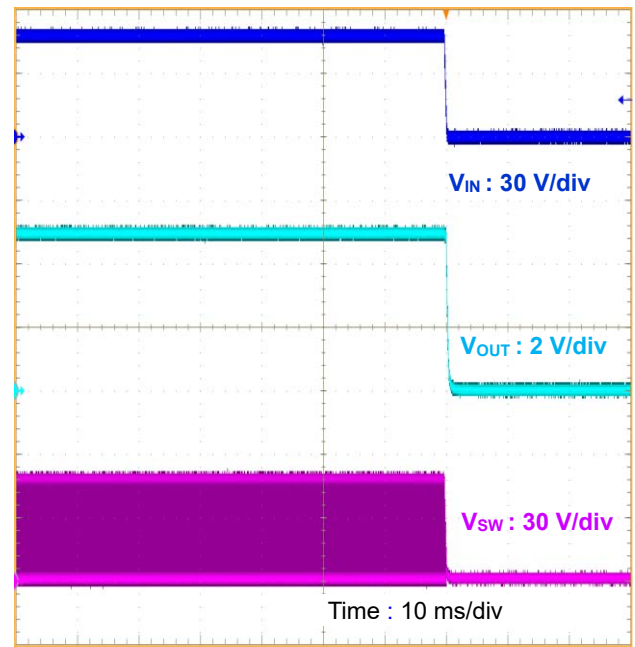
Figure 20. シャットダウン波形 ( V_{IN} = V_{EN} , V_{IN} = 48\text{ V} , V_{OUT} = 5\text{ V} , f_{OSC} = 200\text{ kHz} , I_{OUT} = 5\text{ A} )
