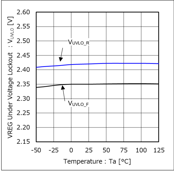
Figure 4. VREG UVLO 電圧 vs 温度
