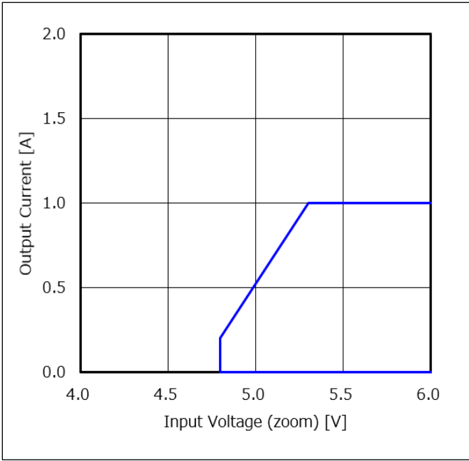
Figure 54. 出力電流 vs 入力電圧 (Note 1) 動作範囲: Tj < 150 °C
