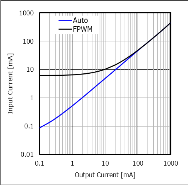
Figure 76. 入力電流 vs 出力負荷電流 (VIN = 12 V)
