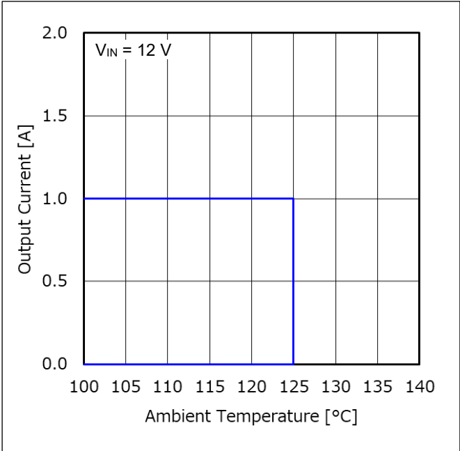
Figure 73. 出力電流 vs 周囲温度 (Note 1) 動作範囲: Tj < 150 °C
