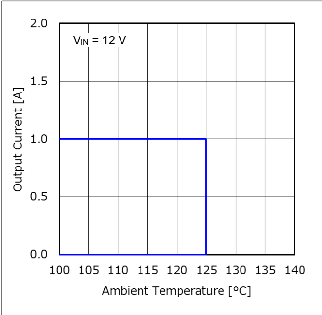
Figure 56. 出力電流 vs 周囲温度 (Note 1) 動作範囲: Tj < 150 °C
