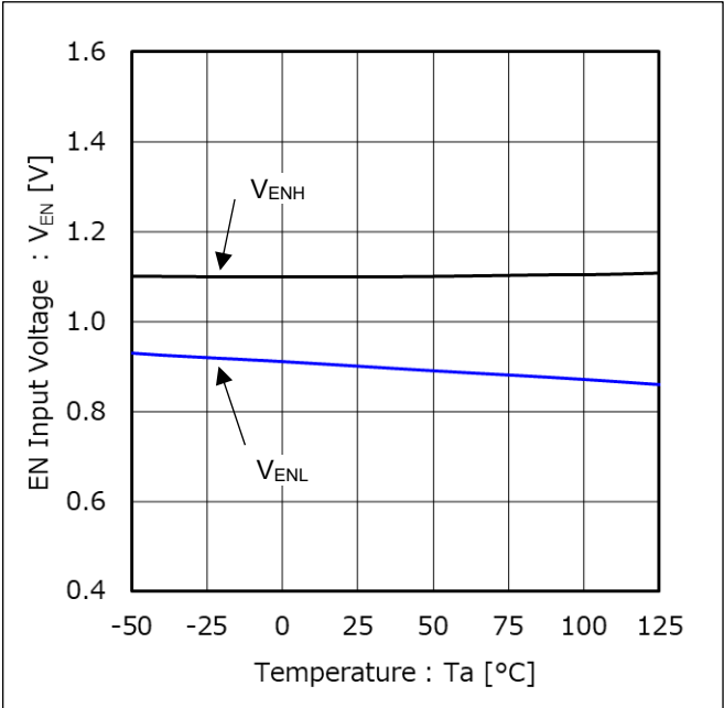
Figure 5. EN 入力電圧 vs 温度
