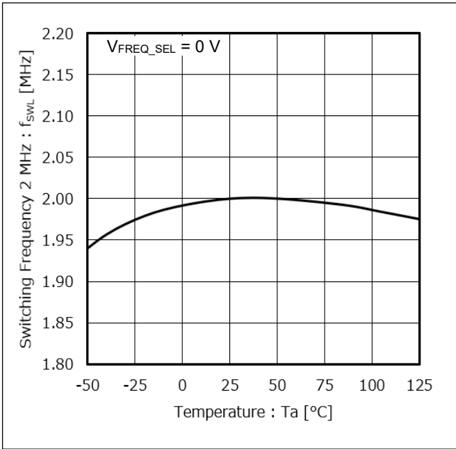
Figure 12. スイッチング周波数(f SWL ) vs 温度
