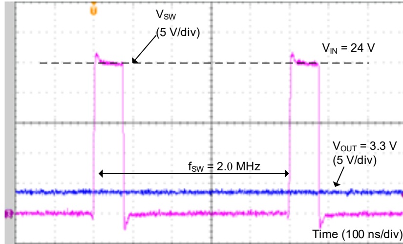
Figure 24. スイッチング波形 ( V_{IN} = 24 V、 V_{OUT} = 3.3 V、 I_{OUT} = 1.0 A、 f_{SW} = 2.0 MHz)
