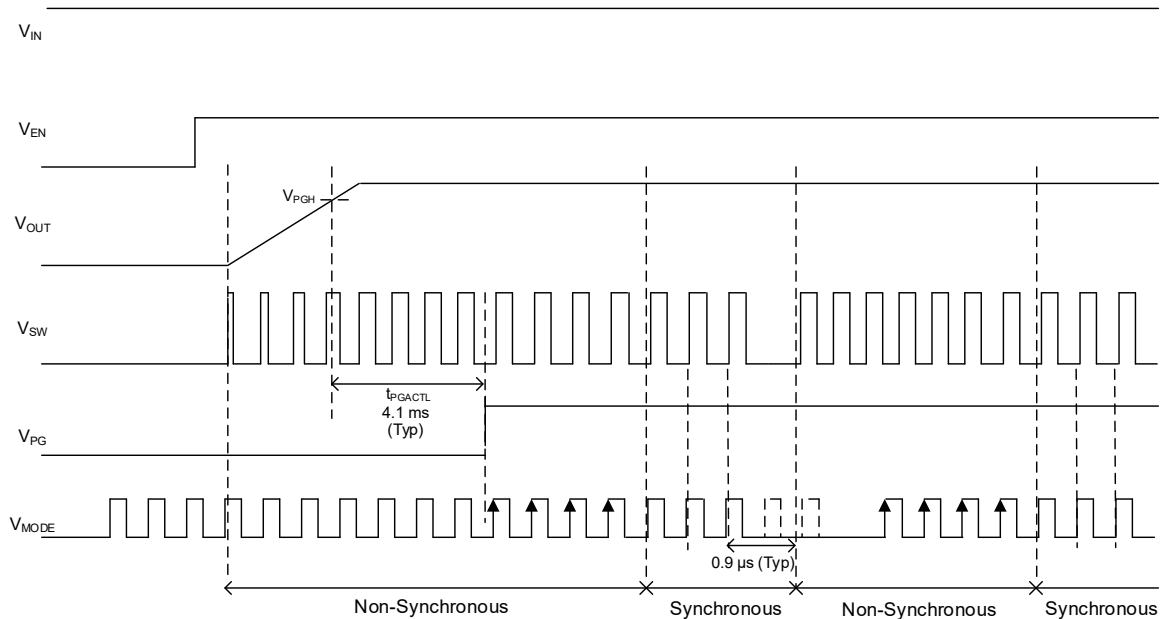
Figure 29. 外部同期機能（FREQ_SEL = L）
