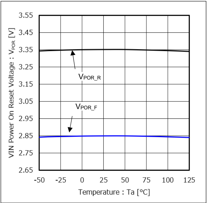
Figure 3. VIN POR 電圧 vs 温度
