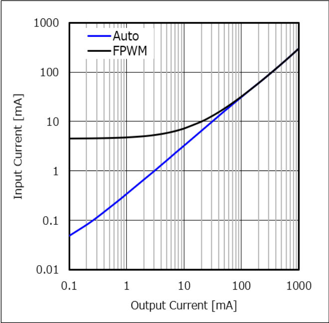
Figure 89. 入力電流 vs 出力負荷電流 (VIN = 12 V)
