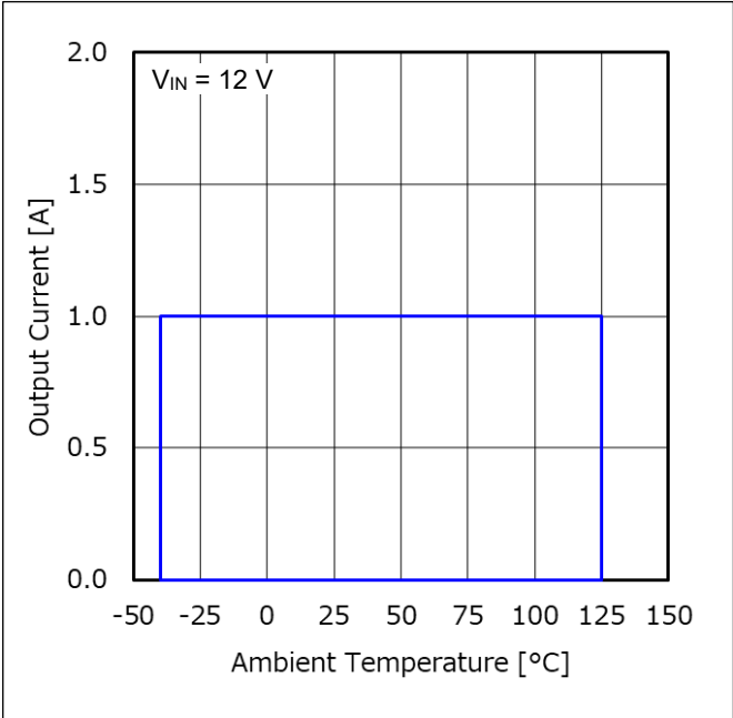
Figure 72. 出力電流 vs 周囲温度 (Note 1) 動作範囲: Tj < 150 °C
