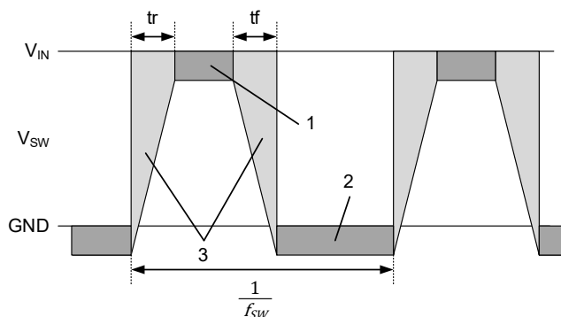
Figure 105. SW 波形
