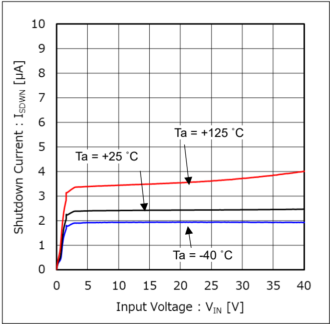
Figure 1. シャットダウン時電流 vs 入力電圧
