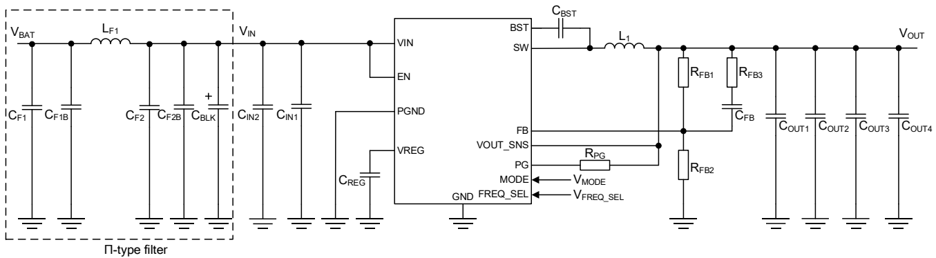
Figure 40. 参考回路
