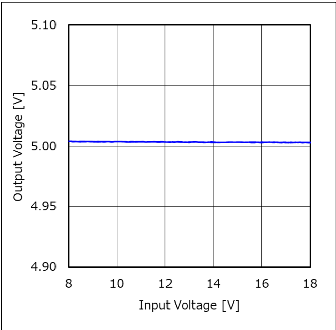
Figure 85. ラインレギュレーション (I OUT = 1 A)
