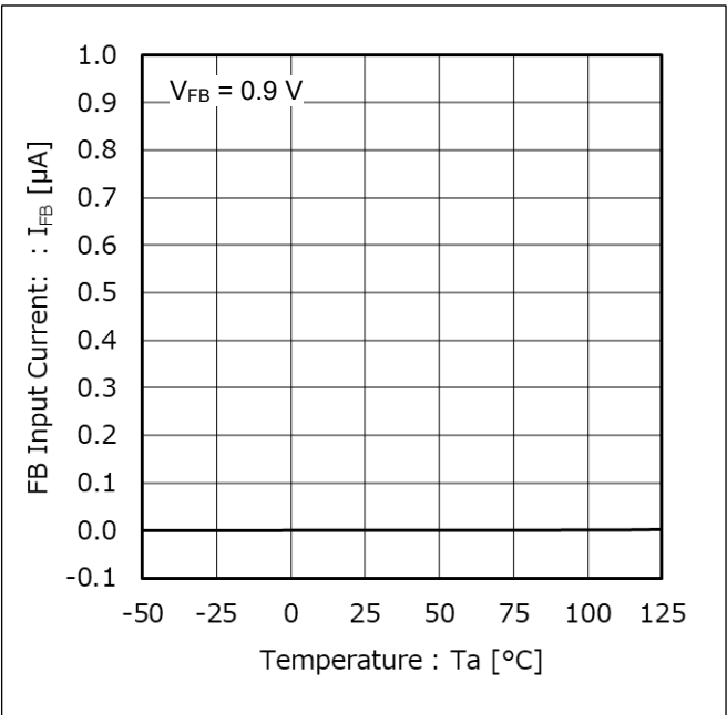
Figure 19. FB 流入電流 vs 温度
