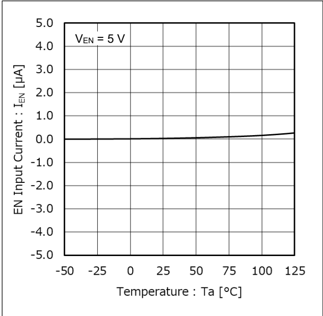
Figure 6. EN 流入電流 vs 温度
