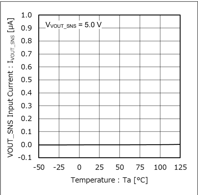
Figure 23. VOUT_SNS 流入電流 vs 温度
