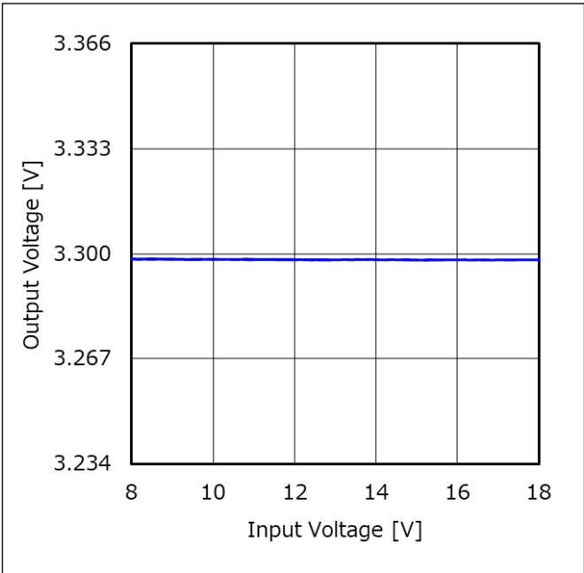
Figure 98. ラインレギュレーション (I OUT = 1 A)
