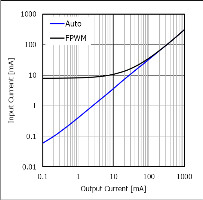
Figure 59. 入力電流 vs 出力負荷電流 (VIN = 12 V)
