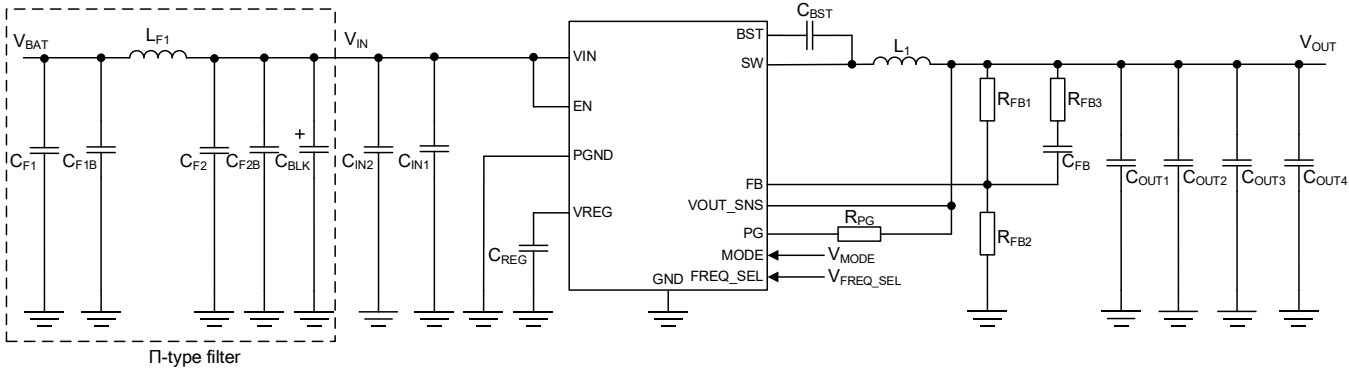
Figure 87. 参考回路
