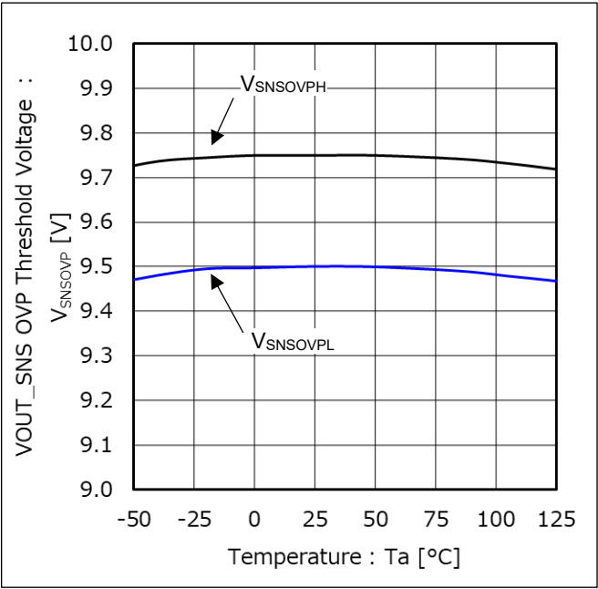
Figure 17. VOUT_SNS OVP スレッシュホールド vs 温度
