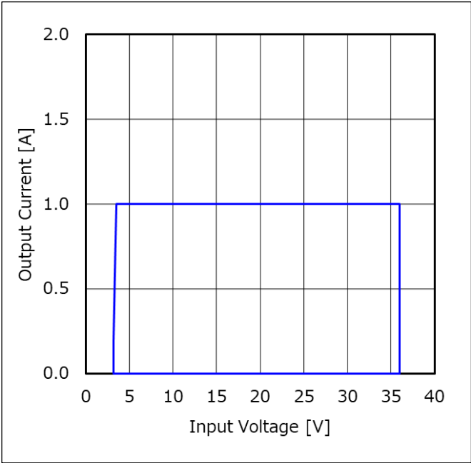
Figure 70. 出力電流 vs 入力電圧 (Note 1) 動作範囲: Tj < 150 °C
