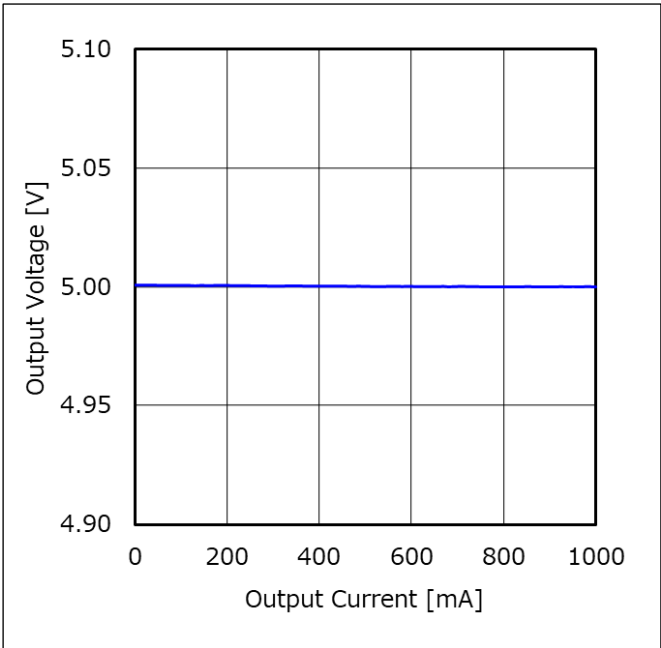
Figure 52. ロードレギュレーション (V IN = 12 V、V MODE = 3.3 V)
