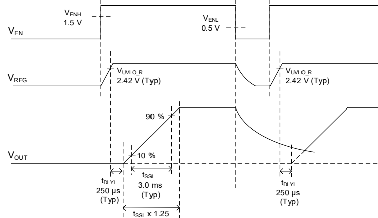
Figure 27. イネーブル ON/OFF タイミングチャート (FREQ_SEL = L)
