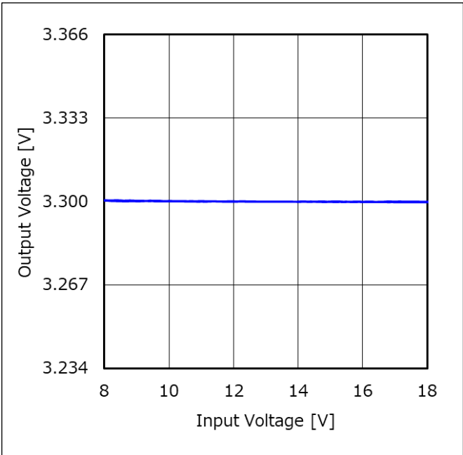
Figure 68. ラインレギュレーション (I OUT = 1 A)
