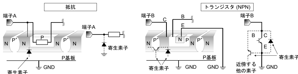
Figure 106. モノリシック IC 構造例
