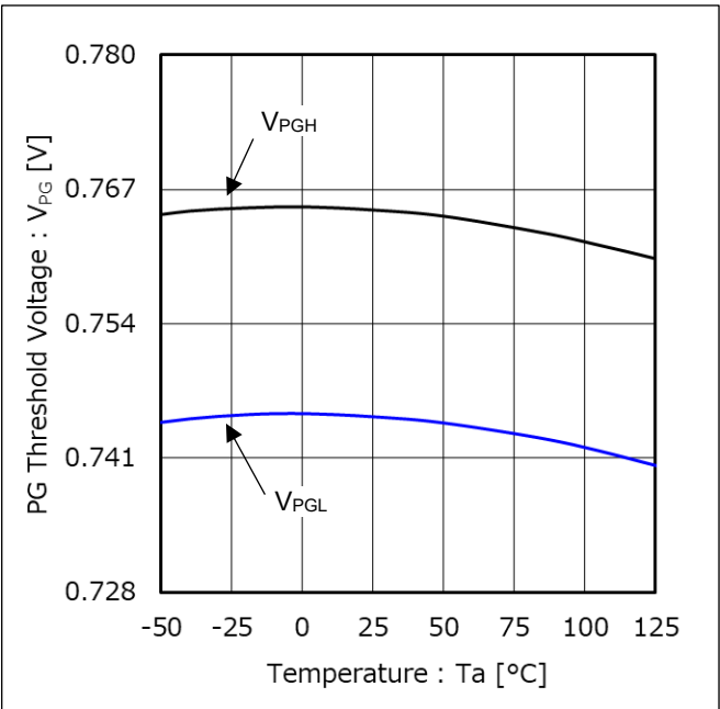
Figure 15. PG スレッシュホールド電圧 vs 温度
