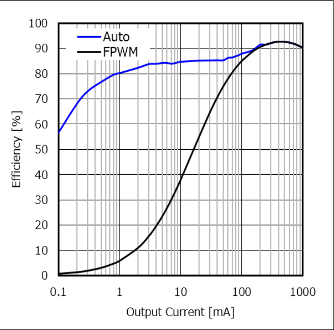
Figure 88. 効率 vs 出力負荷電流 (VIN = 12 V)
