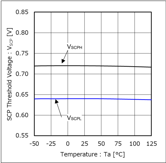
Figure 18. SCP スレッシュホールド vs 温度
