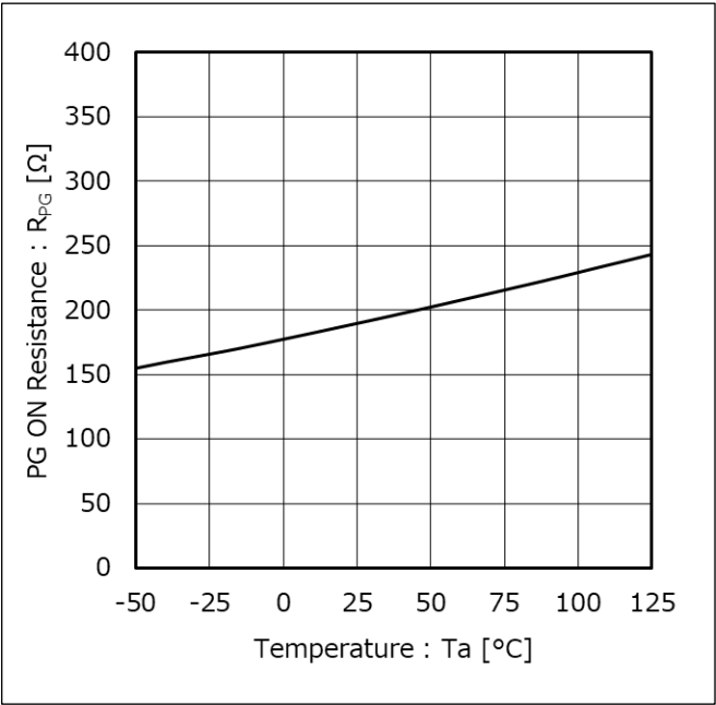
Figure 21. PG ON 抵抗 vs 温度
