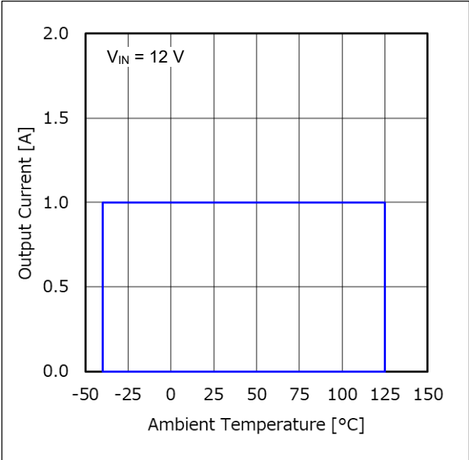
Figure 55. 出力電流 vs 周囲温度 (Note 1) 動作範囲: Tj < 150 °C
