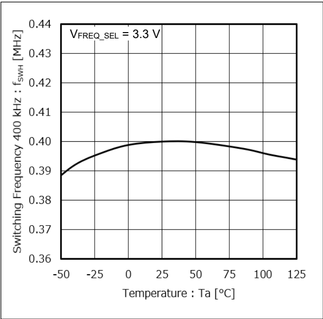
Figure 11. スイッチング周波数(f SWH ) vs 温度
