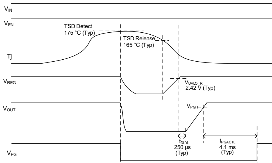
Figure 35. TSD タイミングチャート (FREQ_SEL = L)
