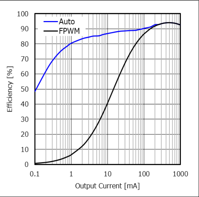
Figure 75. 効率 vs 出力負荷電流 (VIN = 12 V)
