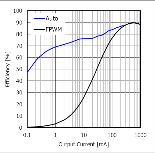
Figure 58. 効率 vs 出力負荷電流 (VIN = 12 V)
