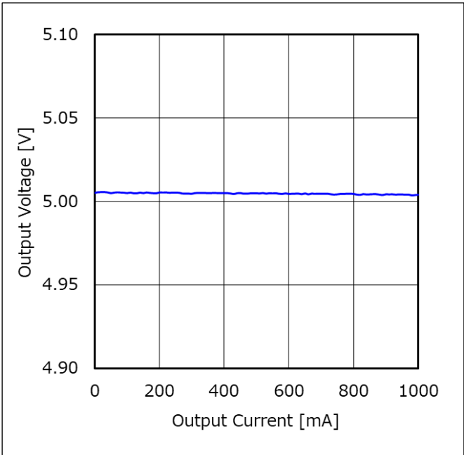
Figure 86. ロードレギュレーション (V IN = 12 V、V MODE = 3.3 V)
