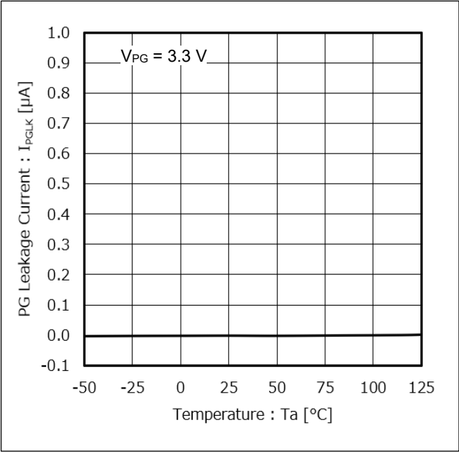
Figure 22. PG リーク電流 vs 温度
