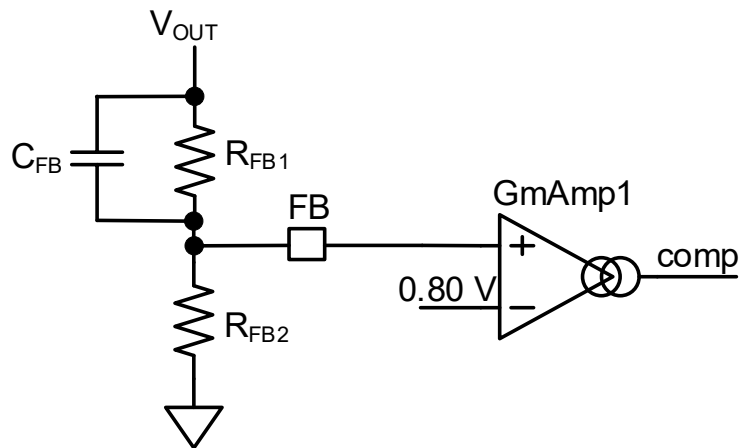
Figure 39. 出力電圧設定抵抗
