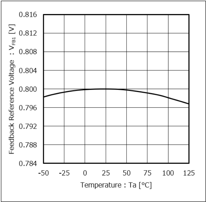
Figure 2. フィードバック電圧 vs 温度
