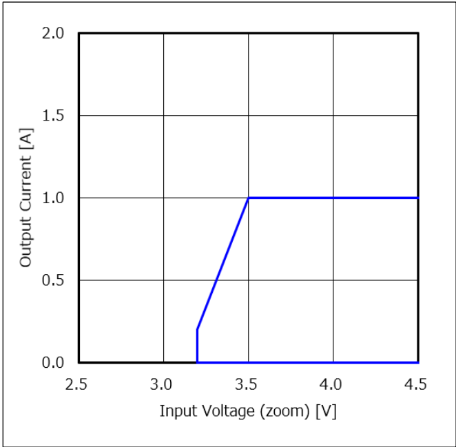
Figure 71. 出力電流 vs 入力電圧 (Note 1) 動作範囲: Tj < 150 °C
