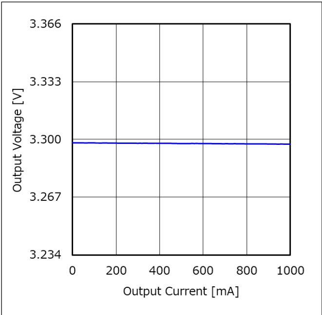
Figure 99. ロードレギュレーション (V IN = 12 V、V MODE = 3.3 V)
