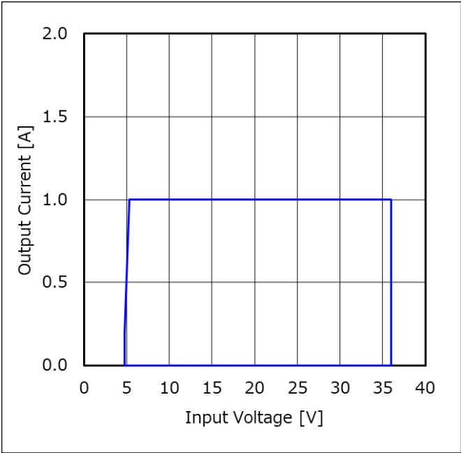
Figure 53. 出力電流 vs 入力電圧 (Note 1) 動作範囲: Tj < 150 °C
