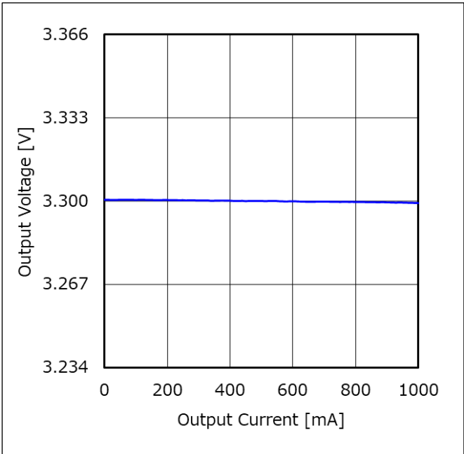
Figure 69. ロードレギュレーション (V IN = 12 V、V MODE = 3.3 V)
