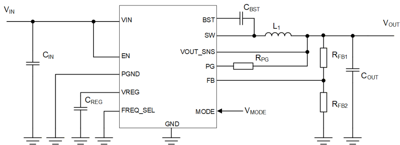
Figure 38. 参考回路
