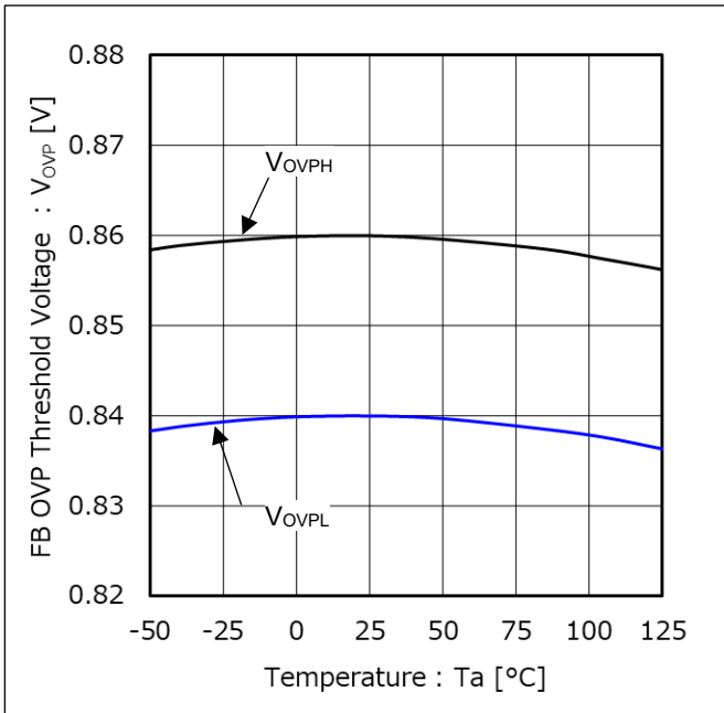
Figure 16. FB OVP スレッシュホールド電圧 vs 温度
