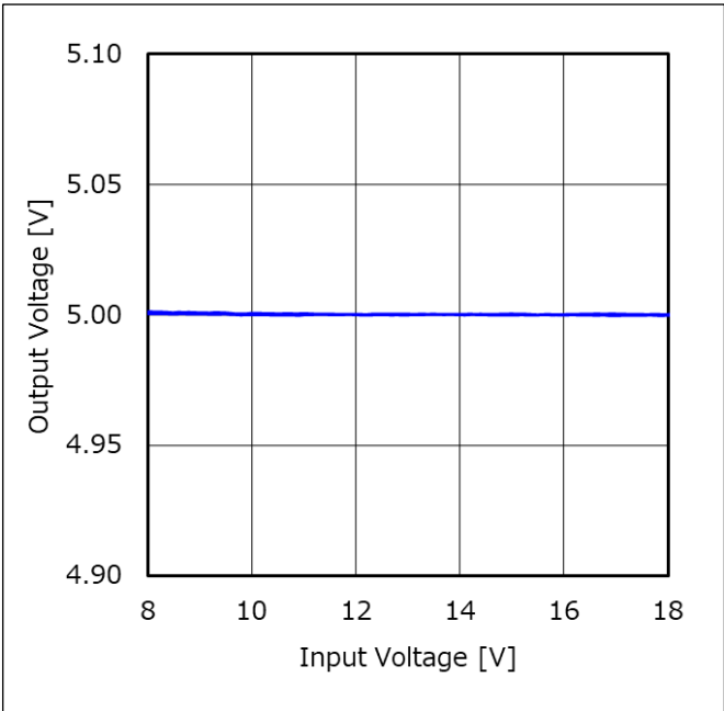
Figure 51. ラインレギュレーション (I OUT = 1 A)
