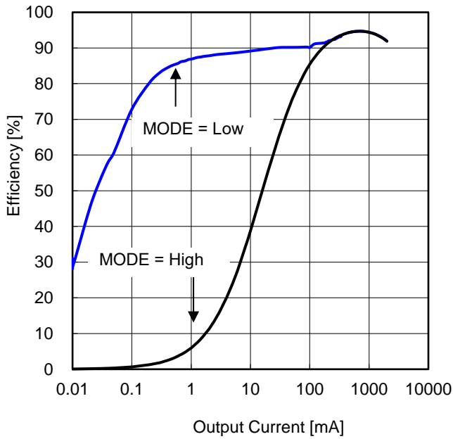
Figure 76. 効率 vs 出力負荷電流 ( V_{IN} = 12\text{ V} )
