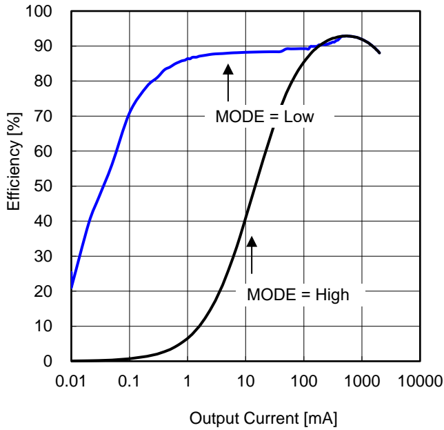
Figure 63. 効率 vs 出力負荷電流 ( V_{IN} = 12\text{ V} )
