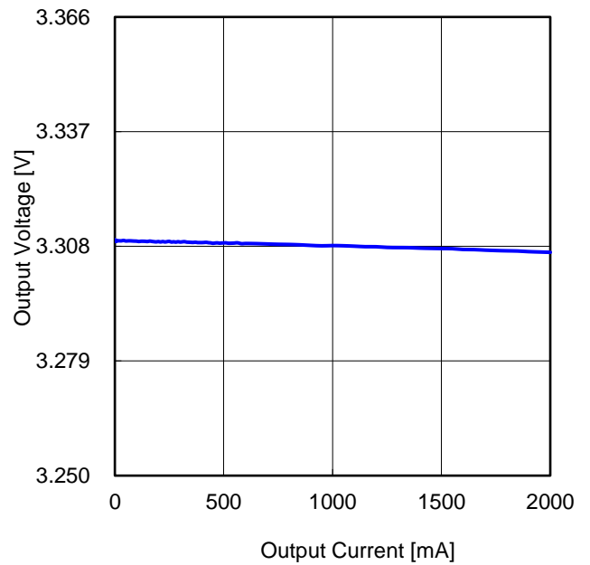
Figure 74. ロードレギュレーション (V IN = 12 V)
