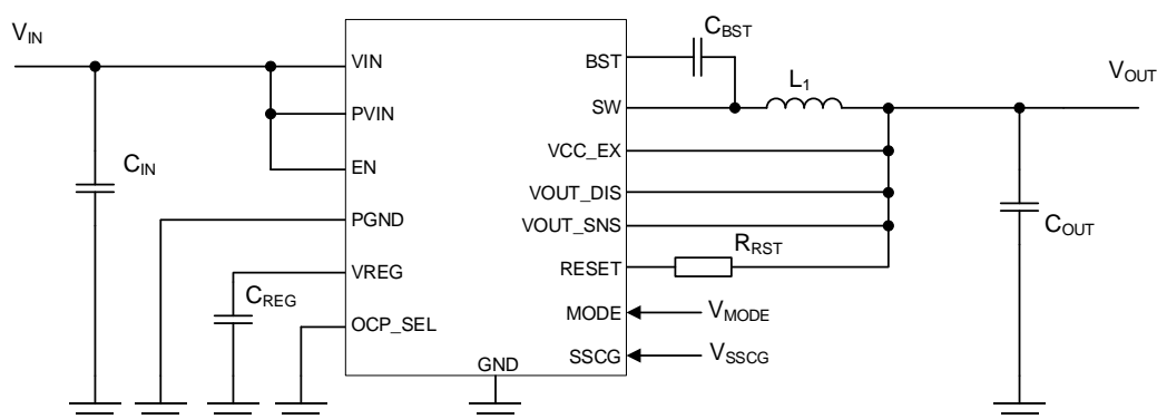
Figure 1. ディスチャージ機能を使用したアプリケーション回路 (BD9P236EFV-C, BD9P256EFV-C)
