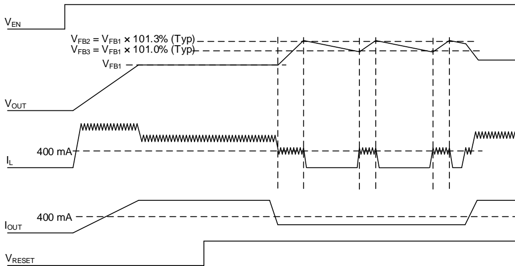
Figure 31. 軽負荷モード中タイミングチャート (OCP_SEL = L)
