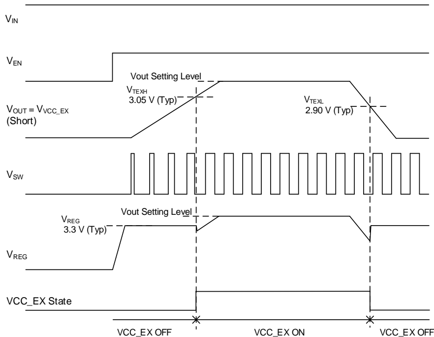
Figure 39. VCC_EX タイミングチャート
