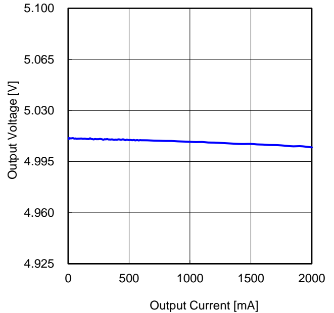
Figure 87. ロードレギュレーション (V IN = 12 V)
