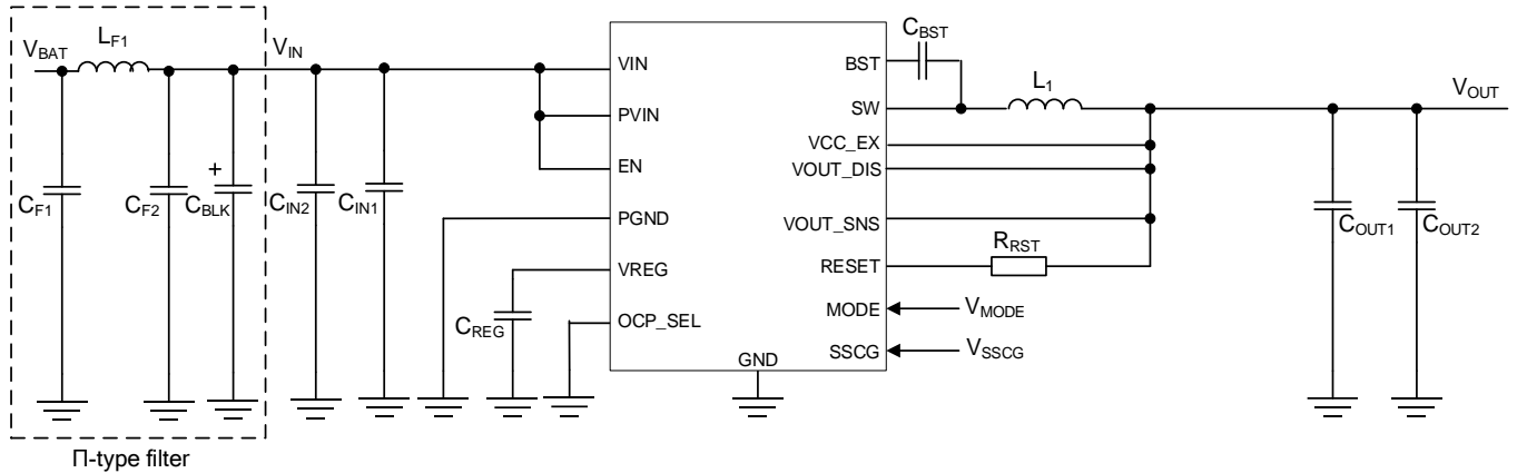
Figure 62. 参考回路 2
