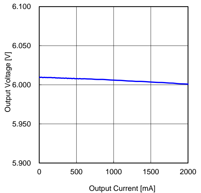
Figure 61. ロードレギュレーション (V IN = 12 V)
