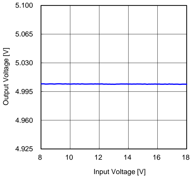
Figure 86. ラインレギュレーション (I OUT = 2 A)
