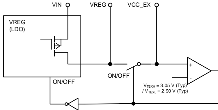
Figure 38. VCC_EX ブロック図
