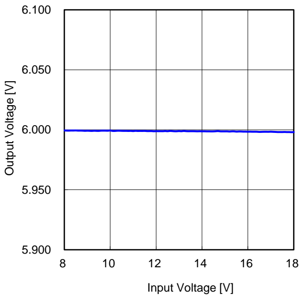
Figure 60. ラインレギュレーション (I OUT = 2 A)
