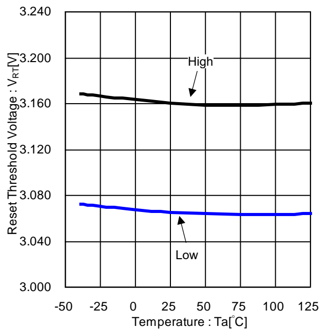
Figure 24. Reset スレッシュホールド電圧 vs 温度 (BD9P236EFV-C)
