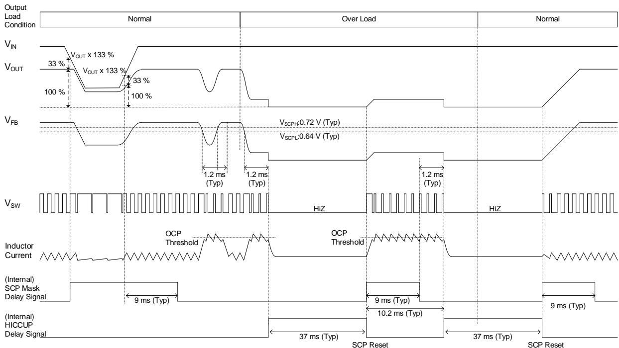
Figure 41. 短絡保護 (SCP) タイミングチャート (BD9P206EFV-C)
