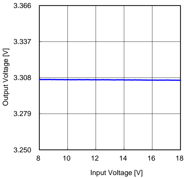
Figure 73. ラインレギュレーション (I OUT = 2 A)
