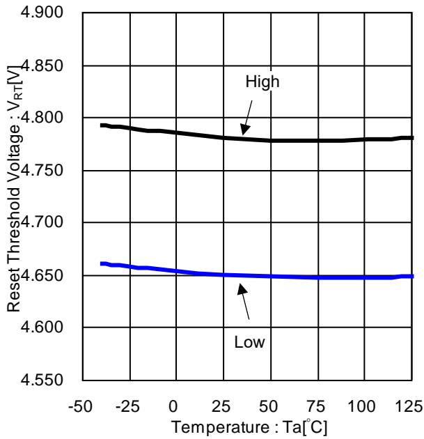
Figure 25. Reset スレッシュヨルド電圧 vs 温度 (BD9P256EFV-C)
