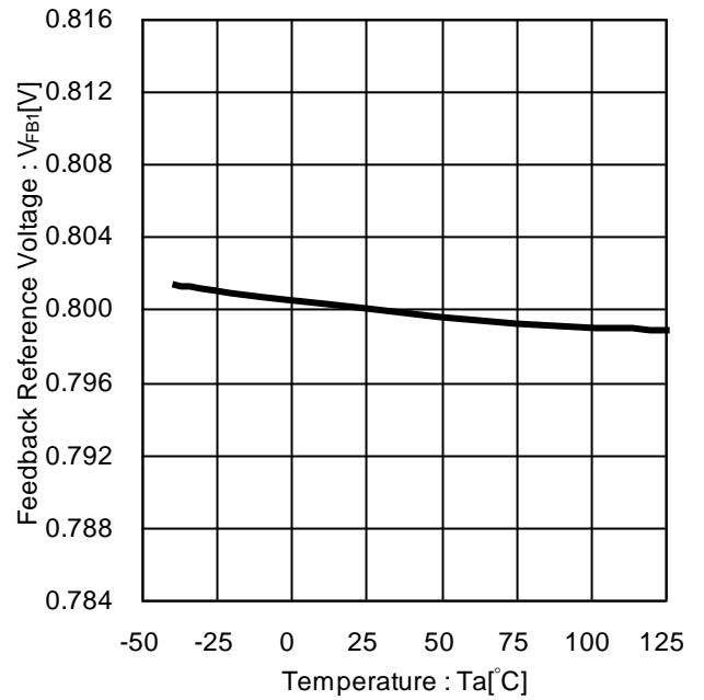
Figure 10. フィードバック電圧 vs 温度 (BD9P206EFV-C)
