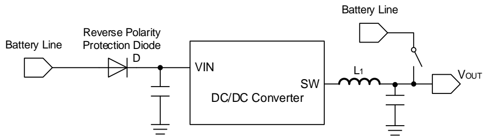
Figure 46. VOUT とバッテリーラインの短絡
