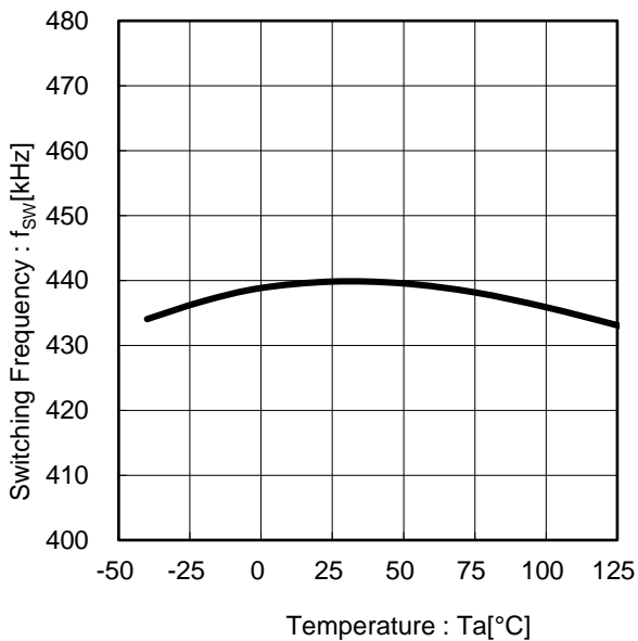
Figure 19. スイッチング周波数 vs 温度
