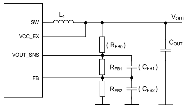
Figure 91. フィードバックの周波数特性測定用抵抗
