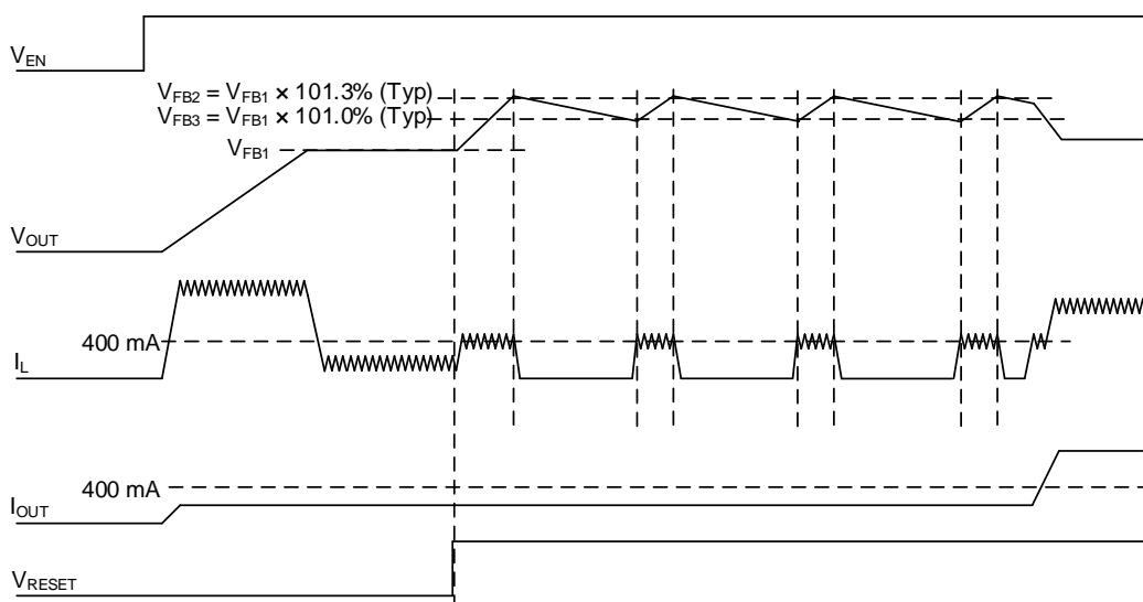
Figure 32. RESET の High 検出後の軽負荷モード中タイミングチャート (OCP_SEL = L)
