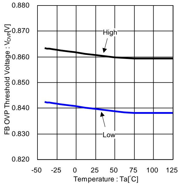
Figure 26. FB OVP スレッシュヨルド電圧 vs 温度 (BD9P206EFV-C)
