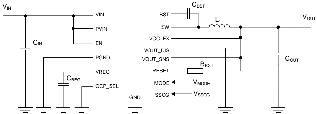
Figure 2. ディスチャージ機能を使用しないアプリケーション回路 (BD9P236EFV-C, BD9P256EFV-C)
