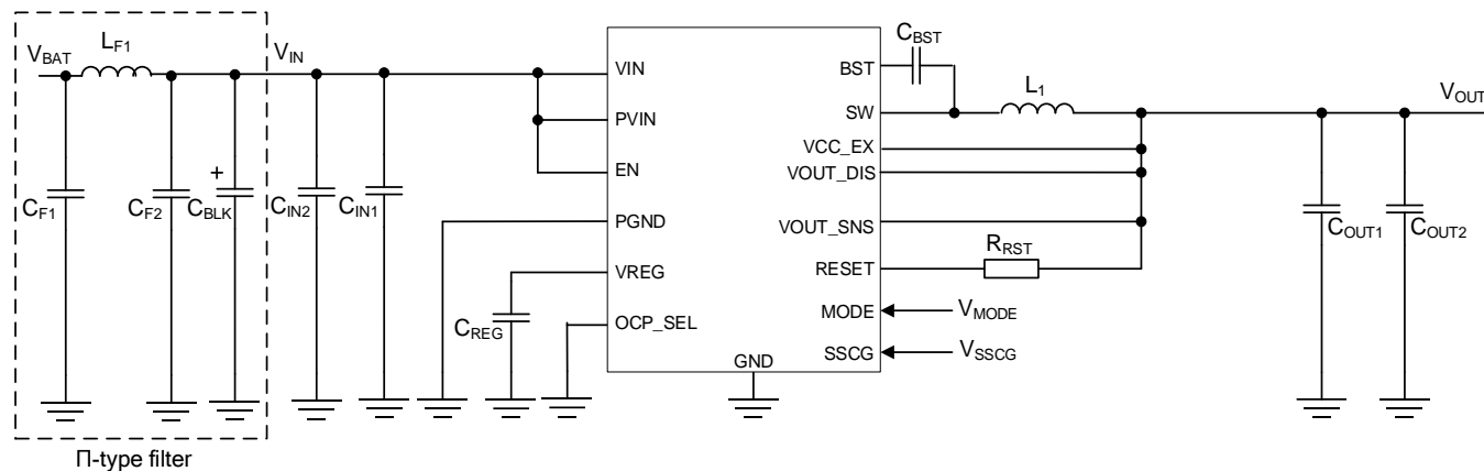
Figure 75. 参考回路 3
