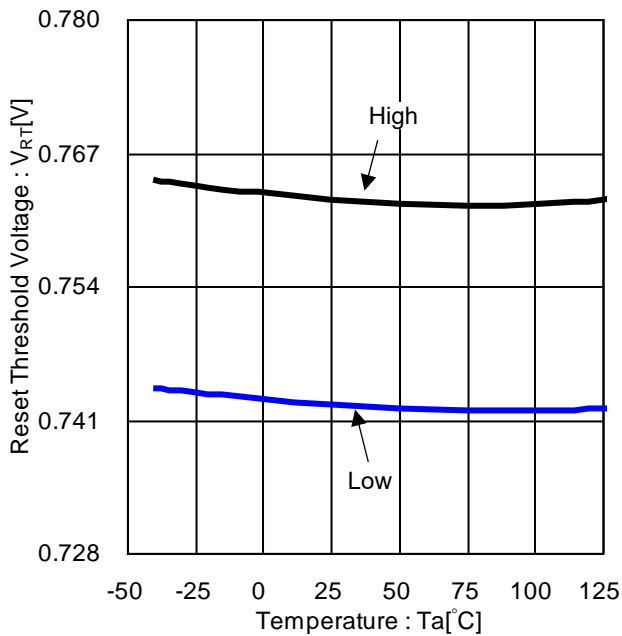
Figure 23. Reset スレッシュホールド電圧 vs 温度 (BD9P206EFV-C)
