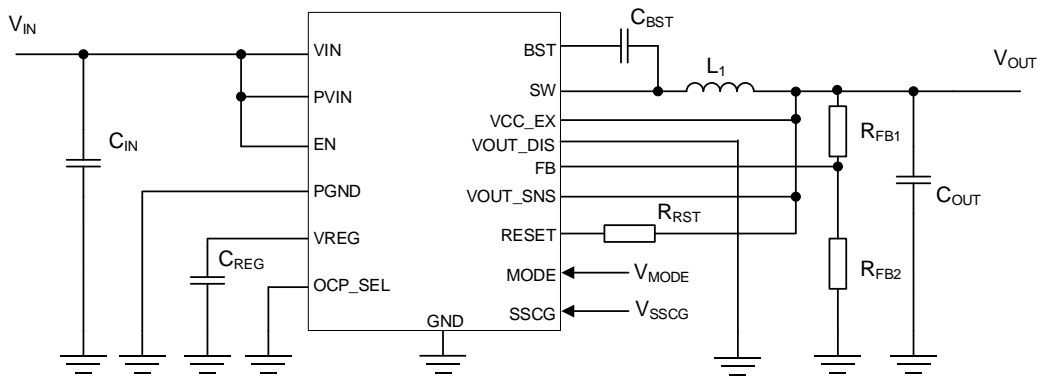
Figure 4. ディスチャージ機能を使用しないアプリケーション回路 (BD9P206EFV-C)
