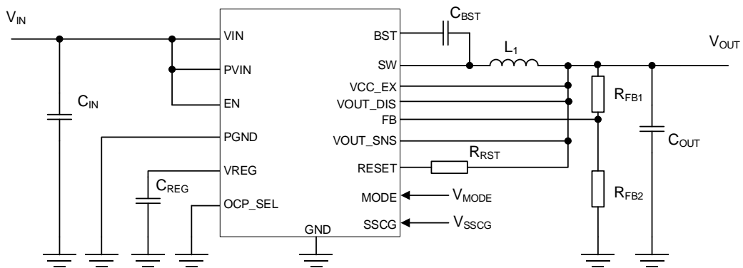
Figure 3. ディスチャージ機能を使用したアプリケーション回路 (BD9P206EFV-C)
