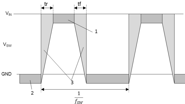
Figure 92. SW 波形
