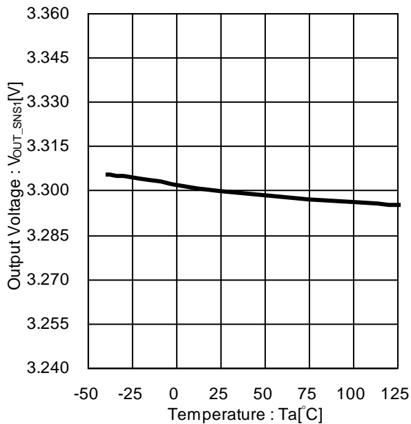
Figure 11. 出力電圧 vs 温度 (BD9P236EFV-C)
