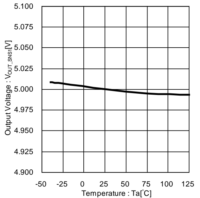
Figure 12. 出力電圧 vs 温度 (BD9P256EFV-C)
