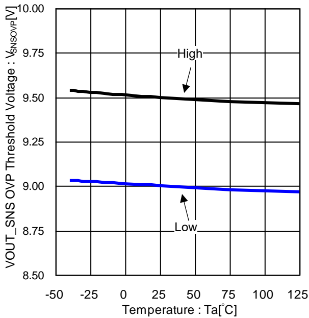
Figure 27. VOUT_SNS OVP スレッシュヨルド電圧 vs 温度 (BD9P206EFV-C)
