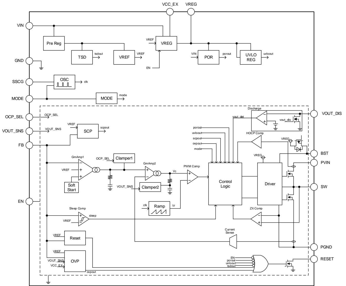
Figure 7. ブロック図 (BD9P206EFV-C)
