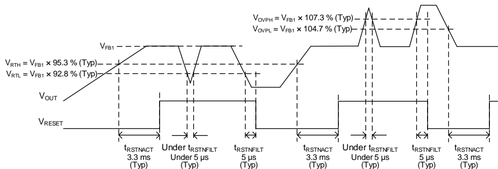
Figure 34. リセットタイミングチャート (BD9P206EFV-C)
