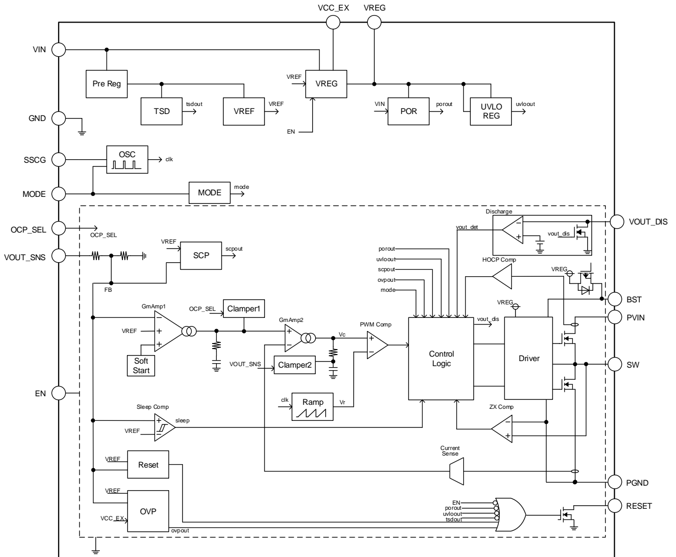
Figure 8. ブロック図 (BD9P236EFV-C, BD9P256EFV-C)
