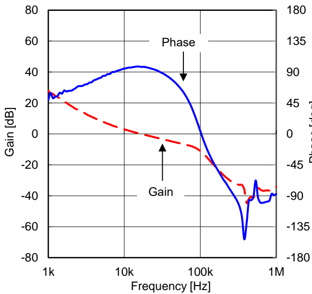
Figure 78. 周波数特性 ( V_{IN} = 12\text{ V} , I_{OUT} = 1.0\text{ A} )
