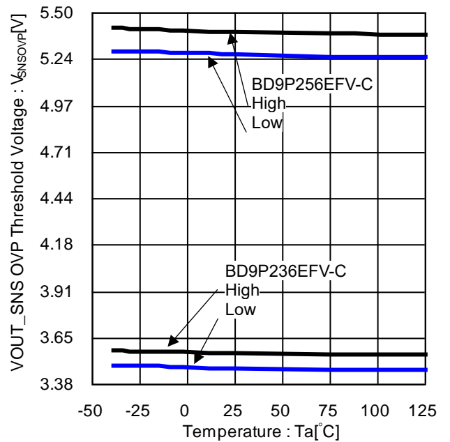
Figure 28. VOUT_SNS OVP スレッシュヨルド電圧 vs 温度 (BD9P236EFV-C/BD9P256EFV-C)
