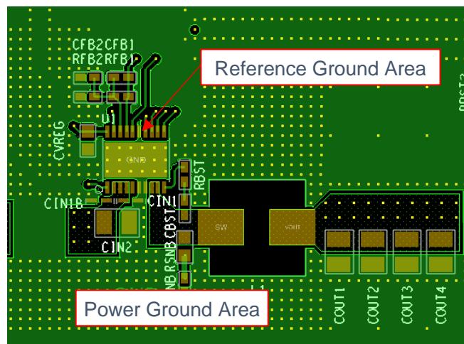
Figure 90. 推奨基板レイアウト例 (BD9P206EFV-C)
