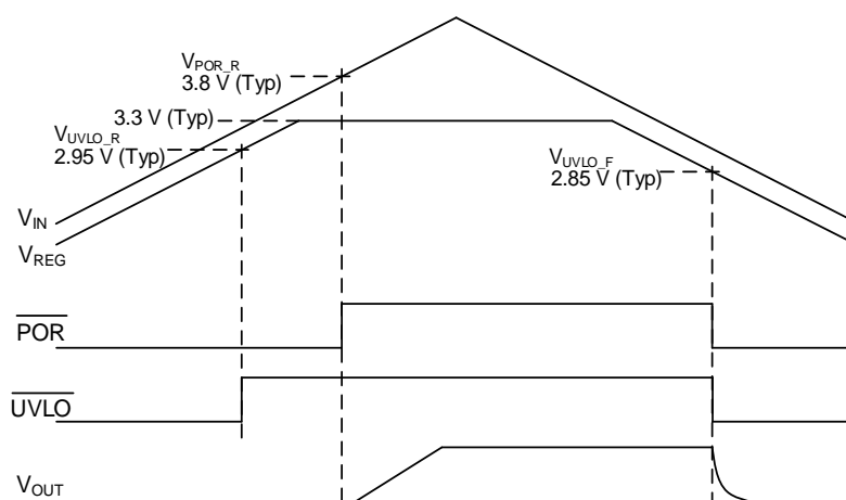
Figure 42. POR/UVLO タイミングチャート
