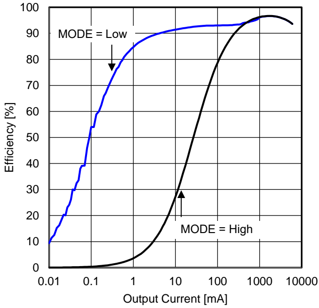
Figure 80. 効率 vs 出力負荷電流 ( V_{IN} = 12\text{ V} )
