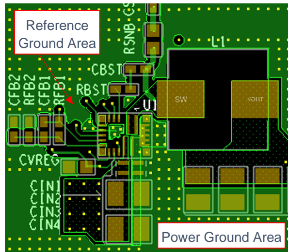
Figure 94. 推奨基板レイアウト例
