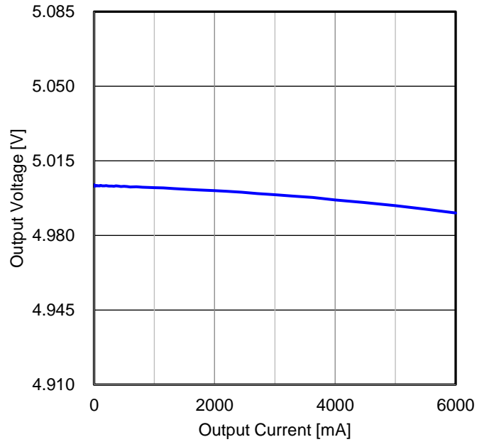
Figure 91. ロードレギュレーション ( V_{IN} = 12\text{ V} )
