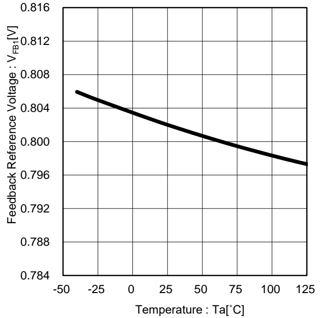
Figure 5. フィードバック電圧 vs 温度
