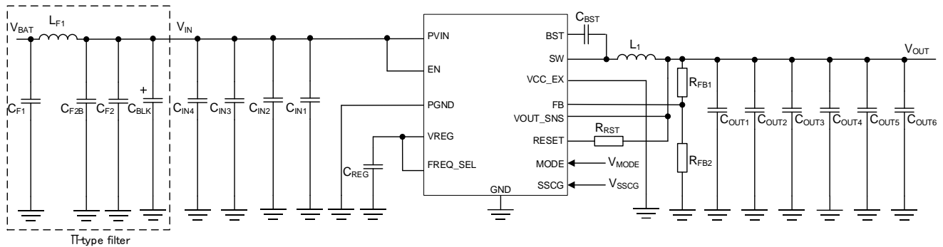
Figure 53. 参考回路 2
