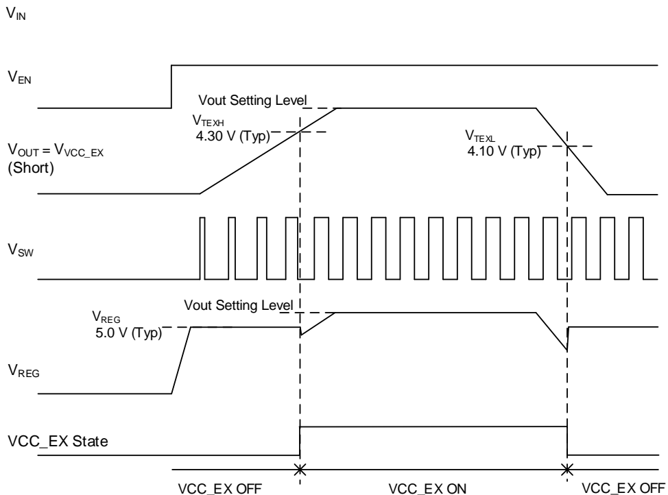
Figure 30. VCC_EX タイミングチャート
