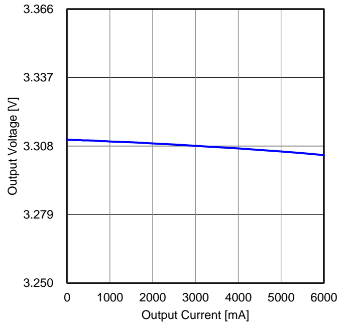
Figure 52. ロードレギュレーション (V IN = 12 V)
