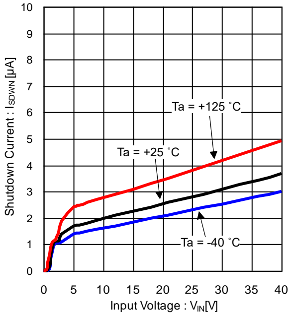
Figure 4. シャットダウン時電流 vs 入力電圧
