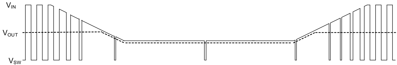
Figure 27. 分周機能 (FREQ_SEL = L)
