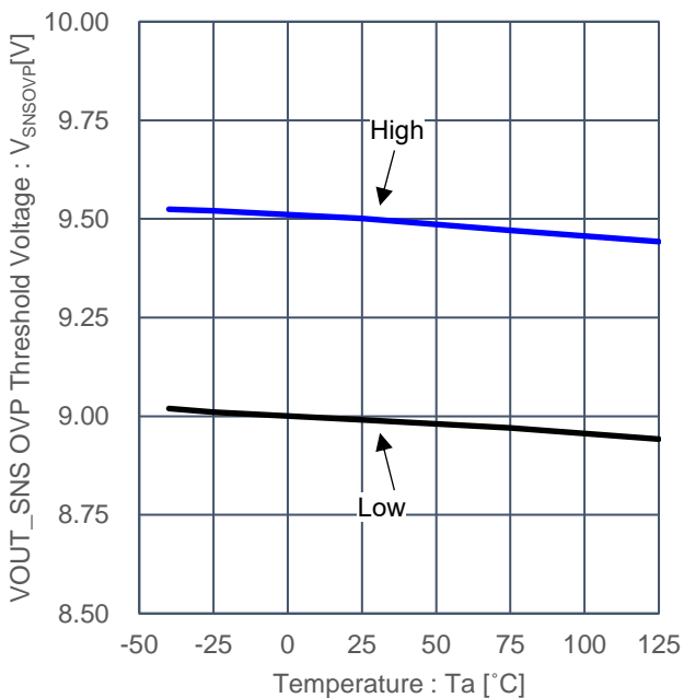
Figure 18. VOUT_SNS OVP スレッシュヨルド電圧 vs 温度
