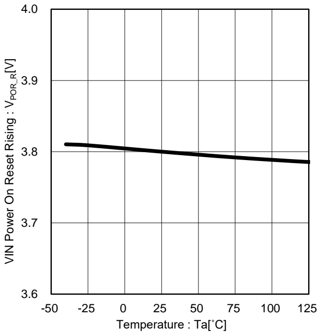
Figure 6. VIN POR 解除電圧 vs 温度
