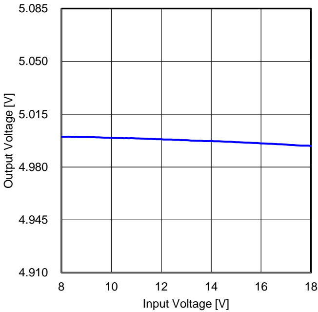
Figure 77. ラインレギュレーション 1 (I OUT = 3 A)
