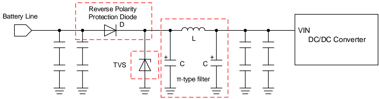
Figure 92. 車載電源供給ライン回路例
