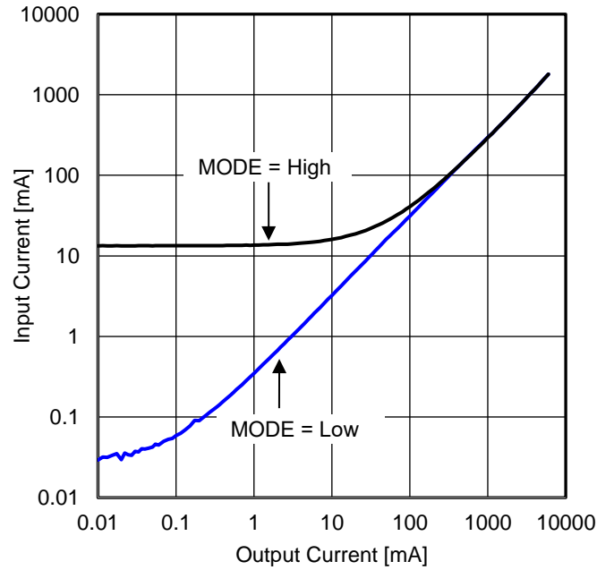
Figure 55. 入力電流 vs 出力負荷電流 ( V_{IN} = 12\text{ V} )
