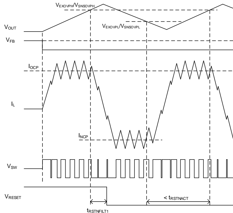
Figure 36. VCC_EX/VOUT_SNS OVP タイミングチャート (FREQ_SEL = L)
