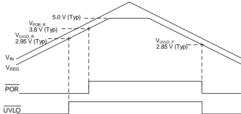
Figure 33. POR/UVLO タイミングチャート
