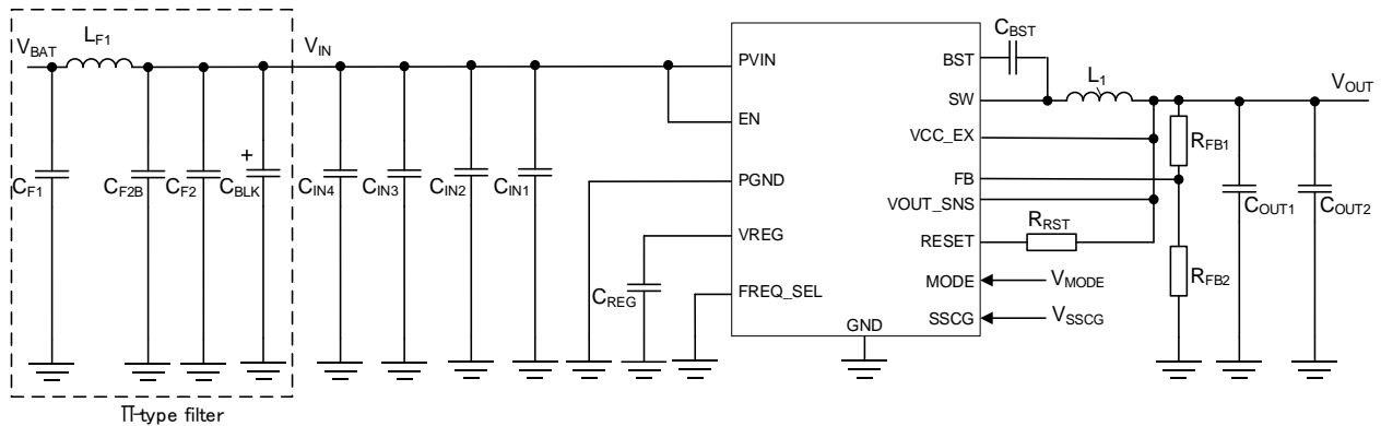
Figure 66. 参考回路 3
