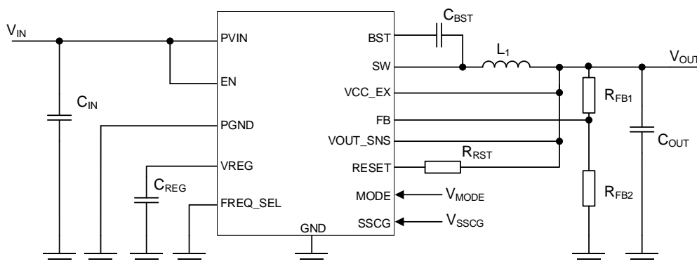
Figure 1. アプリケーション回路
