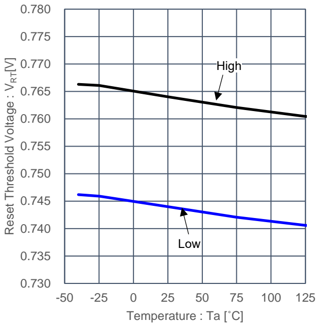
Figure 16. Reset スレッシュヨルド電圧 vs 温度
