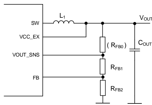
Figure 95. フィードバックの周波数特性測定用抵抗
