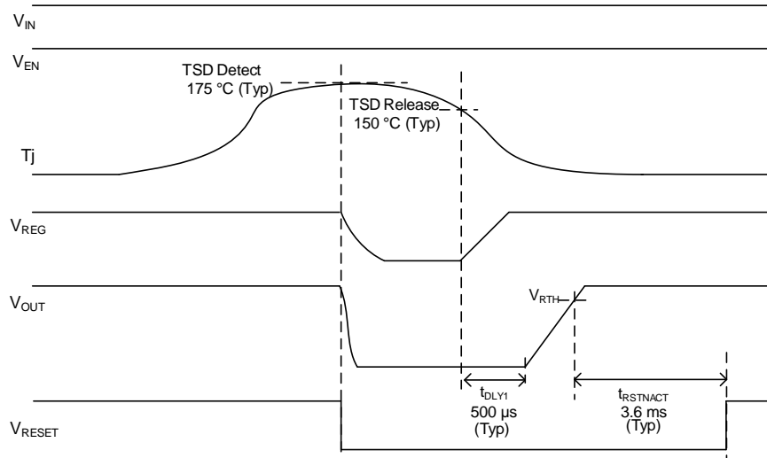
Figure 34. TSD タイミングチャート (FREQ_SEL = L)
