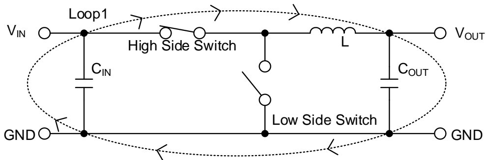
Figure 93 (a). High Side Switch : ON、Low Side Switch : OFF 時の電流経路
