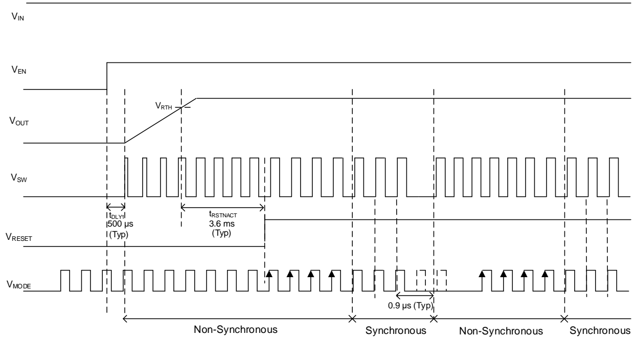
Figure 26. 外部同期機能 (FREQ_SEL = L)
