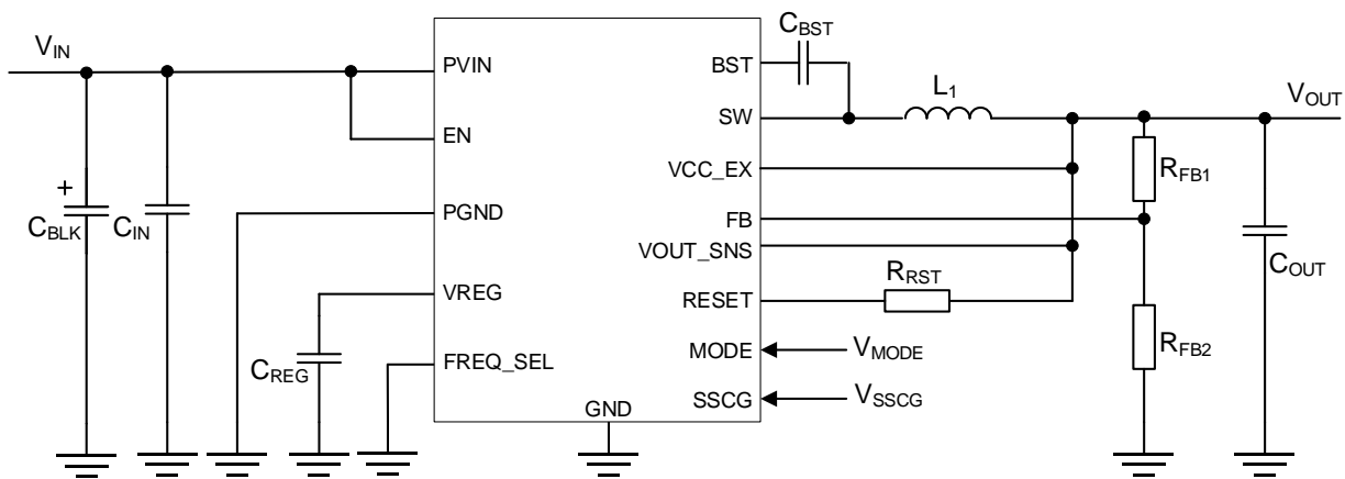
Figure 38. 参考回路
