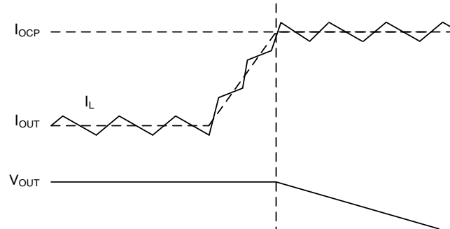
Figure 31. 過電流保護
