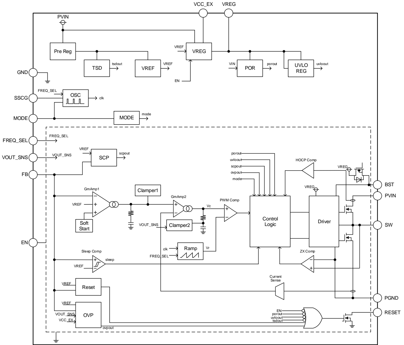
Figure 3. ブロック図
