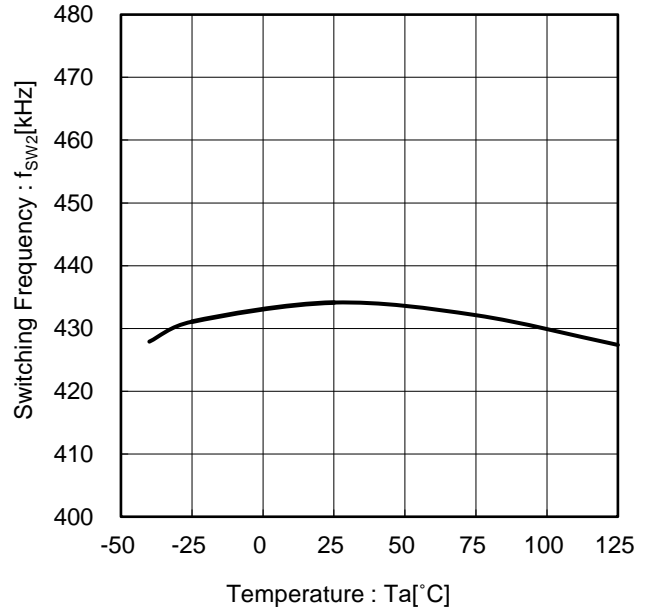
Figure 13. スイッチング周波数 vs 温度 (FREQ_SEL = High)
