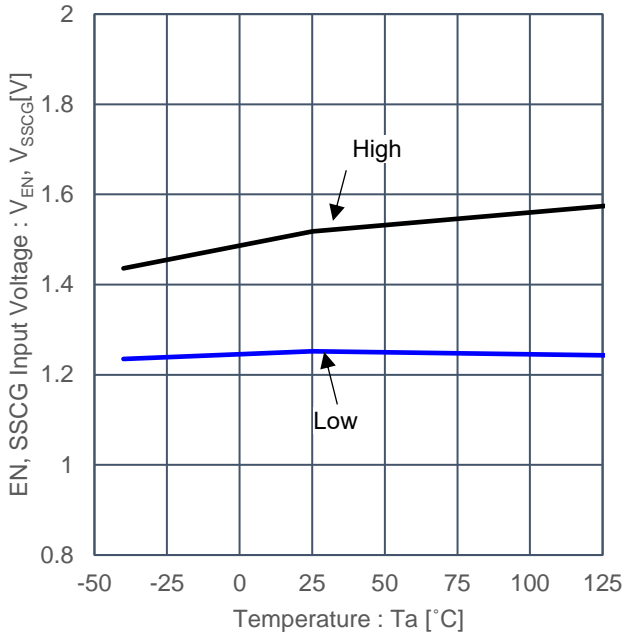
Figure 8. EN, SSCG 入力電圧 vs 温度
