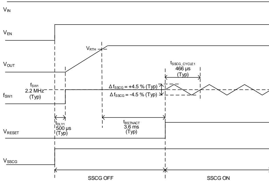
Figure 28. スペクトラム拡散機能 ( FREQ\_SEL = L )
