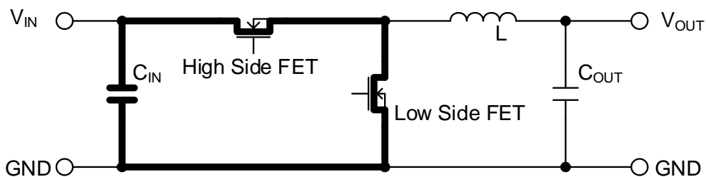
Figure 93 (c). 電流の差分、レイアウト上での重要箇所
