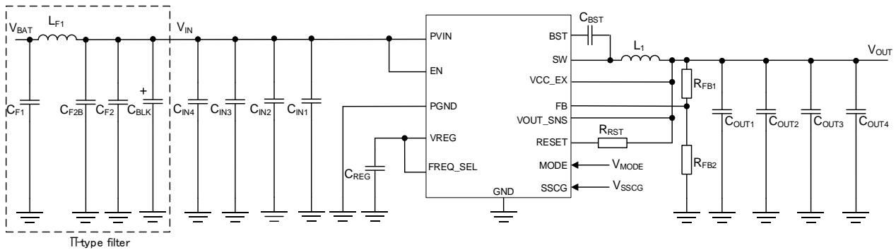
Figure 79. 参考回路 4
