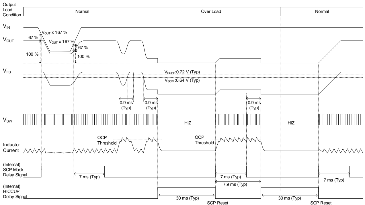
Figure 32. 短絡保護 (SCP) タイミングチャート (FREQ_SEL = L)
