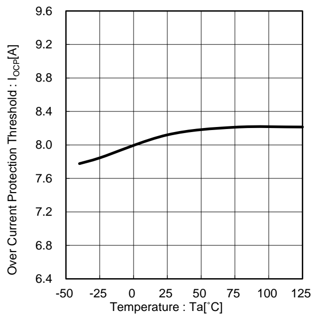
Figure 19. 過電流保護スレッシュヨルド vs 温度
