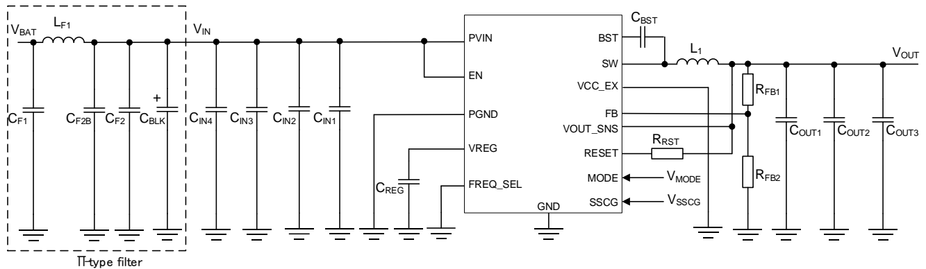
Figure 40. 参考回路 1
