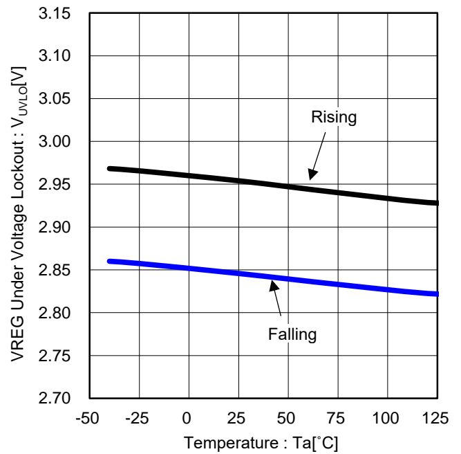
Figure 7. VREG UVLO 電圧 vs 温度
