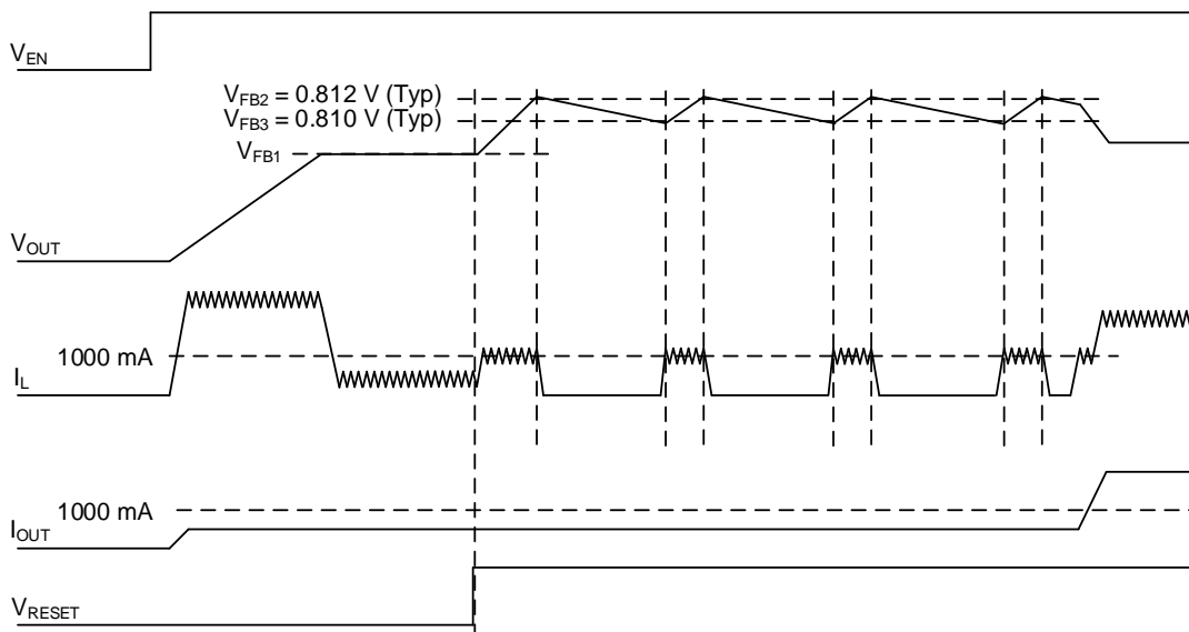
Figure 23. RESET の High 検出後の軽負荷モード中タイミングチャート
