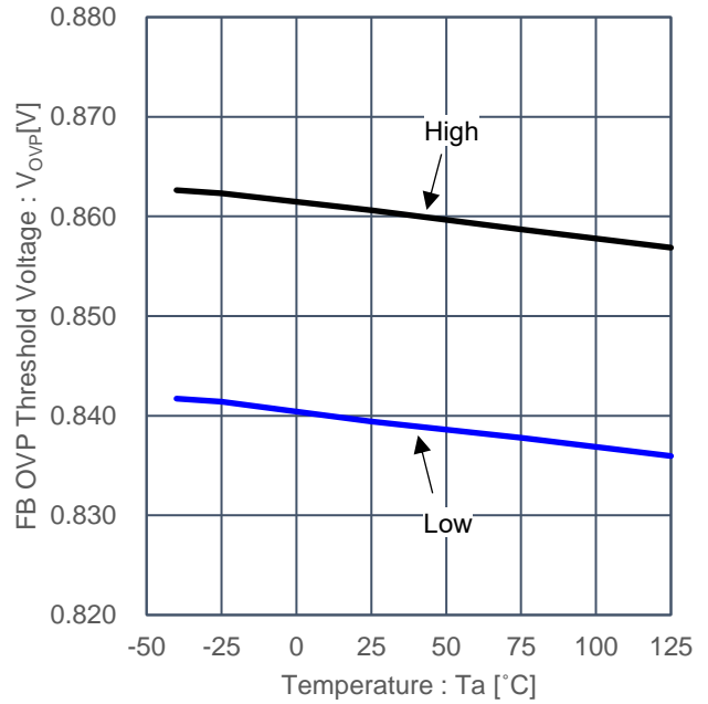
Figure 17. FB OVP スレッシュヨルド電圧 vs 温度
