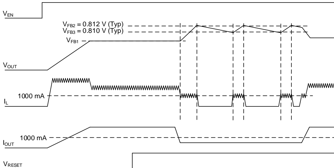
Figure 22. 軽負荷モード中タイミングチャート
