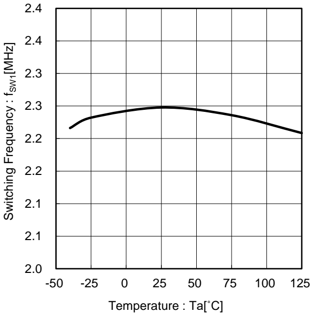
Figure 12. スイッチング周波数 vs 温度 (FREQ_SEL = Low)
