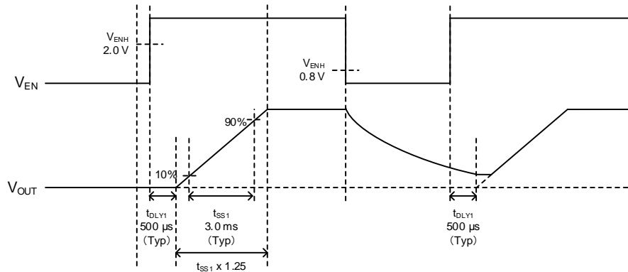
Figure 24. イネーブル ON/OFF タイミングチャート ( FREQ\_SEL = L )
