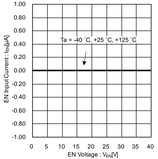
Figure 9. EN 流入電流 vs EN 電圧
