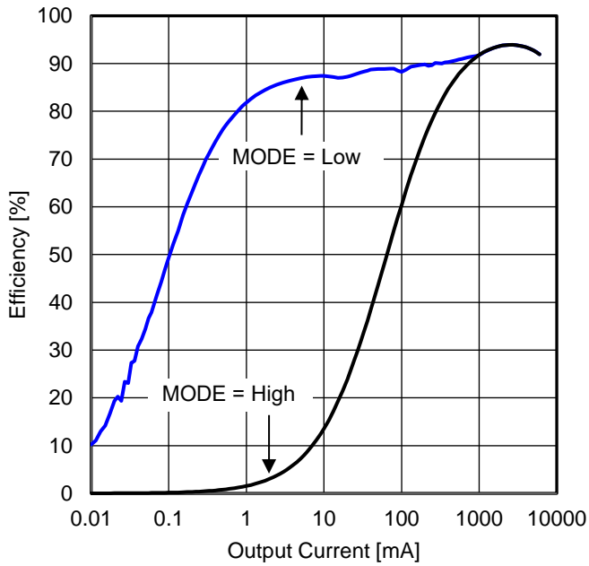
Figure 67. 効率 vs 出力負荷電流 ( V_{IN} = 12\text{ V} )
