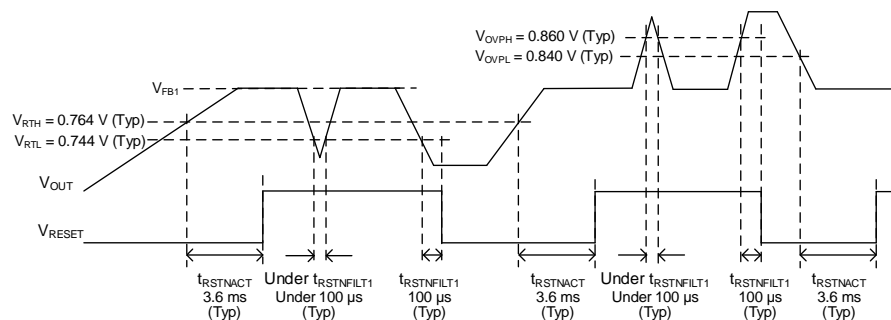
Figure 25. リセットタイミングチャート ( FREQ\_SEL = L )
