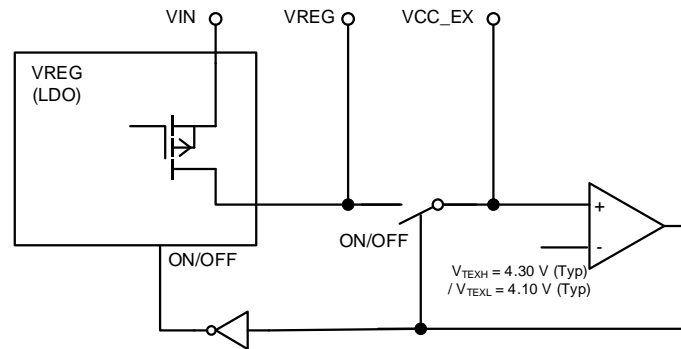
Figure 29. VCC_EX ブロック図
