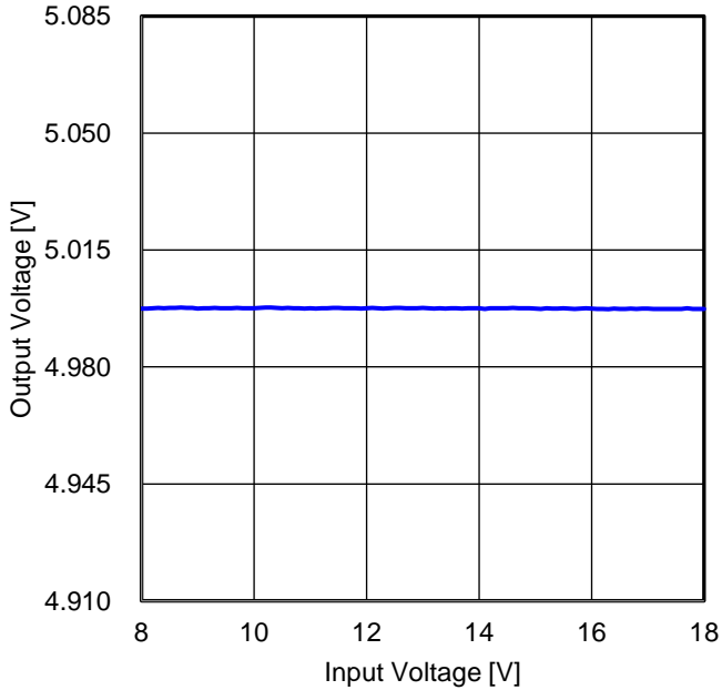
Figure 90. ラインレギュレーション ( I_{OUT} = 3\text{ A} )
