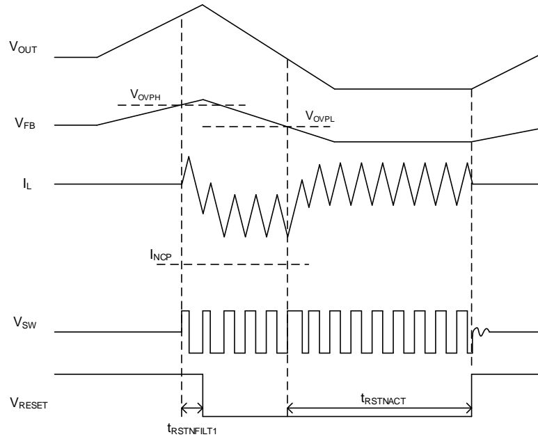
Figure 35. FB OVP タイミングチャート (FREQ_SEL = L)
