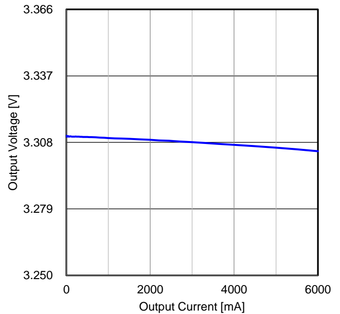
Figure 65. ロードレギュレーション ( V_{IN} = 12 V )
