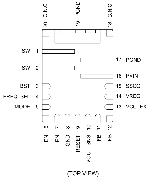
Figure 2. 端子配置図
