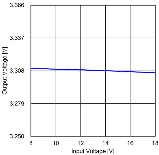
Figure 51. ラインレギュレーション (I OUT = 3 A)
