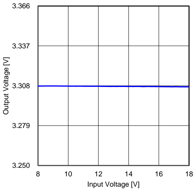
Figure 64. ラインレギュレーション ( I_{OUT} = 3 A )
