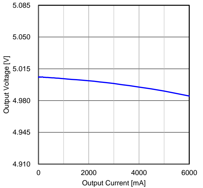
Figure 78. ロードレギュレーション 2 (V IN = 12 V)
