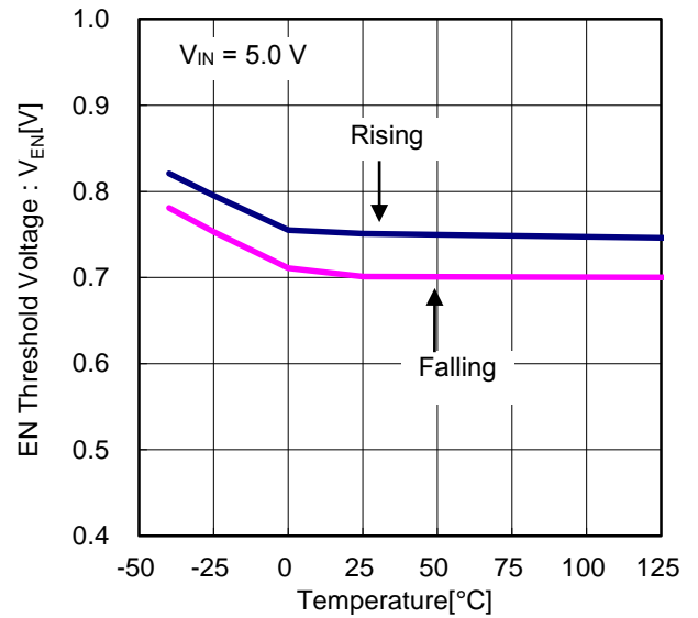
Figure 14. EN スレッシュヨルド電圧 vs 温度
