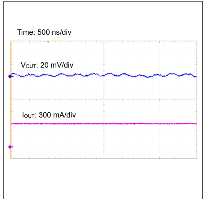
Figure 43. 出力リップル電圧 ( I_{OUT}=0.6\text{ A} )
