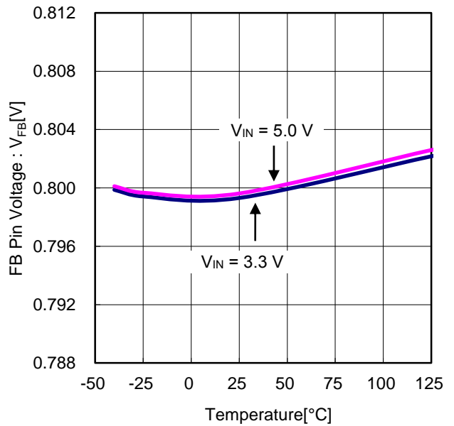
Figure 6. FB 端子電圧 vs 温度
