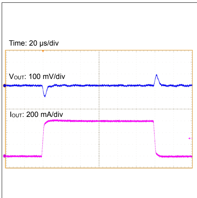
Figure 47. 負荷応答 ( I_{OUT}=0\text{ A} \leftrightarrow 0.6\text{ A} )
