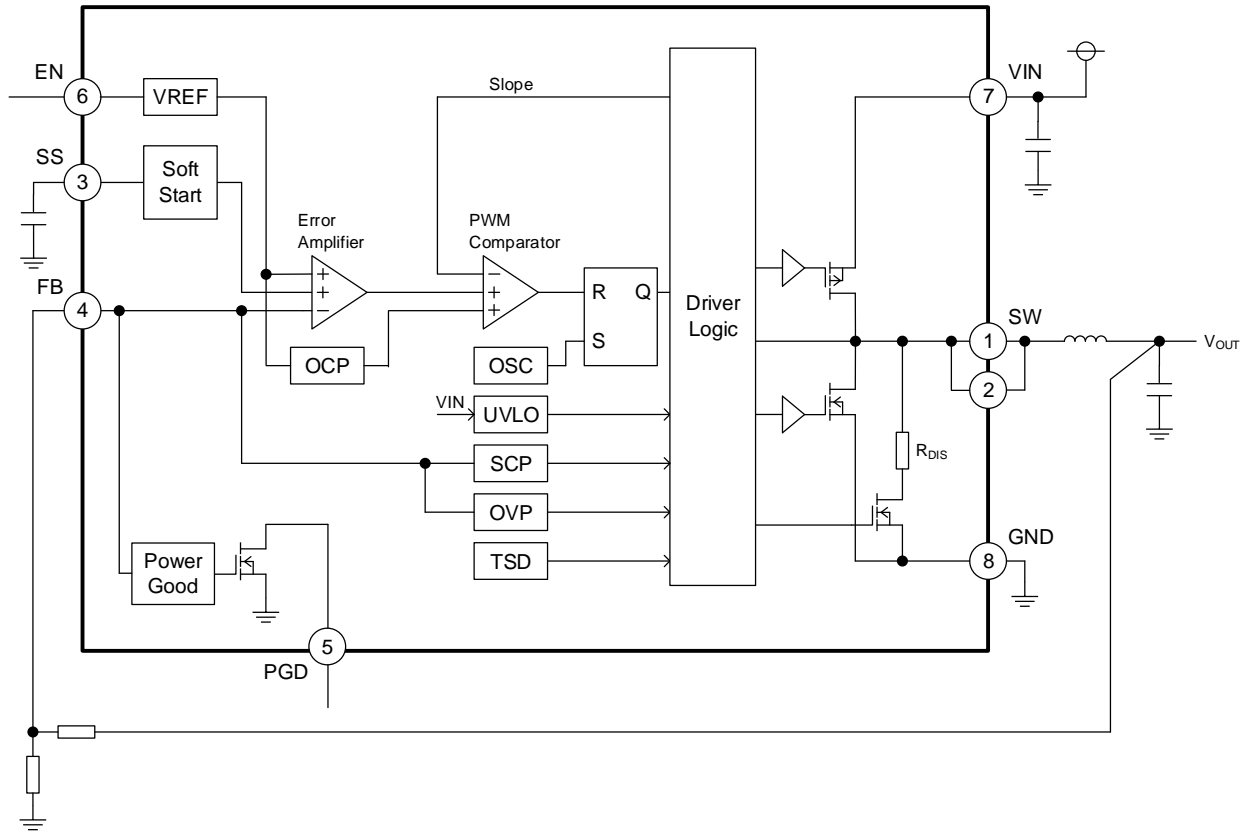
Figure 2. ブロック図
