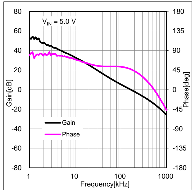
Figure 41. 周波数特性 ( I_{OUT}=0.6\text{ A} )
