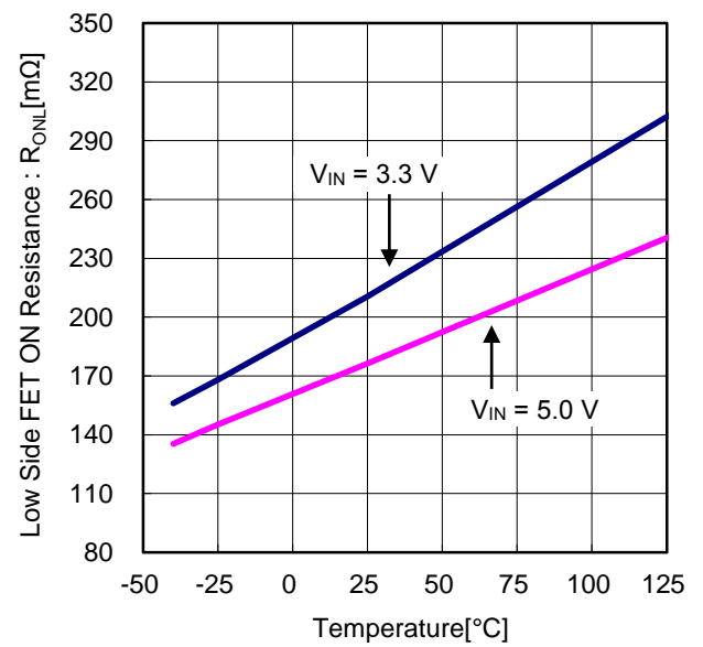
Figure 10. Low Side FET ON 抵抗 vs 温度
