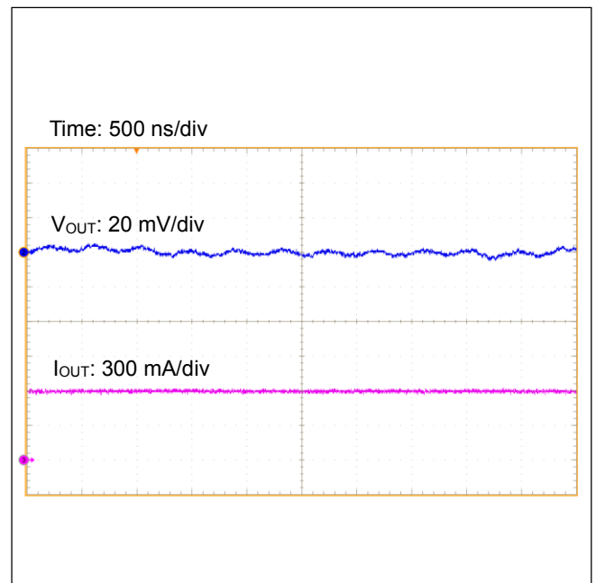
Figure 48. 出力リップル電圧 ( I_{OUT}=0.6\text{ A} )
