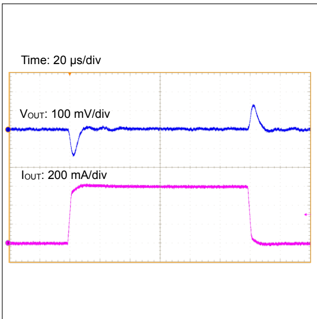
Figure 52. 負荷応答 ( I_{OUT}=0\text{ A} \leftrightarrow 0.6\text{ A} )
