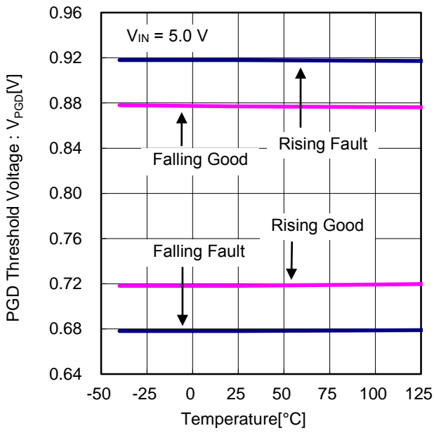
Figure 11. PGD スレッシュヨルド電圧 vs 温度
