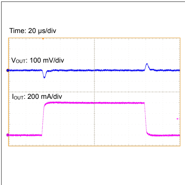
Figure 37. 負荷応答 ( I_{OUT}=0\text{ A} \leftrightarrow 0.6\text{ A} )
