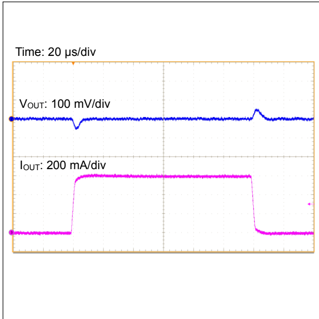
Figure 32. 負荷応答 ( I_{OUT}=0\text{ A} \leftrightarrow 0.6\text{ A} )
