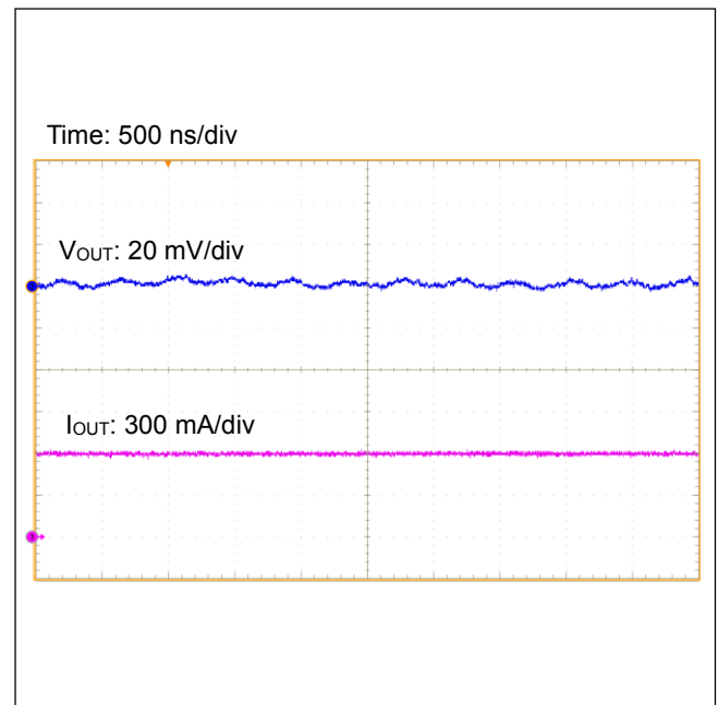
Figure 53. 出力リップル電圧 ( I_{OUT}=0.6\text{ A} )
