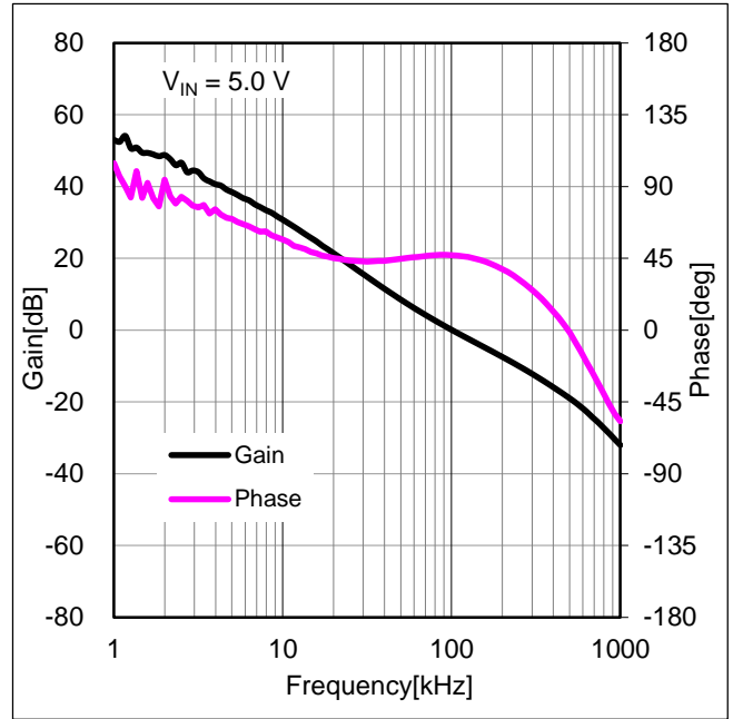
Figure 51. 周波数特性 ( I_{OUT}=0.6\text{ A} )
