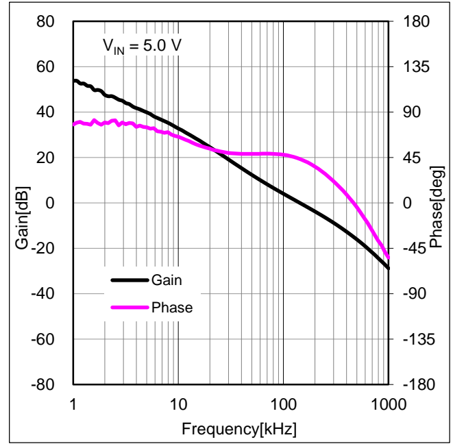
Figure 46. 周波数特性 ( I_{OUT}=0.6\text{ A} )
