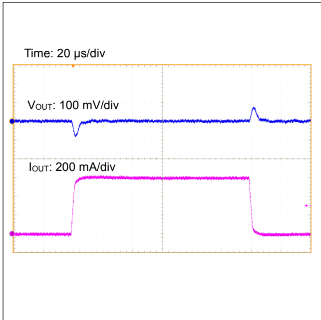
Figure 42. 負荷応答 ( I_{OUT}=0\text{ A}\leftrightarrow 0.6\text{ A} )
