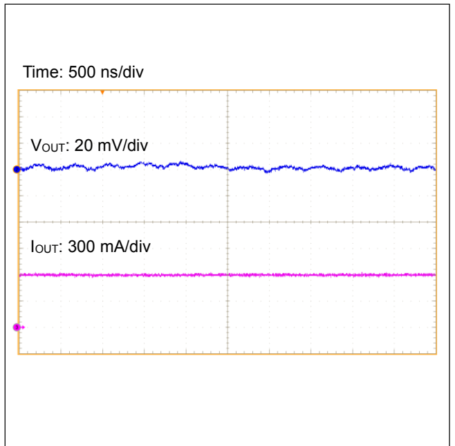
Figure 38. 出力リップル電圧 ( I_{OUT}=0.6\text{ A} )
