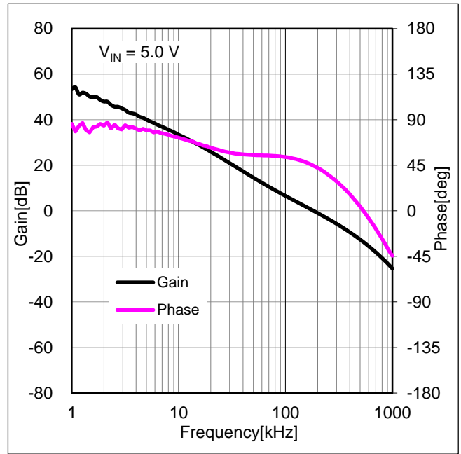
Figure 36. 周波数特性 ( I_{OUT}=0.6\text{ A} )
