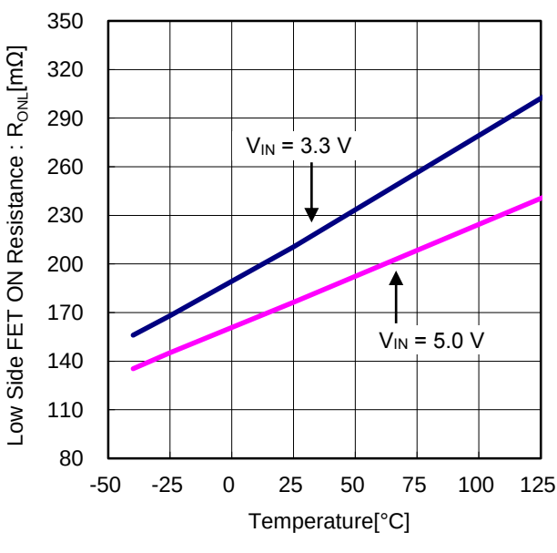
Figure 10. Low Side FET ON 抵抗 vs 温度
