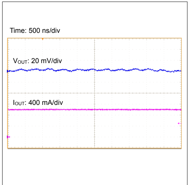
Figure 38. 出力リップル電圧 ( I_{OUT}=1\text{ A} )
