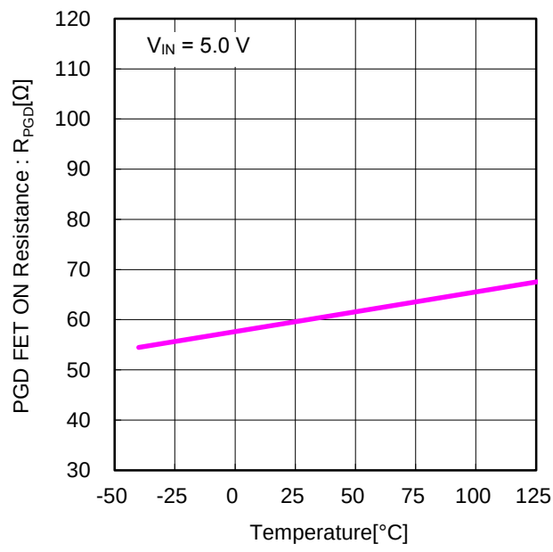
Figure 12. PGD FET ON 抵抗 vs 温度
