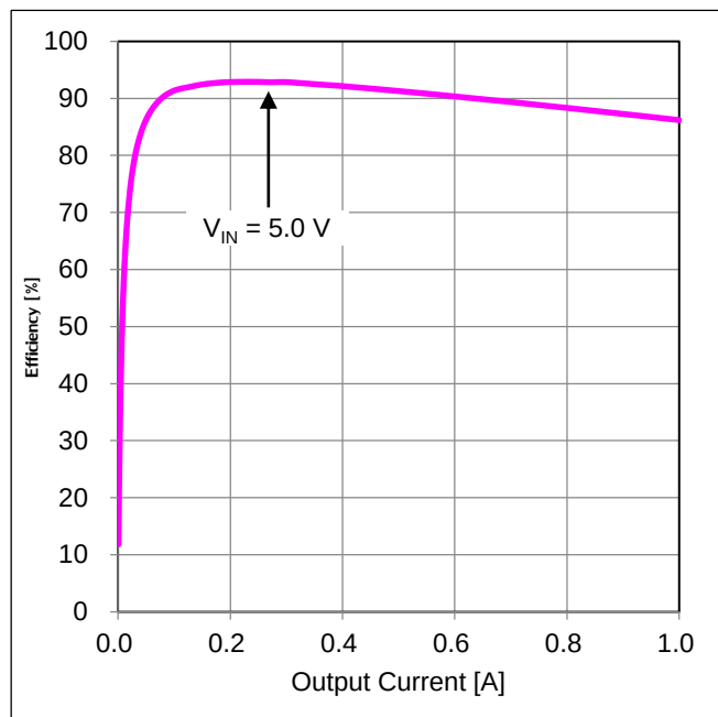
Figure 50. 効率 vs 出力電流
