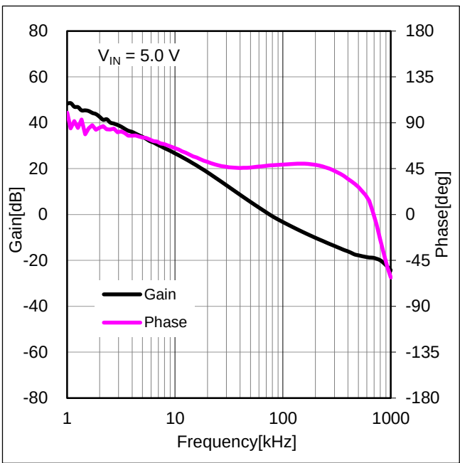
Figure 51. 周波数特性 ( I_{OUT}=1\text{ A} )
