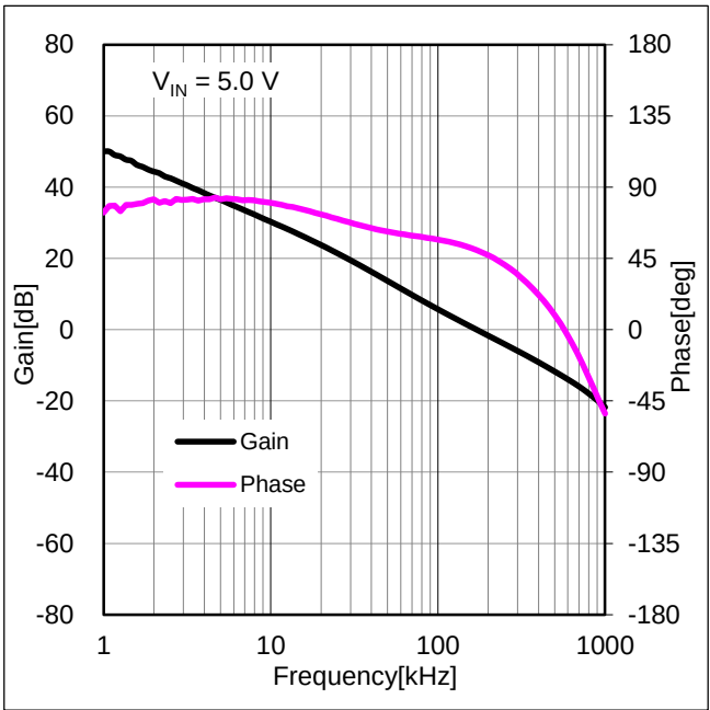
Figure 31. 周波数特性 ( I_{OUT} = 1\text{ A} )
