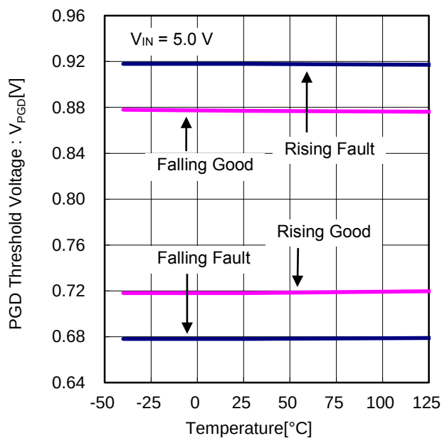
Figure 11. PGD スレッシュホールド電圧 vs 温度
