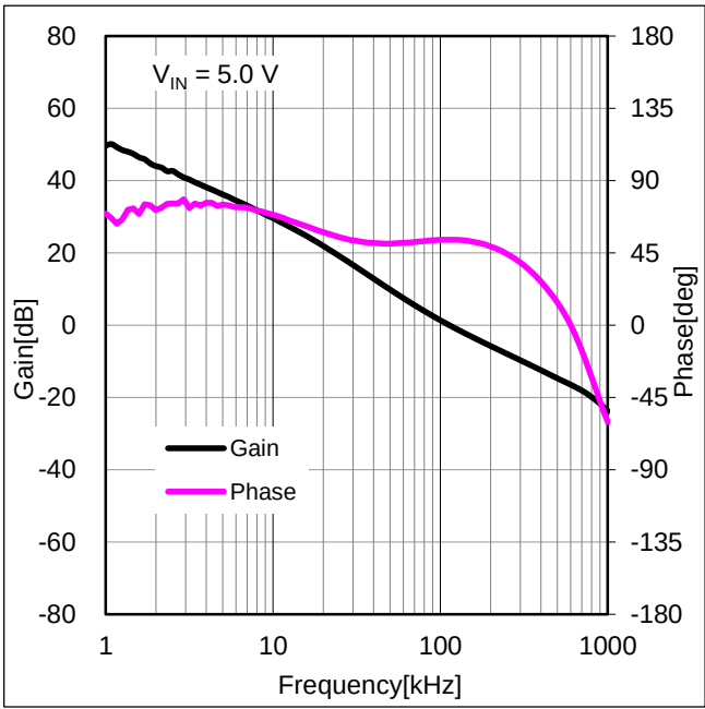
Figure 46. 周波数特性 ( I_{OUT} = 1\text{ A} )
