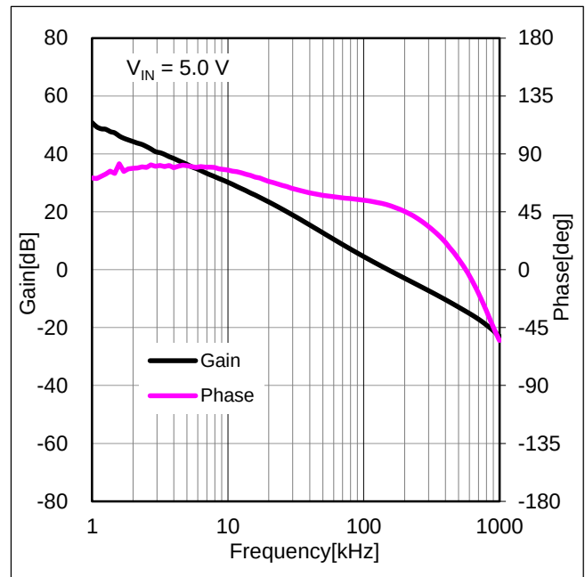
Figure 36. 周波数特性 ( I_{OUT}=1\text{ A} )
