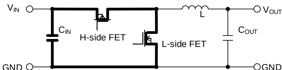
Figure 54-c. 電流の差分、レイアウト上での重要箇所
