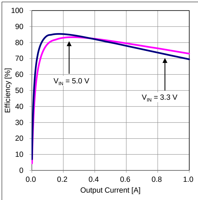
Figure 35. 効率 vs 出力電流
