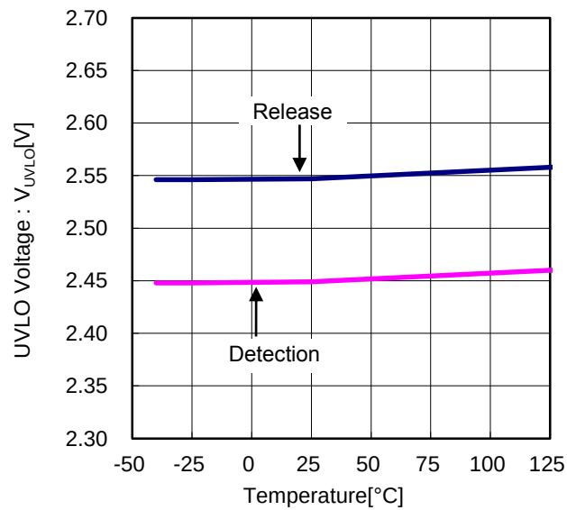
Figure 13. UVLO 電圧 vs 温度
