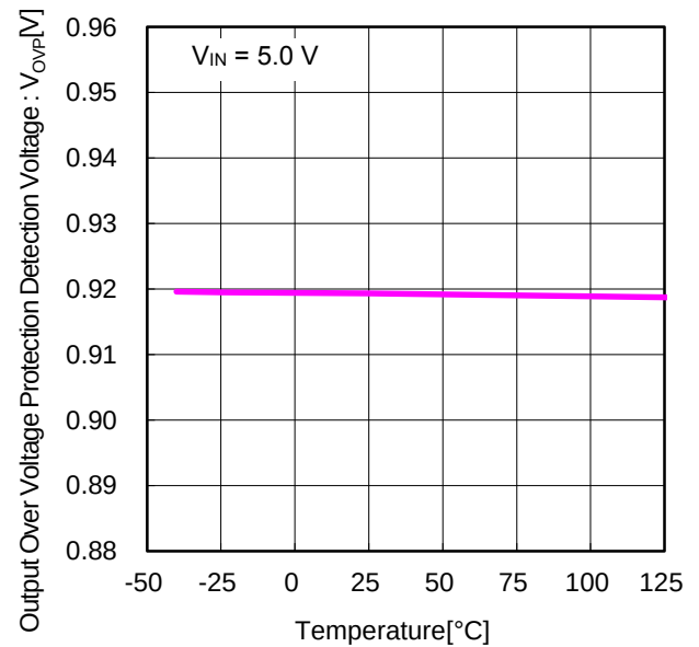
Figure 18. 出力過電圧保護検出電圧 vs 温度
