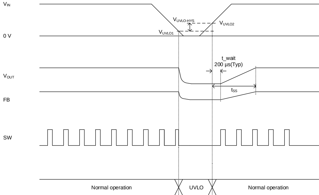
Figure 22. UVLO タイミングチャート
