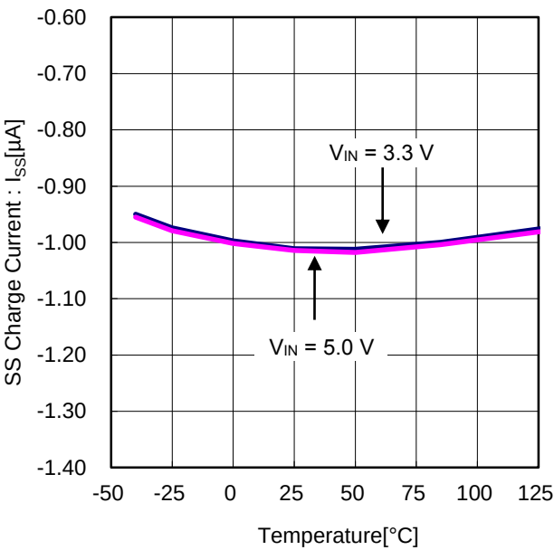
Figure 8. SS 充電電流 vs 温度
