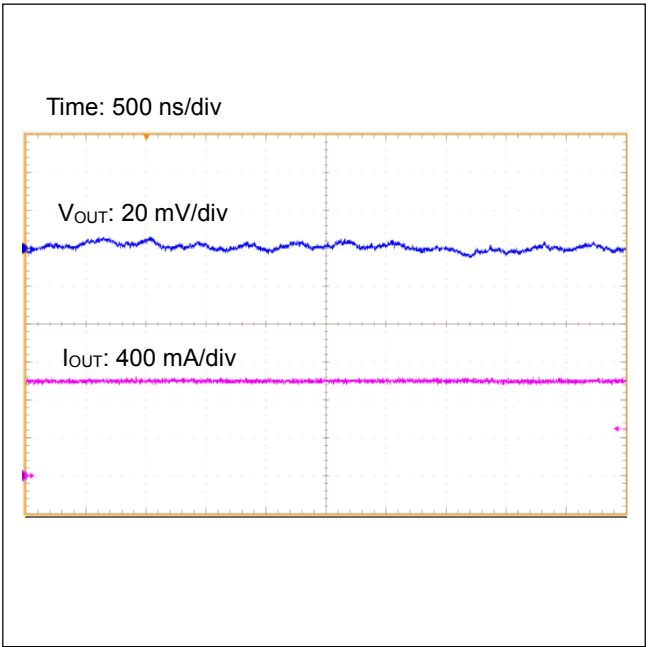
Figure 43. 出力リップル電圧 ( I_{OUT} = 1\text{ A} )
