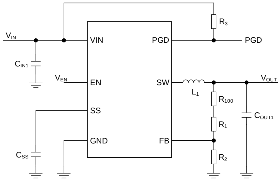
Figure 24. アプリケーション回路
