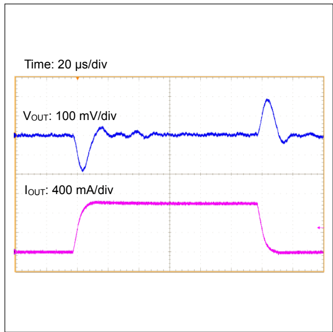
Figure 52. 負荷応答 ( I_{OUT}=0\text{ A} \leftrightarrow 1\text{ A} )
