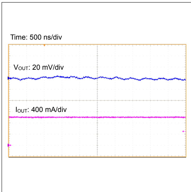
Figure 53. 出力リップル電圧 ( I_{OUT}=1\text{ A} )
