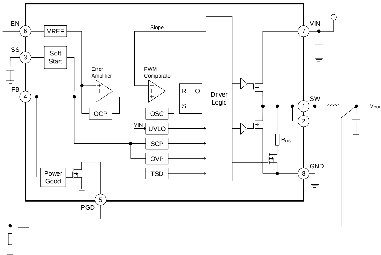
Figure 2. ブロック図
