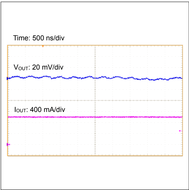
Figure 48. 出力リップル電圧 ( I_{OUT} = 1\text{ A} )
