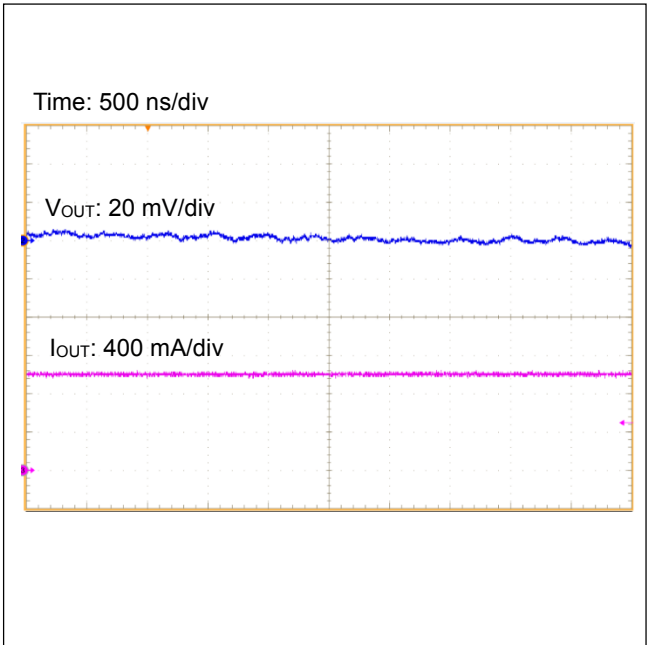
Figure 33. 出力リップル電圧 ( I_{OUT} = 1\text{ A} )
