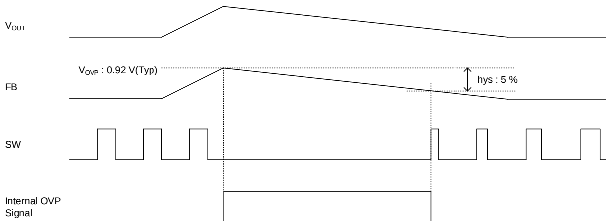
Figure 23. OVP タイミングチャート
