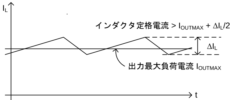
Figure 26. インダクタに流れる電流波形
