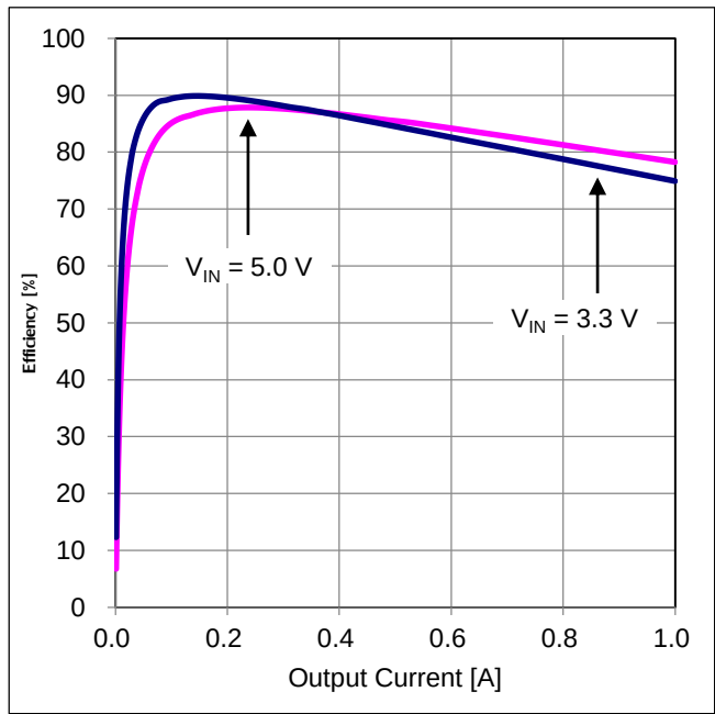
Figure 45. 効率 vs. 出力電流
