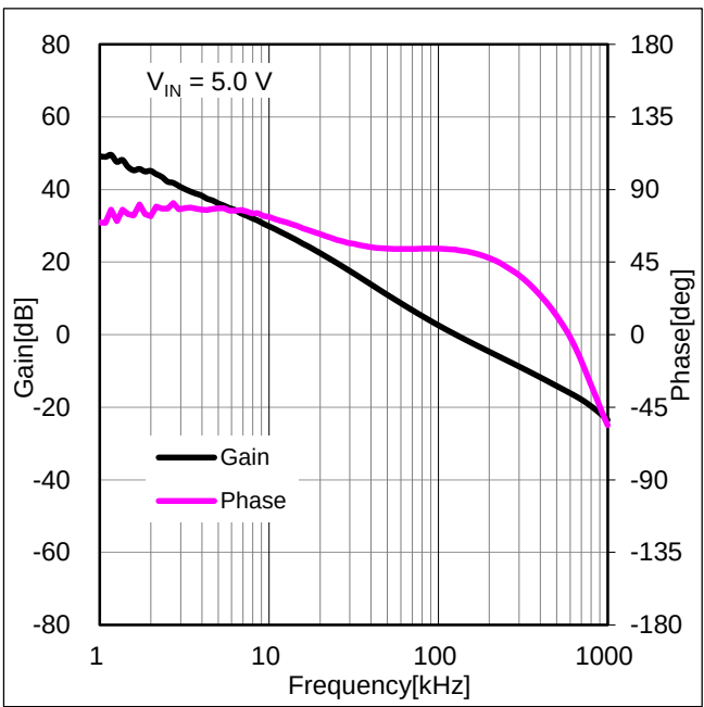
Figure 41. 周波数特性 ( I_{OUT} = 1\text{ A} )
