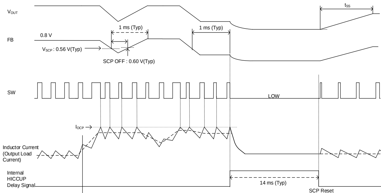
Figure 21. 負荷短絡保護機能(SCP)タイミングチャート
