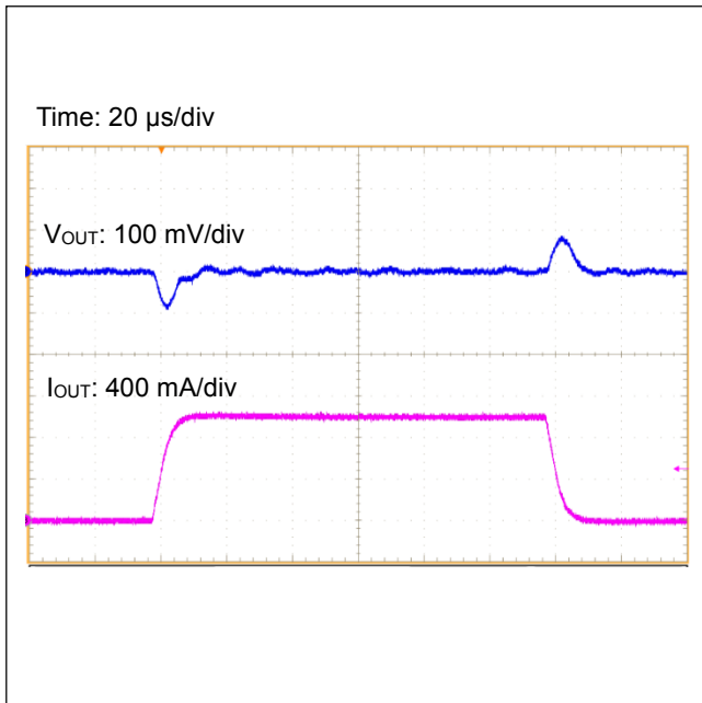
Figure 37. 負荷応答 ( I_{OUT}=0\text{ A} \leftrightarrow 1\text{ A} )
