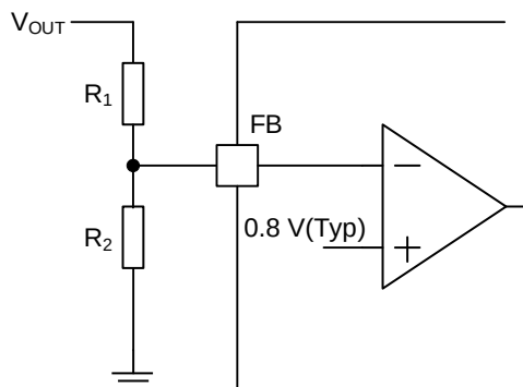
Figure 25. フィードバック抵抗回路
