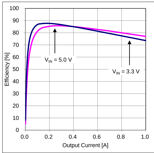
Figure 40. 効率 vs 出力電流
