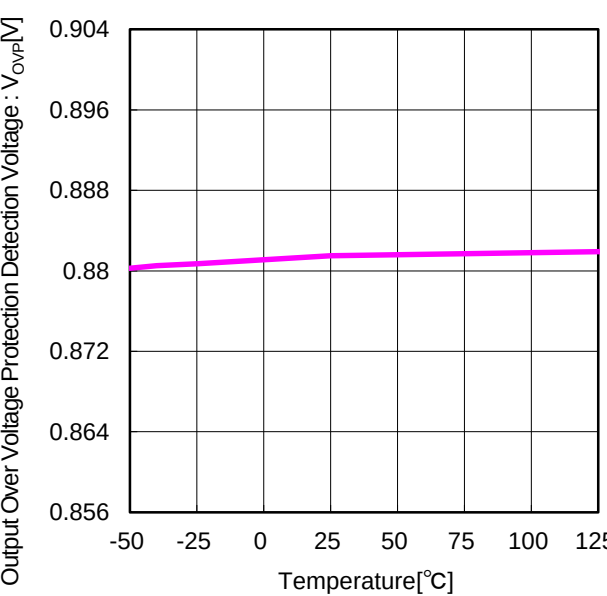
Figure 23. 出力過電圧保護検出電圧 vs 温度
