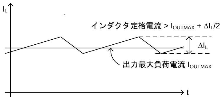
Figure 36. インダクタに流れる電流波形
