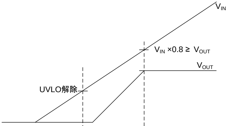
Figure 40. 入力電圧起動時間
