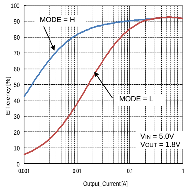
Figure 22. 効率 vs 負荷電流 ( V_{IN}=5V , V_{OUT}=1.8V , L=2.2\mu H )
