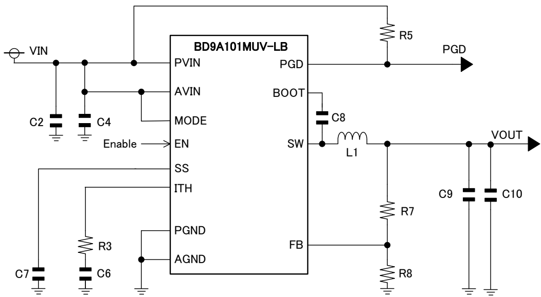
Figure 47. アプリケーション回路
