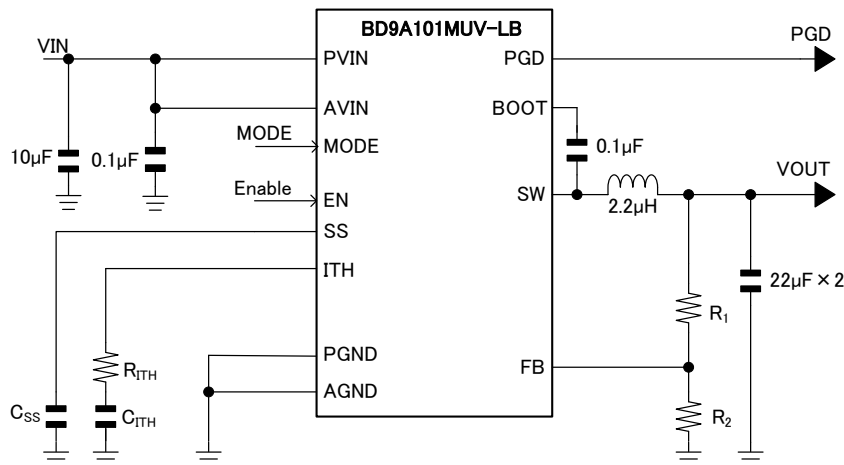
Figure 1. アプリケーション回路
