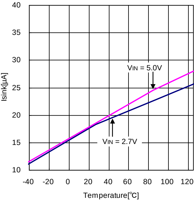
Figure 8. ITH シンク電流 vs 温度
