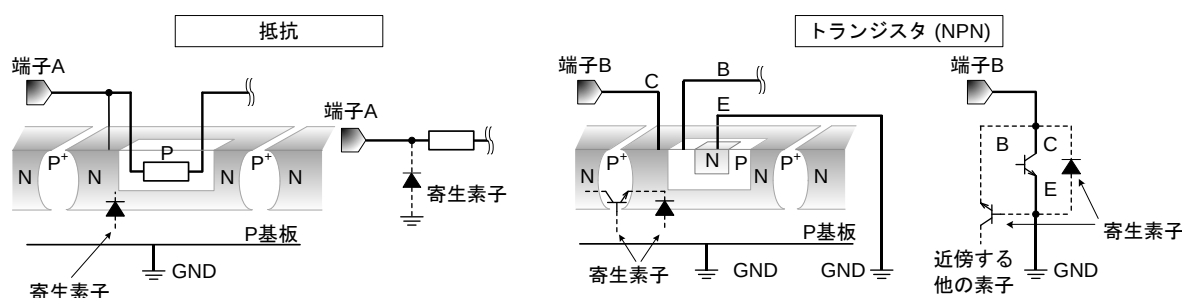
Figure 56. モノリシック IC 構造例
