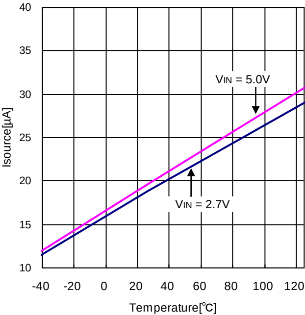
Figure 9. ITH ソース電流 vs 温度
