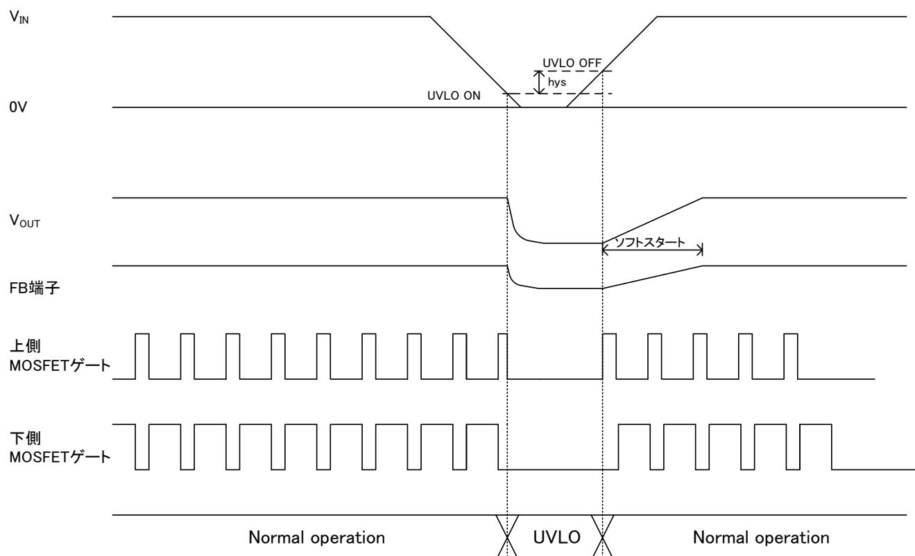
Figure 46. UVLO タイミングチャート
