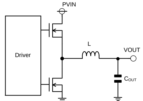
Figure 49. 出力 LC フィルタ回路
