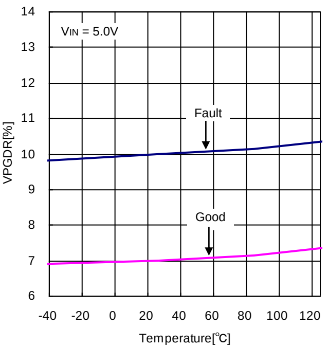
Figure 17. PGD Rising 電圧 vs 温度
