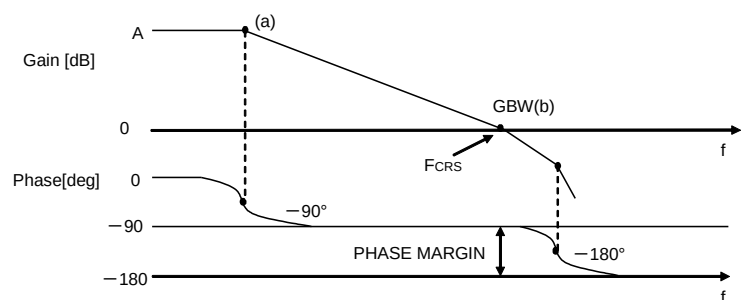
Figure 52. ボード線図
