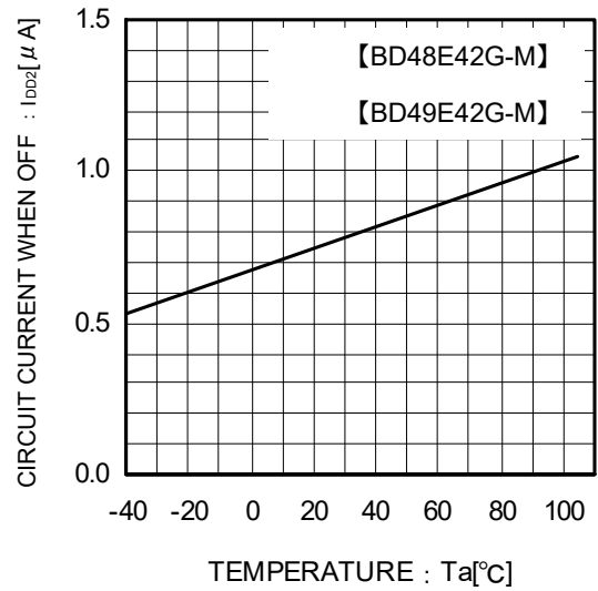
Fig.10 OFF 時回路電流
