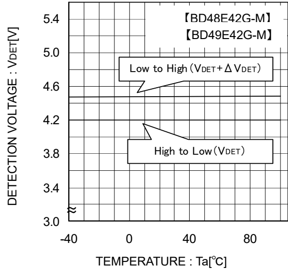
Fig.8 検出電圧 解除電圧
