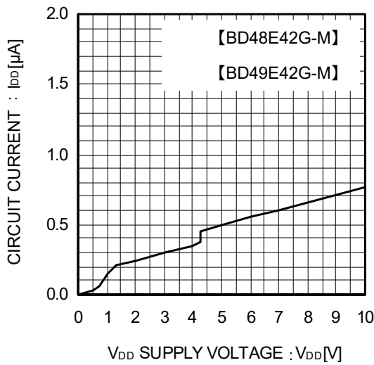
Fig.3 回路電流
