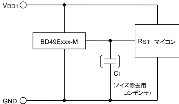
Fig.16 CMOS 出力タイプ
