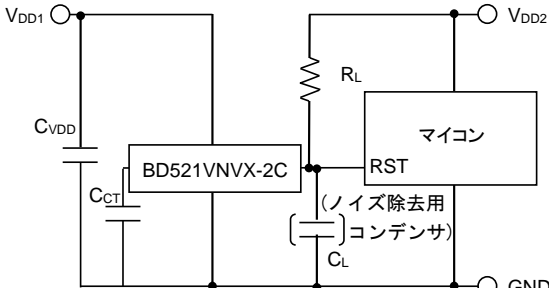
Figure 1. オープンドレイン出力タイプ BD521VNVX-2C
