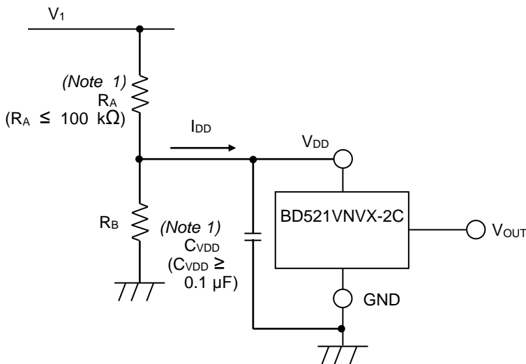
Figure 22. 抵抗分割での使用例
