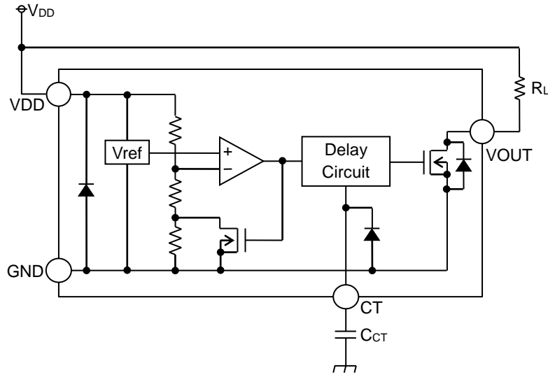
Figure 18. BD521VNVX-2C セットアップ図
