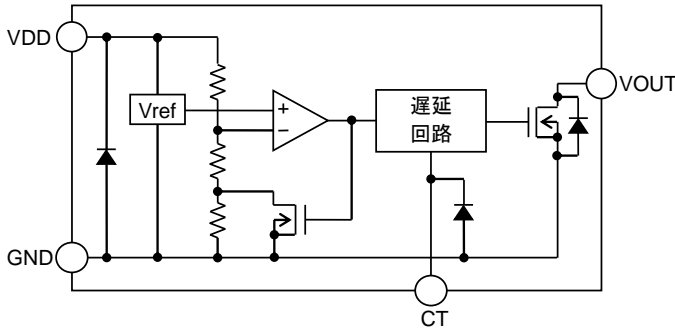
Figure 17. (BD521VNVX-2C タイプ内部ブロック図)
