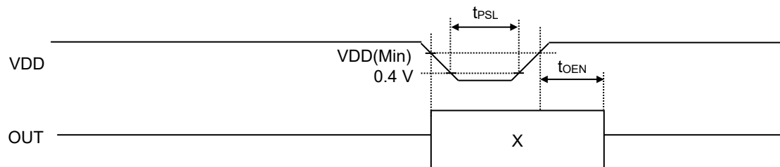
Figure 9. 電源 OFF 時のタイミングチャート
