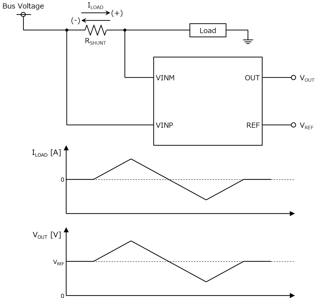
Figure 7. 基本動作説明
