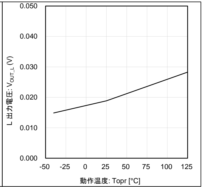
Figure 6. L出力電圧 vs 動作温度
