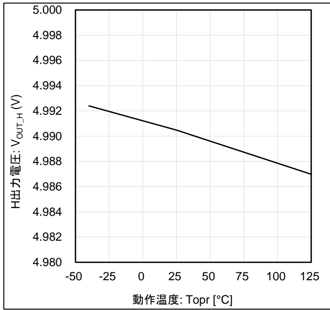
Figure 5. H出力電圧 vs 動作温度
