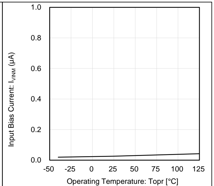
Figure 4. 入力電流 vs 動作温度
