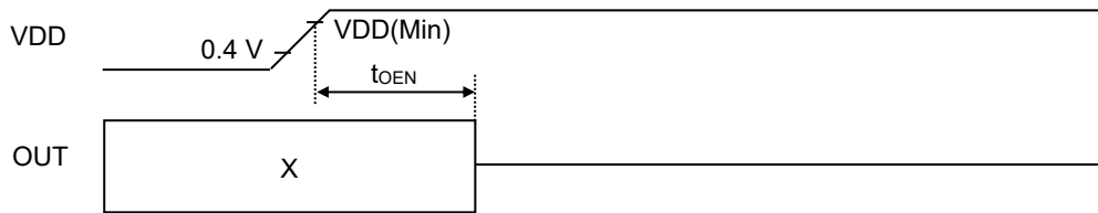
Figure 8. 電源投入時のタイミングチャート
