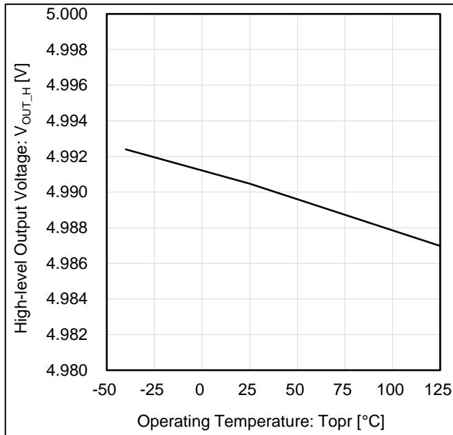
Figure 5. H 出力電圧 vs 動作温度
