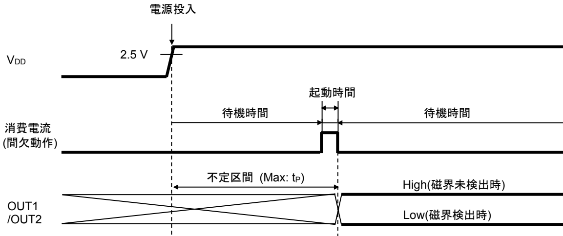
Figure 16. 電源投入時の間欠動作のタイミングチャート
