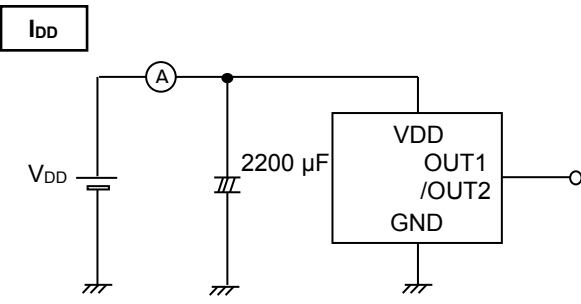
Figure 4. IDD 測定回路図
