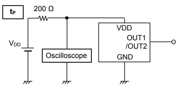
Oscilloscopeにて周期をモニタ
