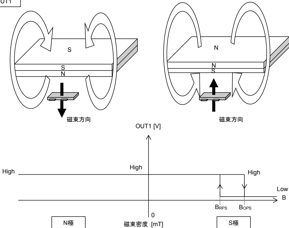
Figure 14. S 極検出動作
