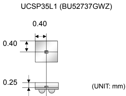
Figure 17. ホール素子位置
