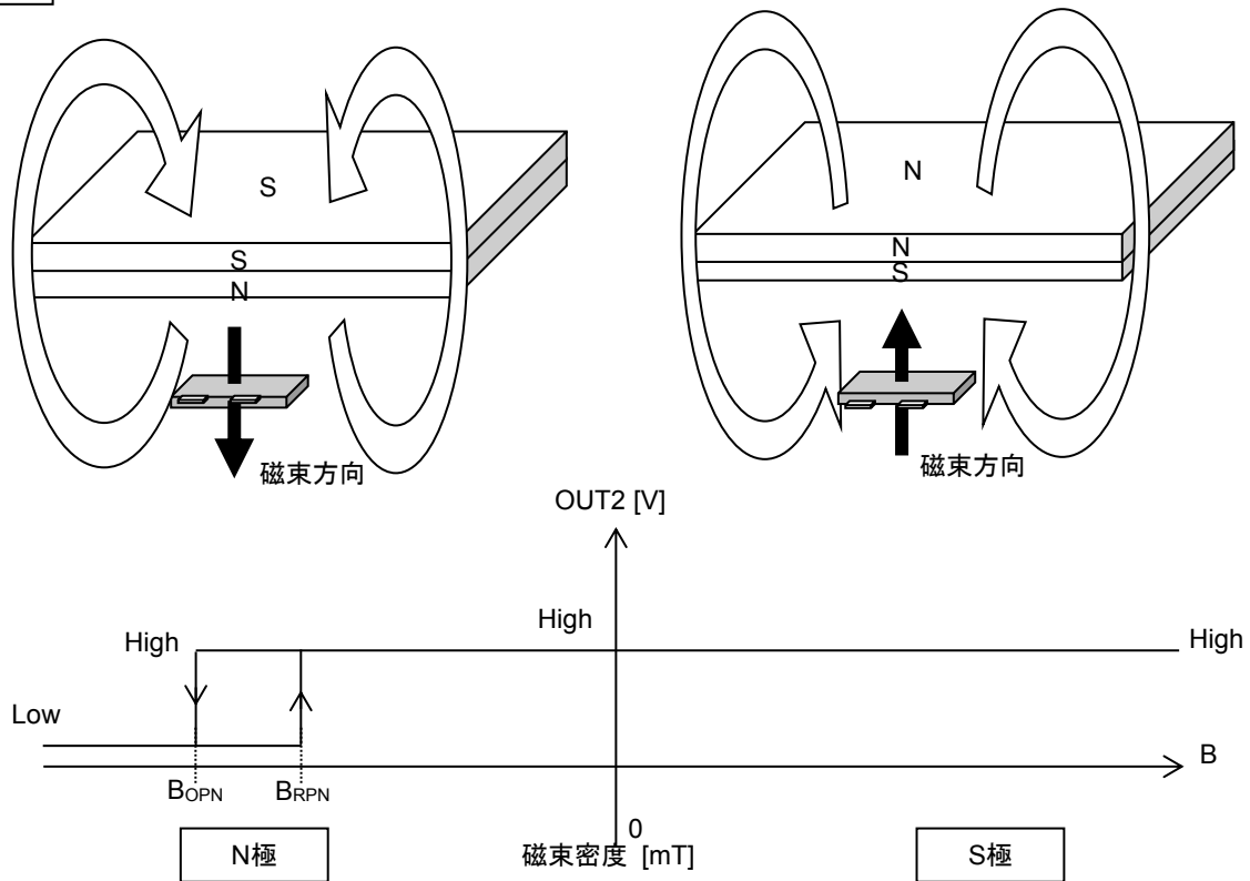
Figure 15. N 極検出動作
