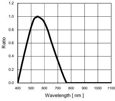
Fig.1 分光感度特性
