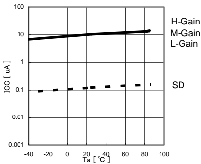
Fig.7 Ta - ICC (0 lx 時)
