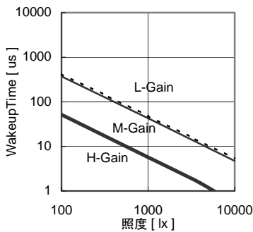
Fig.10 照度 - Wake up Time
