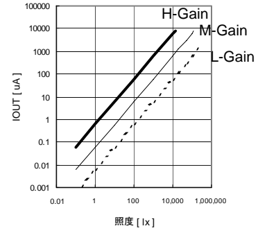
Fig.3 照度 - IOUT 特性
