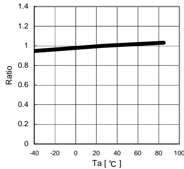
Fig.8 IOUT 出力温度特性 (100 lx 時)
