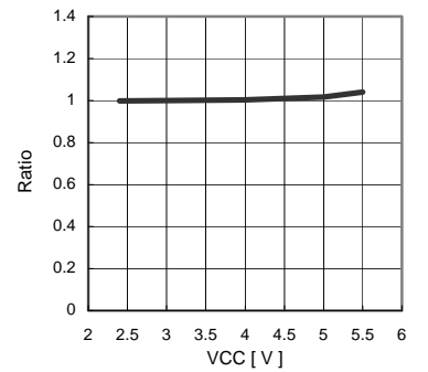
Fig.9 IOUT 出力 VCC 依存特性
