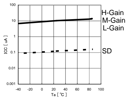
Fig.7 Ta - ICC ( 0 lx 時 )
