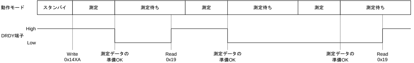
＜DRDY 端子動作の動作例：1 ショット測定モード＞
