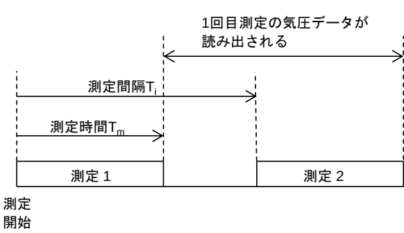
<連続測定モード>
