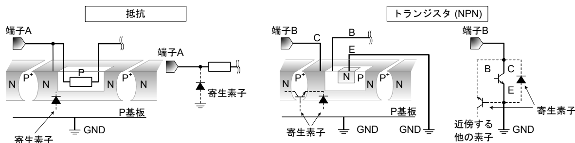
Figure 5. モノリシック IC 構造例
