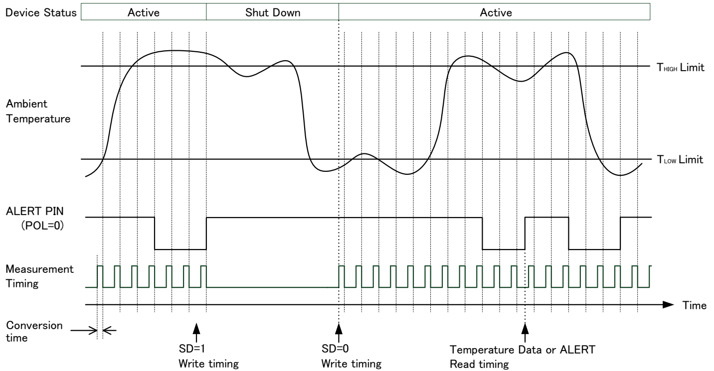
Figure 4. Comparator Mode Action Sequence (フォールト回数=2 回設定時)
