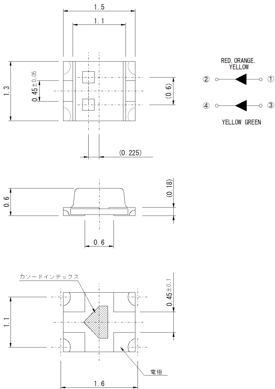
【图-1. 外形寸法图】
