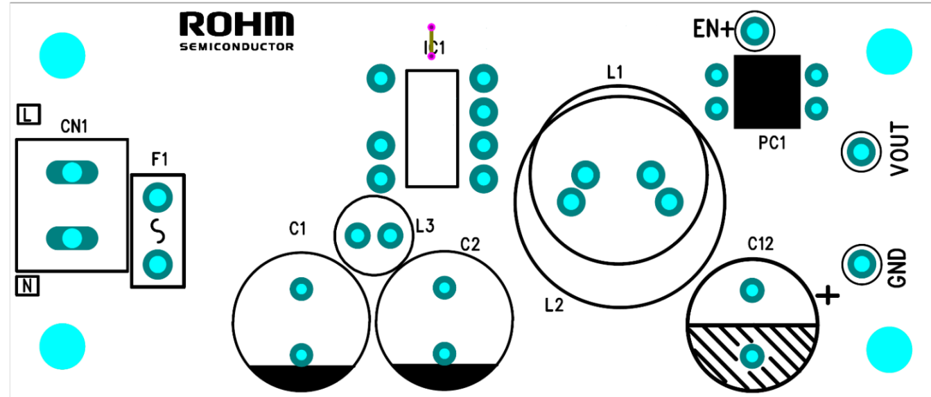
Top Layer
