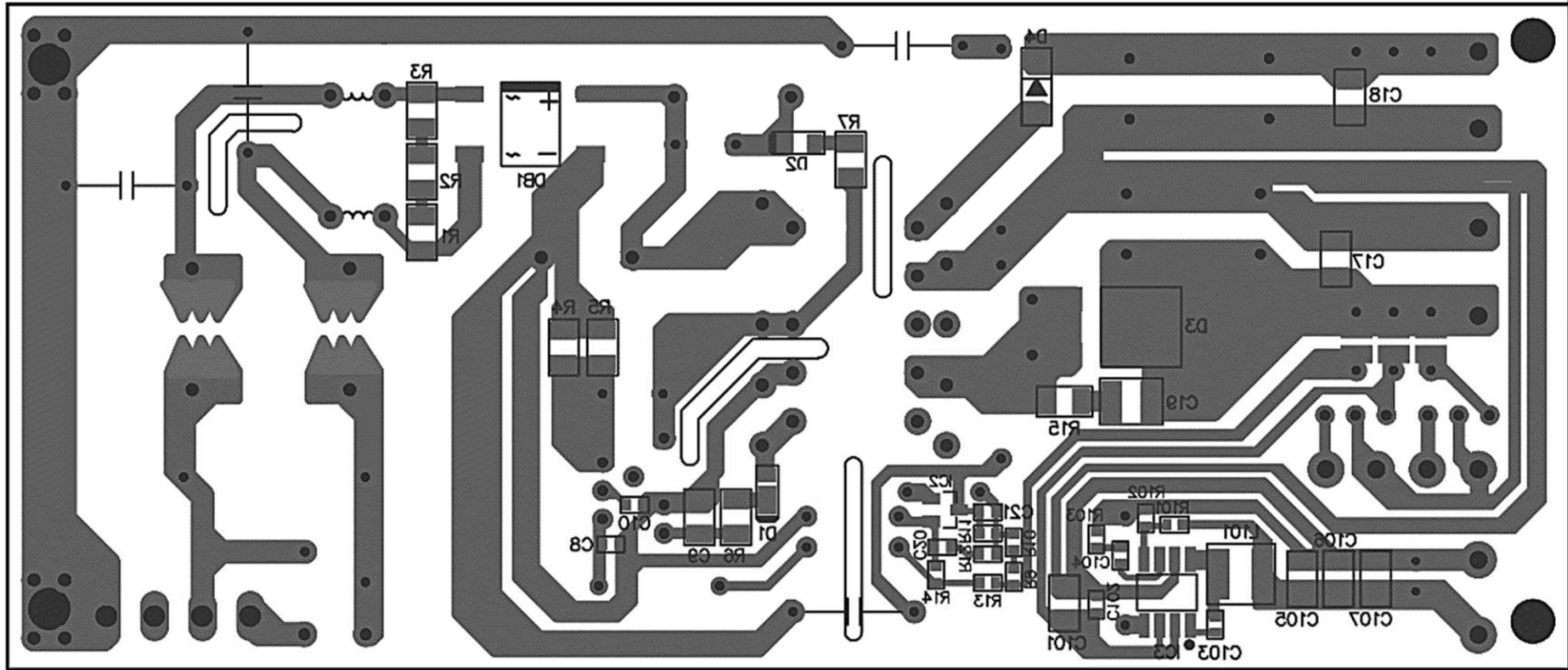
Bottom Layer
