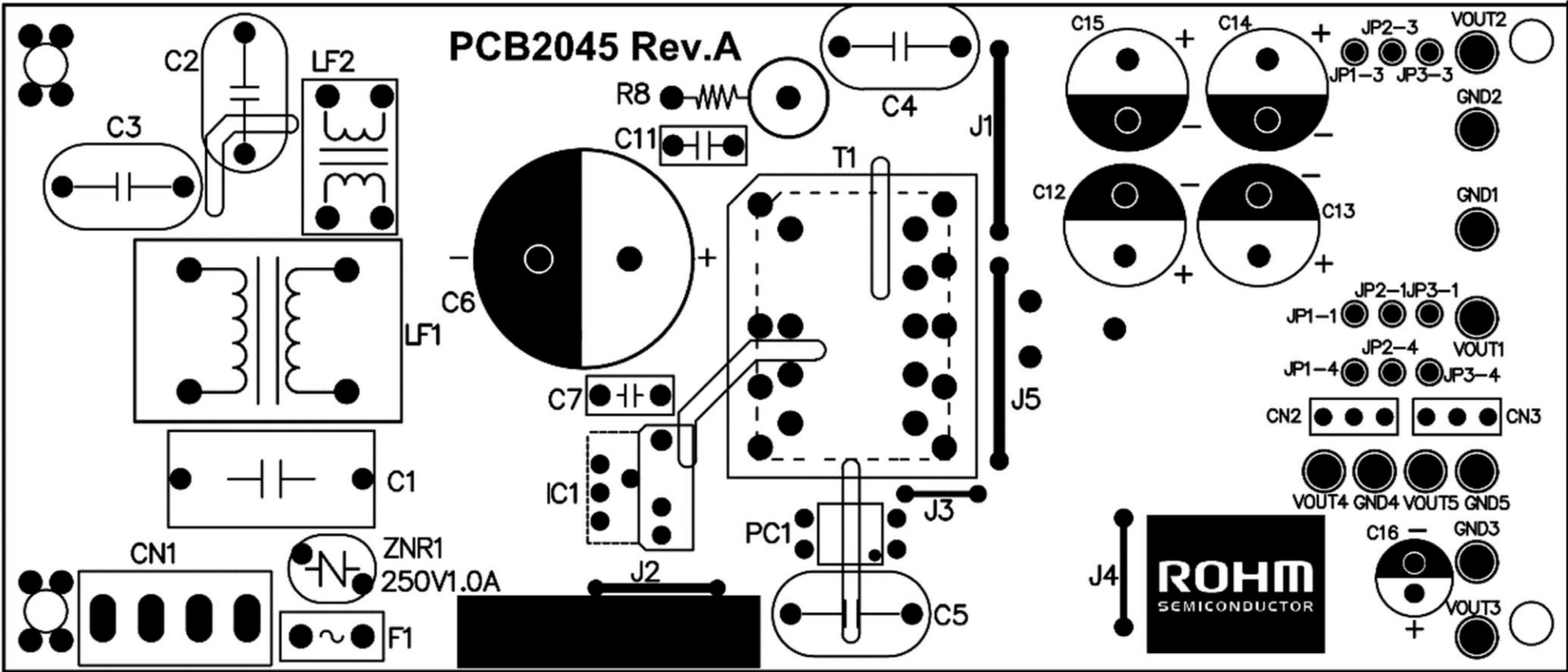
Top Layer
