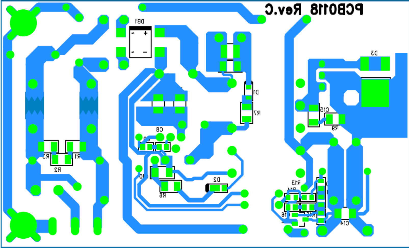
Bottom Layer
