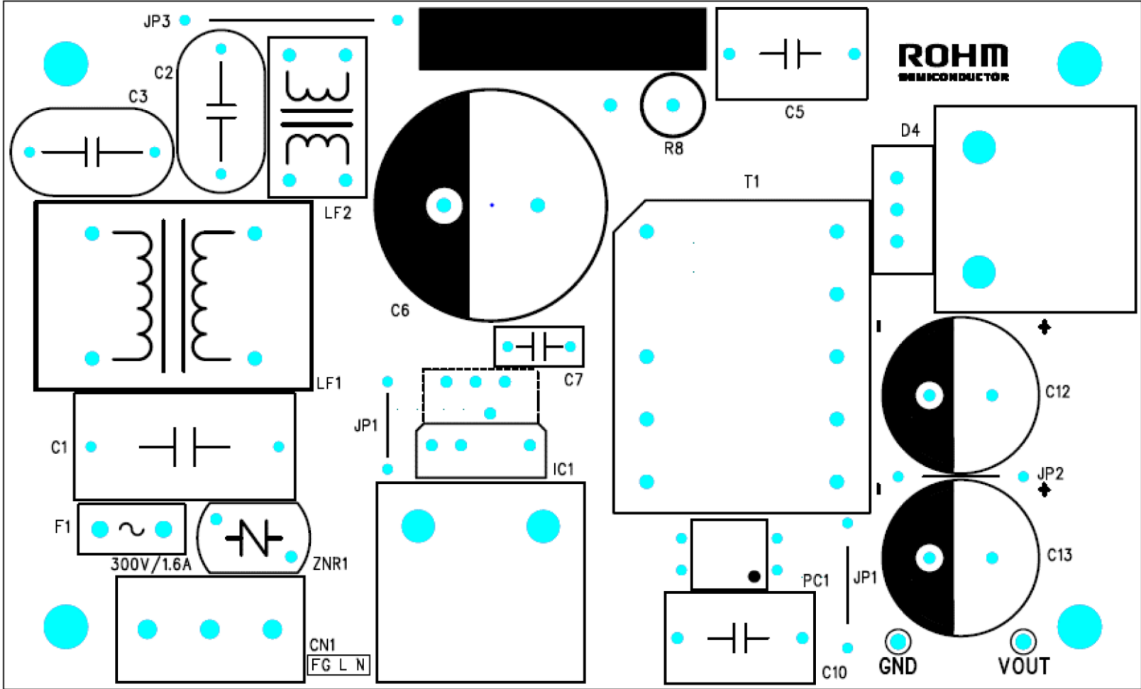
Top Layer
