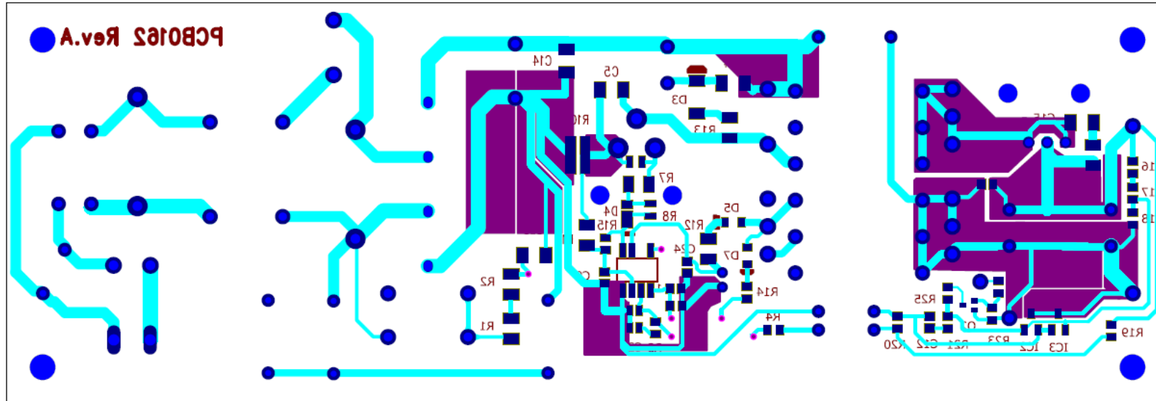
Bottom Layer
