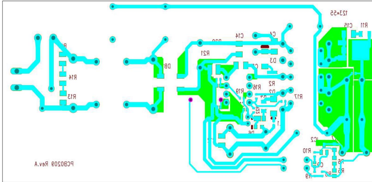
Bottom Layer
