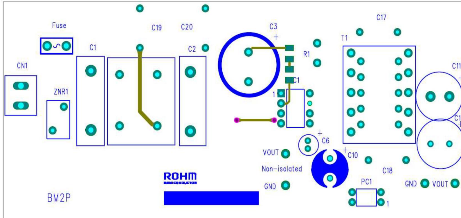
Top Layer
