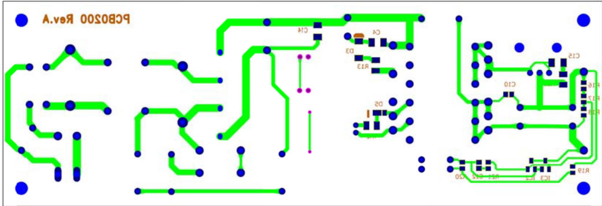
Bottom Layer
