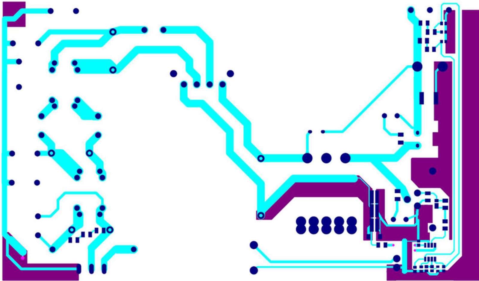
Bottom Layer
