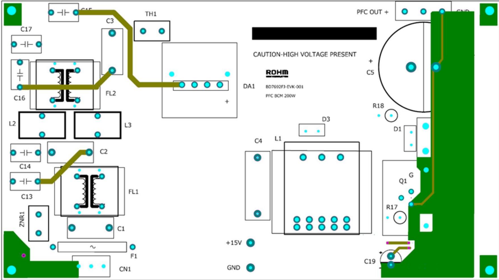
Top Layer
