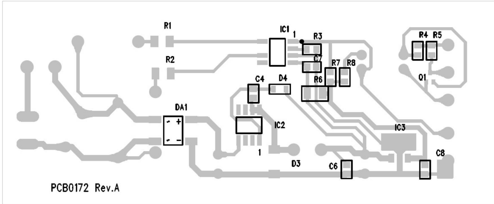
Bottom Layer
